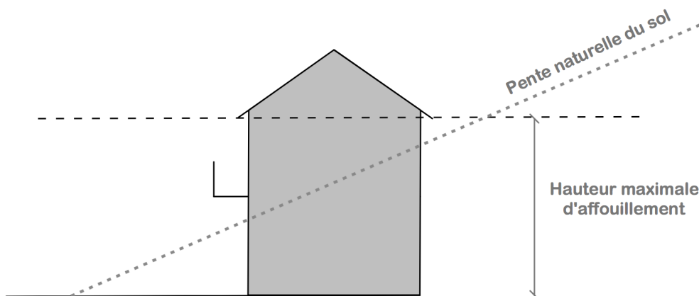
Croquis 2.1
