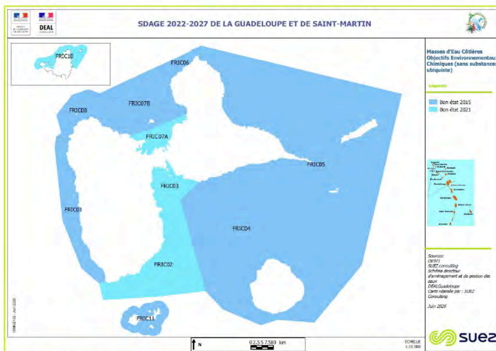
Figure 12 : Carte des objectifs environnementaux chimiques des masses d'eau côtières (sans substances ubiquistes)
