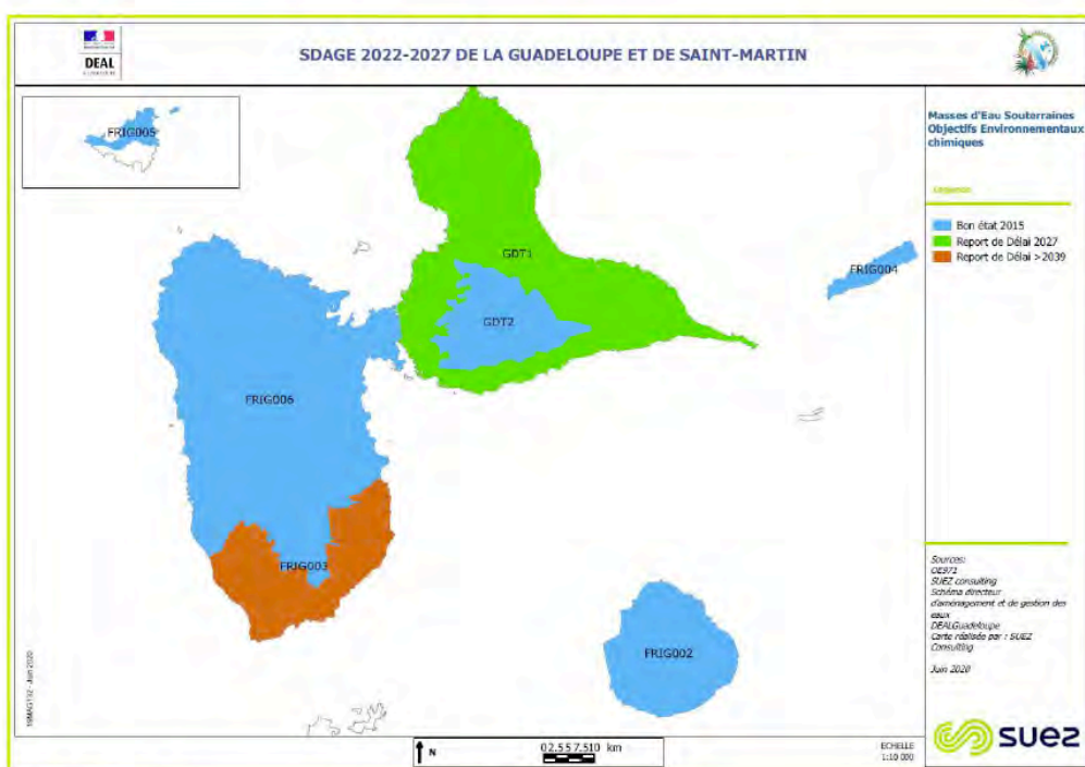
Figure 17 : Carte des objectifs environnementaux chimiques des masses d'eau souterraines
