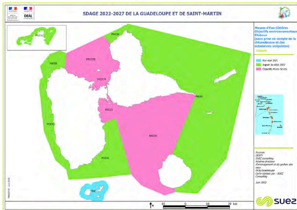
Figure 16 : Carte des objectifs environnementaux globaux des masses d'eau côtières (sans chlordécone ni ubiquistes)
