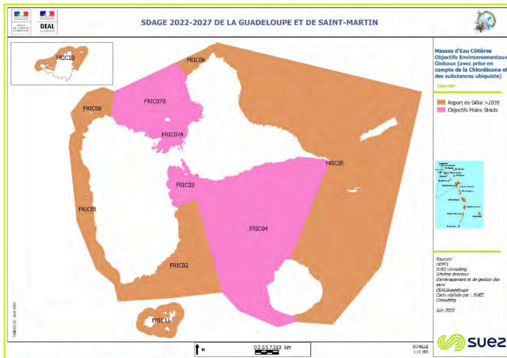
Figure 15 : Carte des objectifs environnementaux globaux des masses d'eau côtières (avec chlordécone et ubiquistes)
