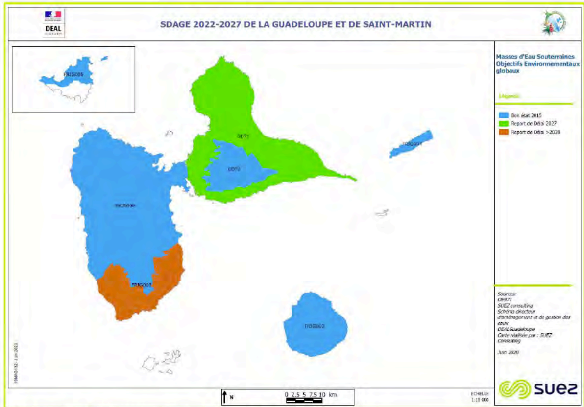
Figure 20 : Carte des objectifs environnementaux globaux des masses d'eau souterraines
