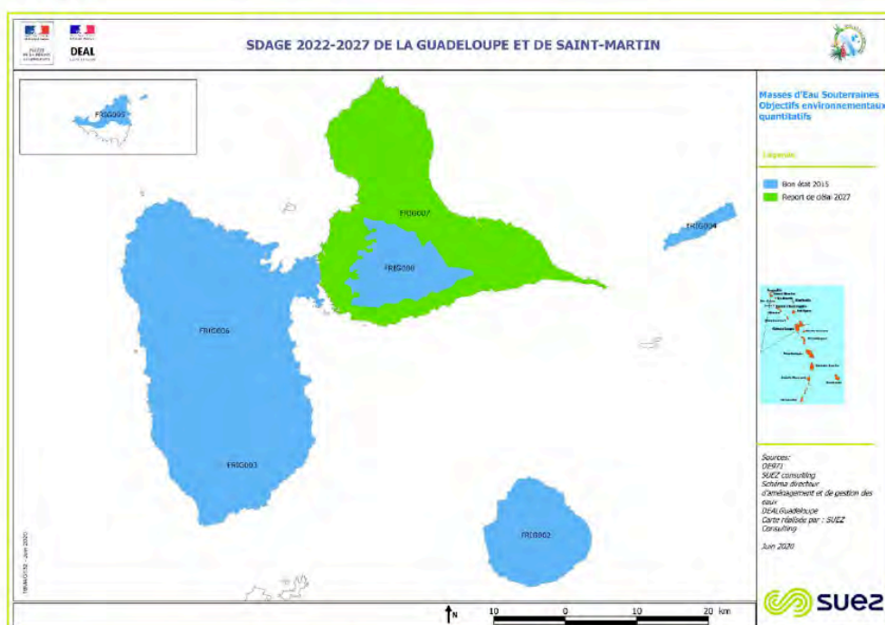
Figure 18 : Carte des objectifs environnementaux quantitatifs des masses d'eau souterraines
