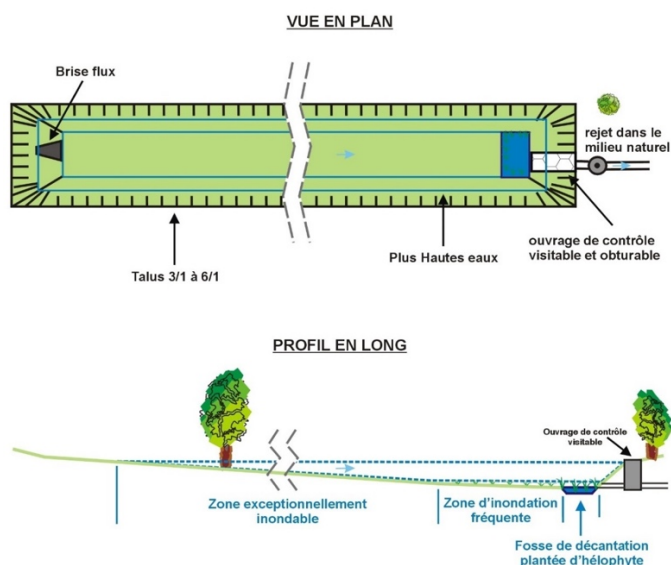
Schéma d'un bassin de rétention à sec enherbé
