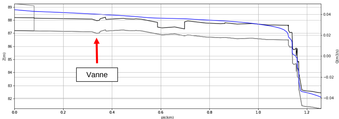
Figure 4.5 : Scénario A, profil de l'Aubette et dalot en charge
