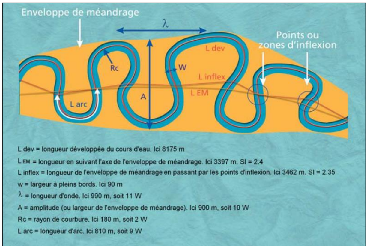
Figure 5.26 : Caractéristiques des méandres
