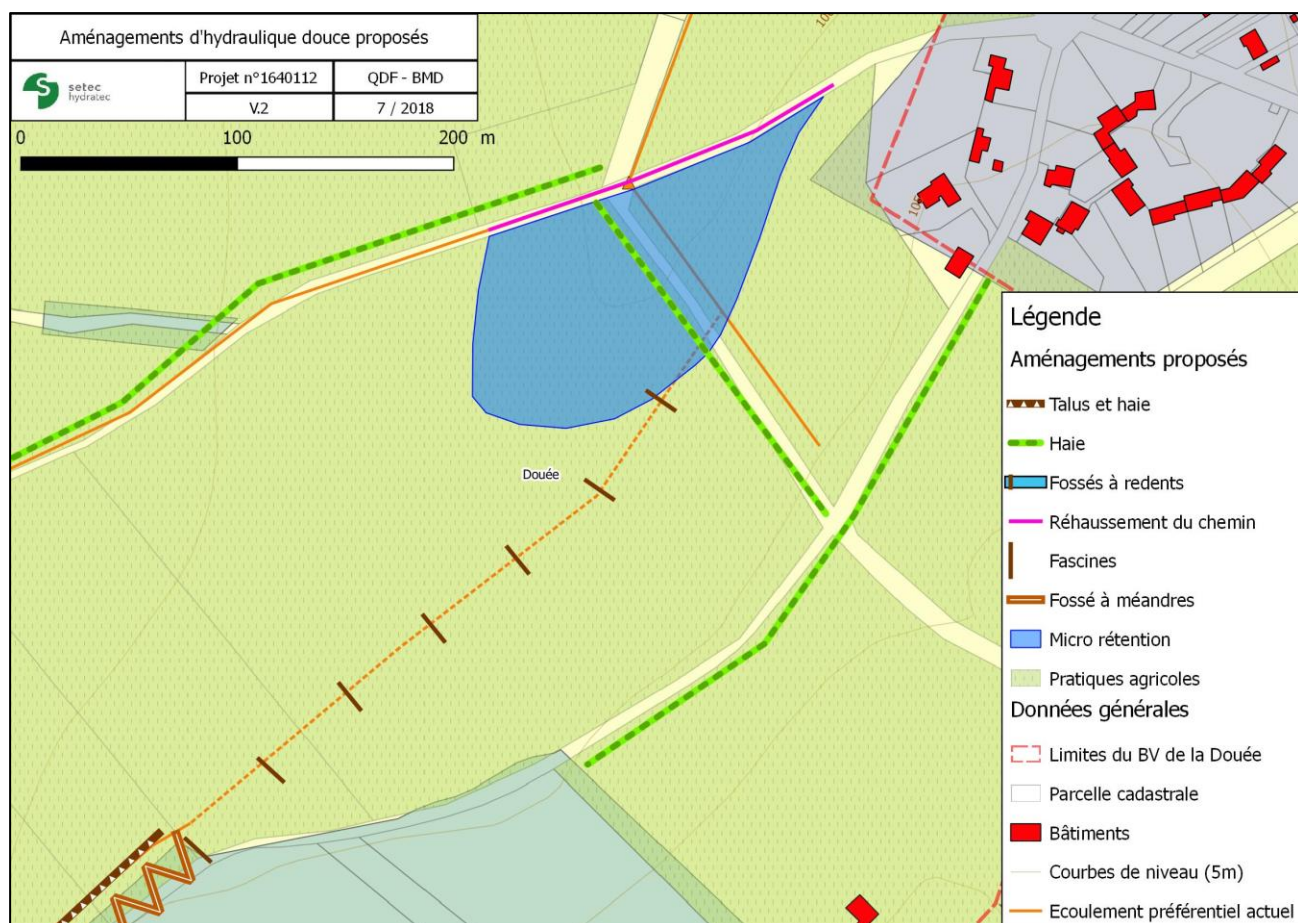
Figure 5.27 : Aménagements de l'aval du bassin versant de la Douée
