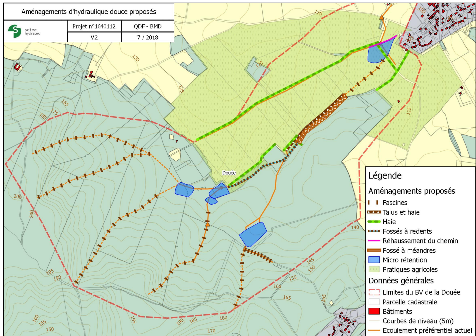
Figure 5.21 : Ensemble des aménagements d'hydraulique douce proposés
