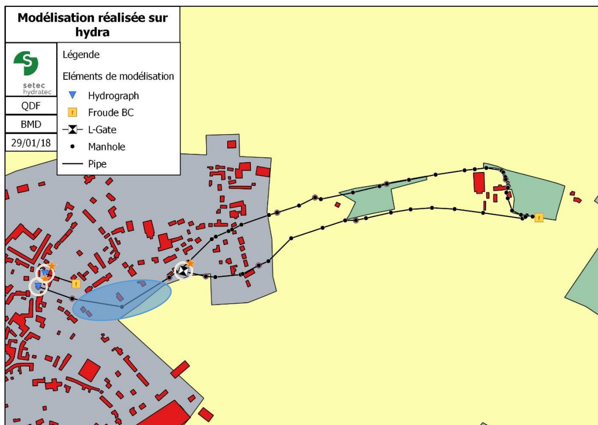
Figure 4.8 : Zone sujette à inondation lors de la simulation
