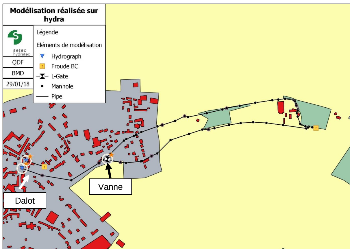
Figure 4.4 : Modèle réalisé sur hydra
