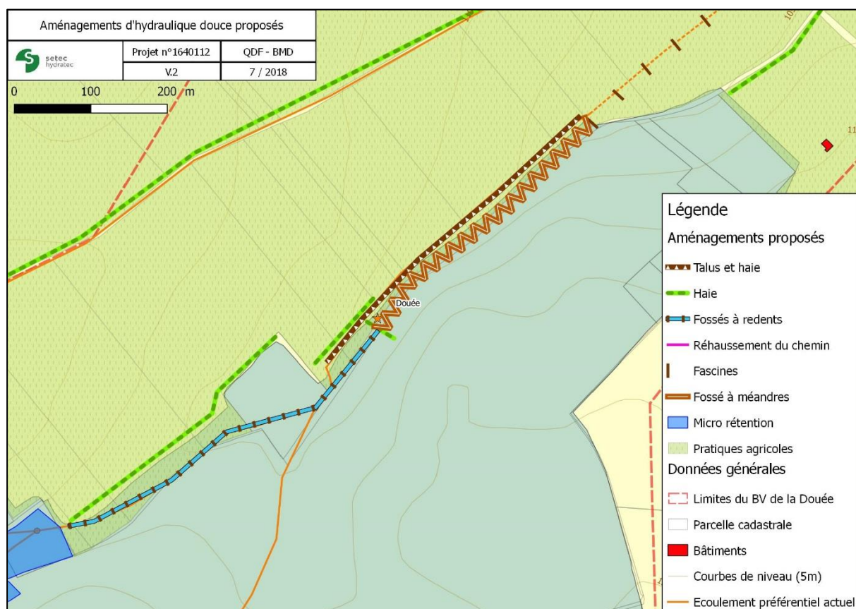
Figure 5.24 : Aménagement le long du bois des Moque-Panier
