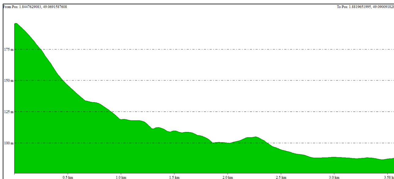
Figure 2.2 : Profil du bassin versant de la Douée
