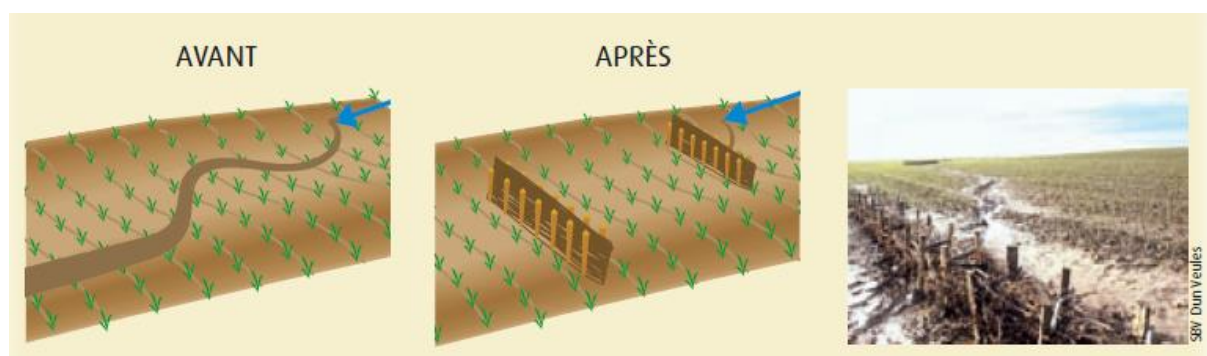
Figure 5.16 : Schéma de fonctionnement de la fascine sur une parcelle agricole
