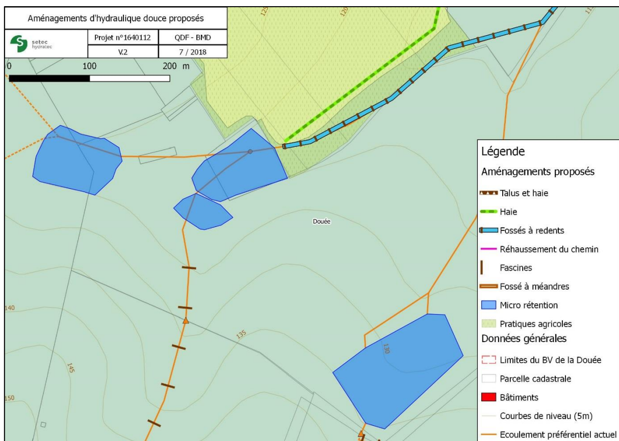
Figure 5.23 : Micro rétentions proposées
