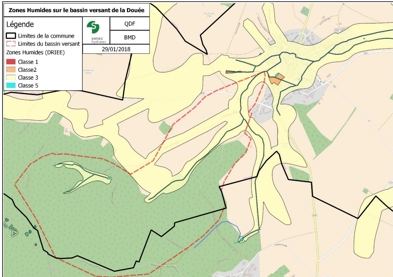
Figure 2.5 : Zones humides du bassin versant de la Douée (DRIEE)
