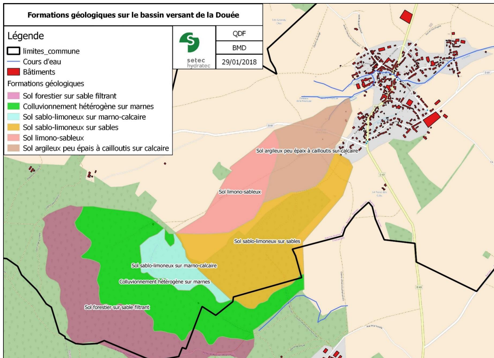
Figure 2.3 : Formation géologiques du bassin versant de la Douée (BRGM)
