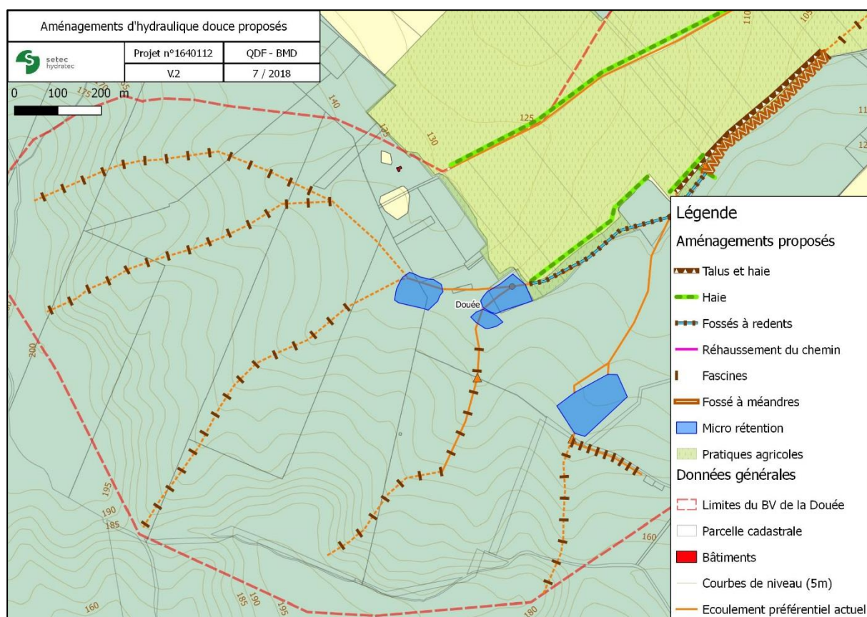
Figure 5.22 : Aménagement à l'amont du bois des Galluis
