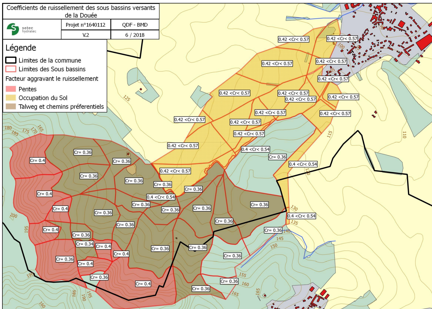
Figure 3.2 : Coefficients de ruissellement des sous bassins versants de la Douée
