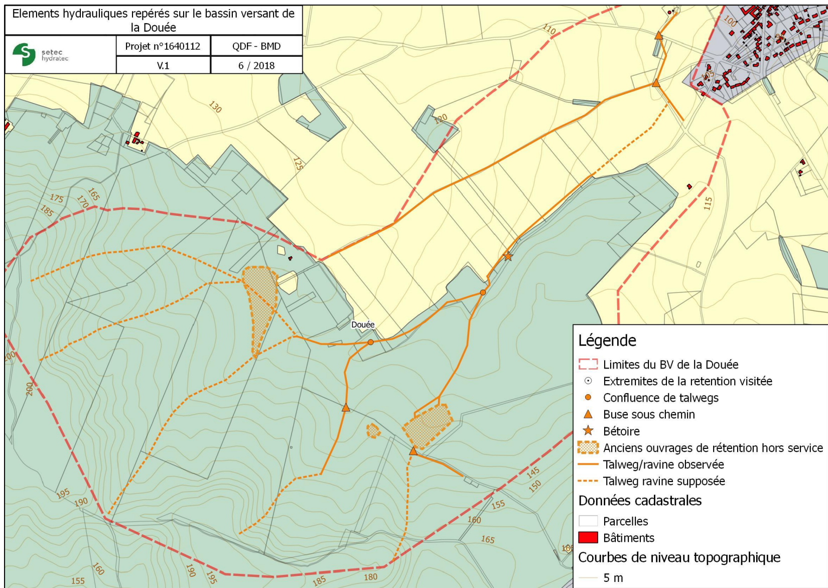
Figure 5.1 : Eléments hydrauliques repérés et supposés sur le bassin versant de la Douée
