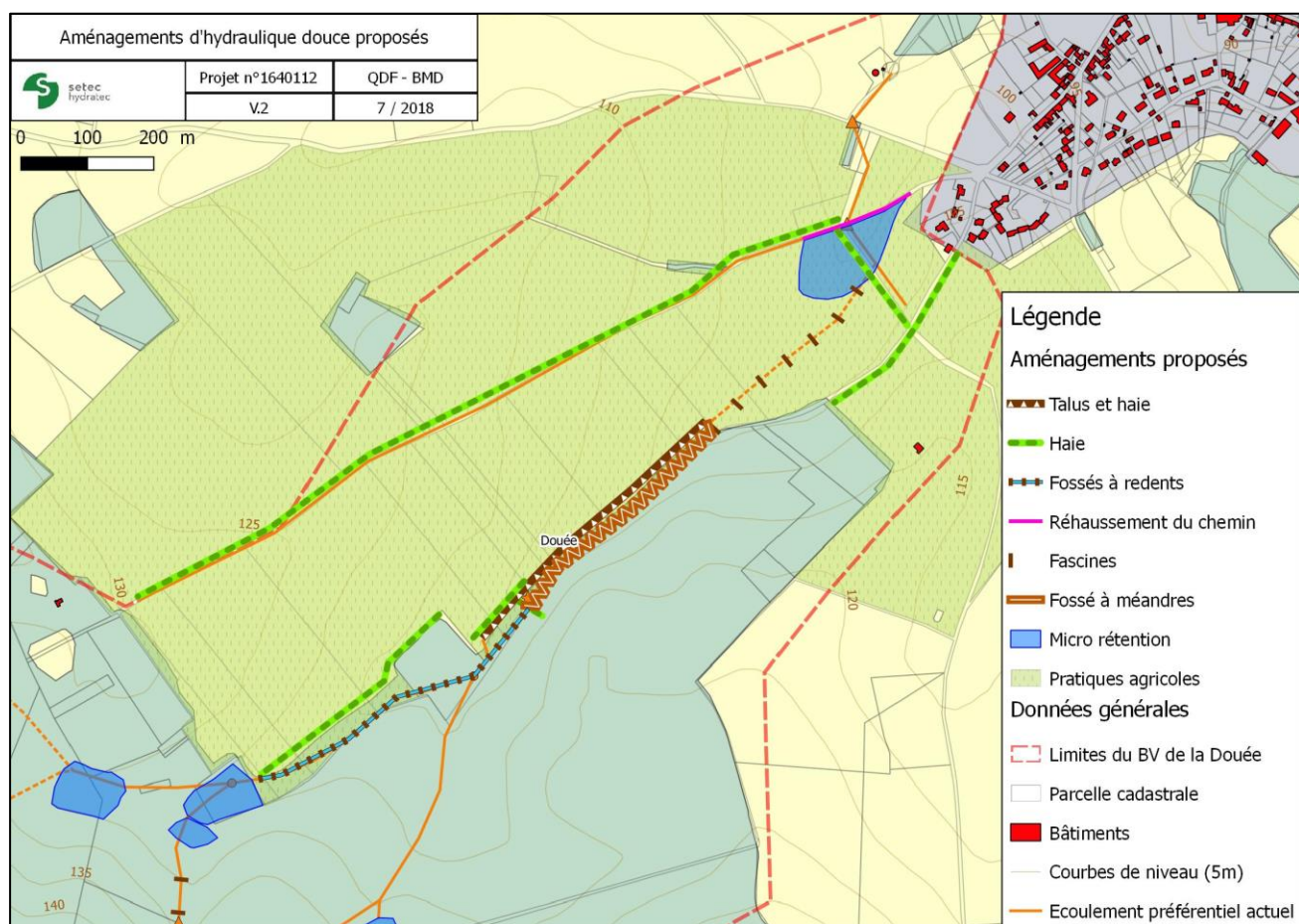
Figure 5.28 : Aménagements proposés au niveau des parcelles agricoles
