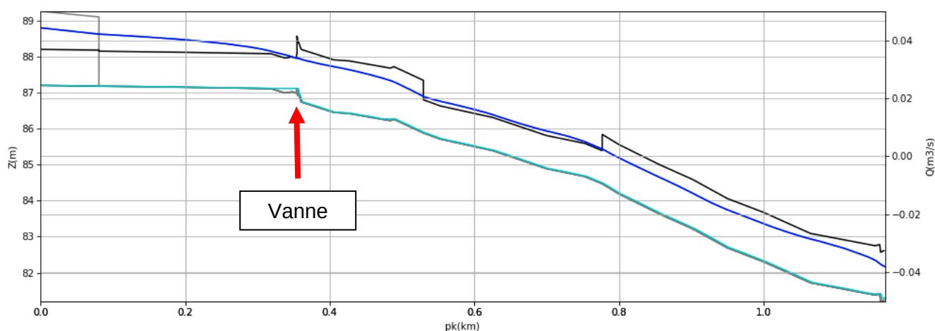
Figure 4.6 : Scénario B, profil du bras de décharge et dalot en charge
