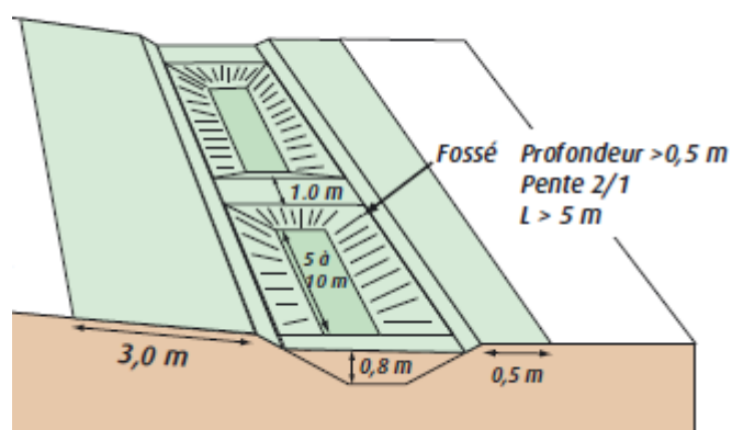
Figure 5.25 : Schéma de conception classique du fossé à redents
