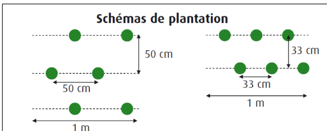
Figure 5.14 : Schémas de plantation d'une haie
