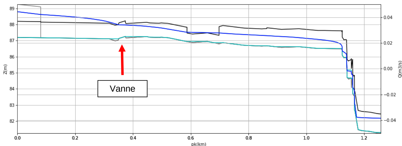
Figure 4.7 : Scénario B, profil de l'Aubette et dalot en charge
