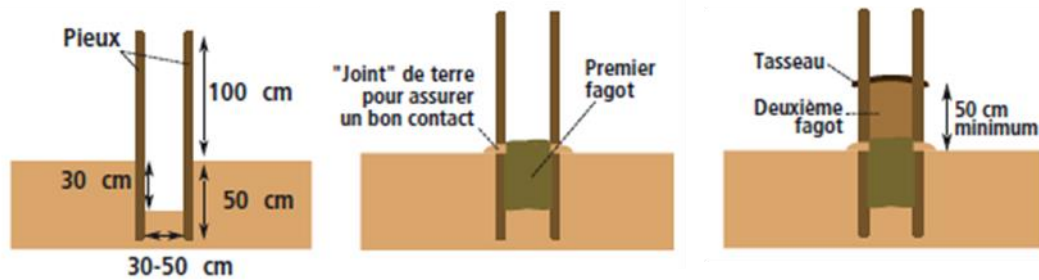
Figure 5.17 : Schémas de principe de la mise en place d'une fascine
