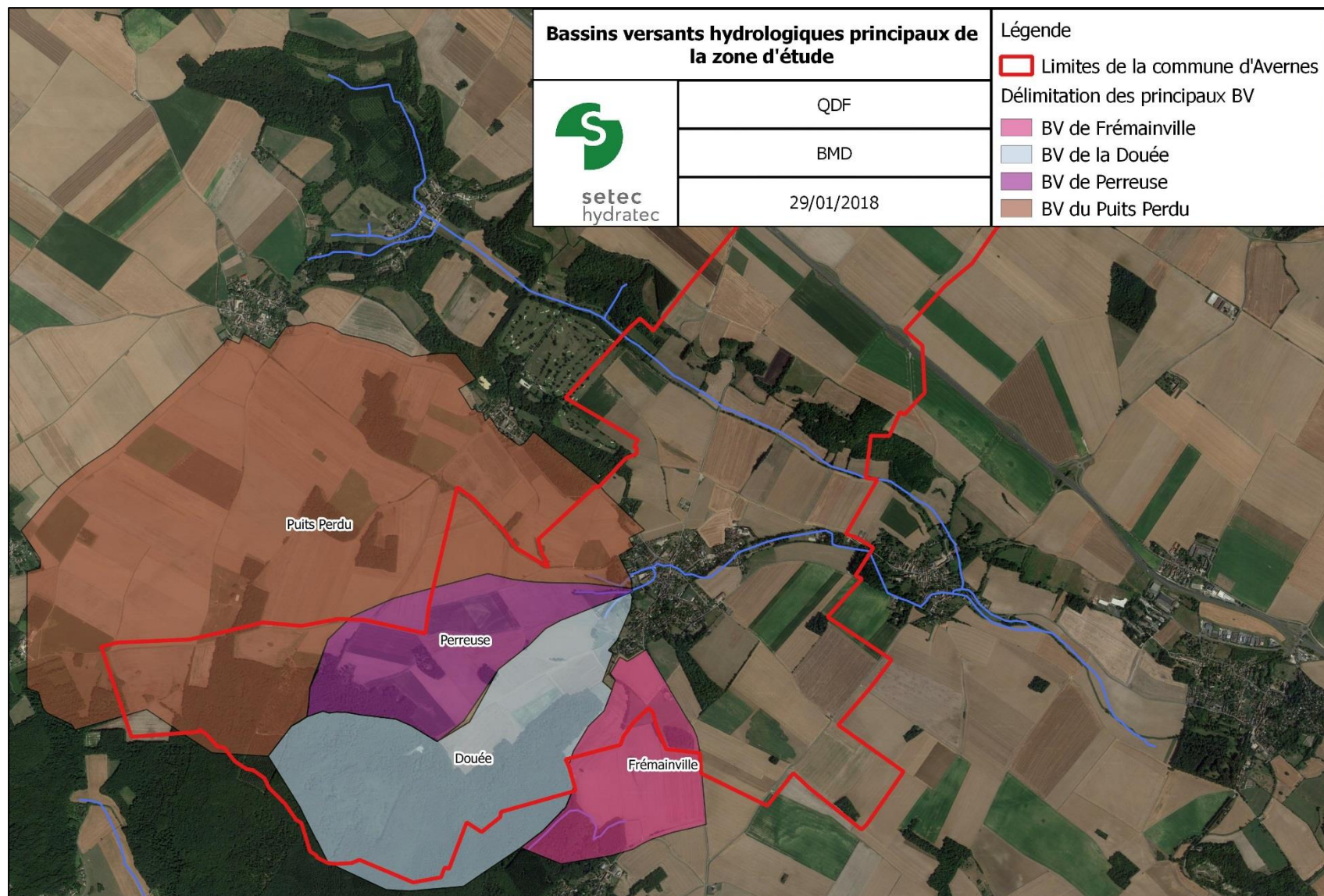
Figure 1.1 : Bassins versants hydrologiques principaux de la zone d'étude
