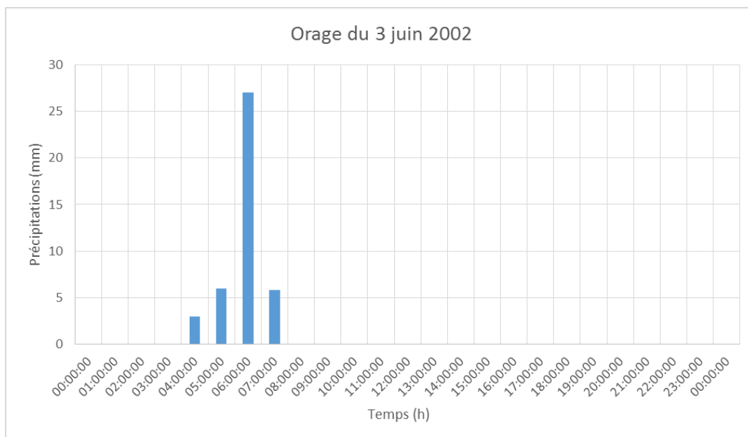
Figure 1.2 : Précipitations à la station Wy-dit-Joli-Village le 3 juin 2002 (source SET ENVIRONNEMENT)
