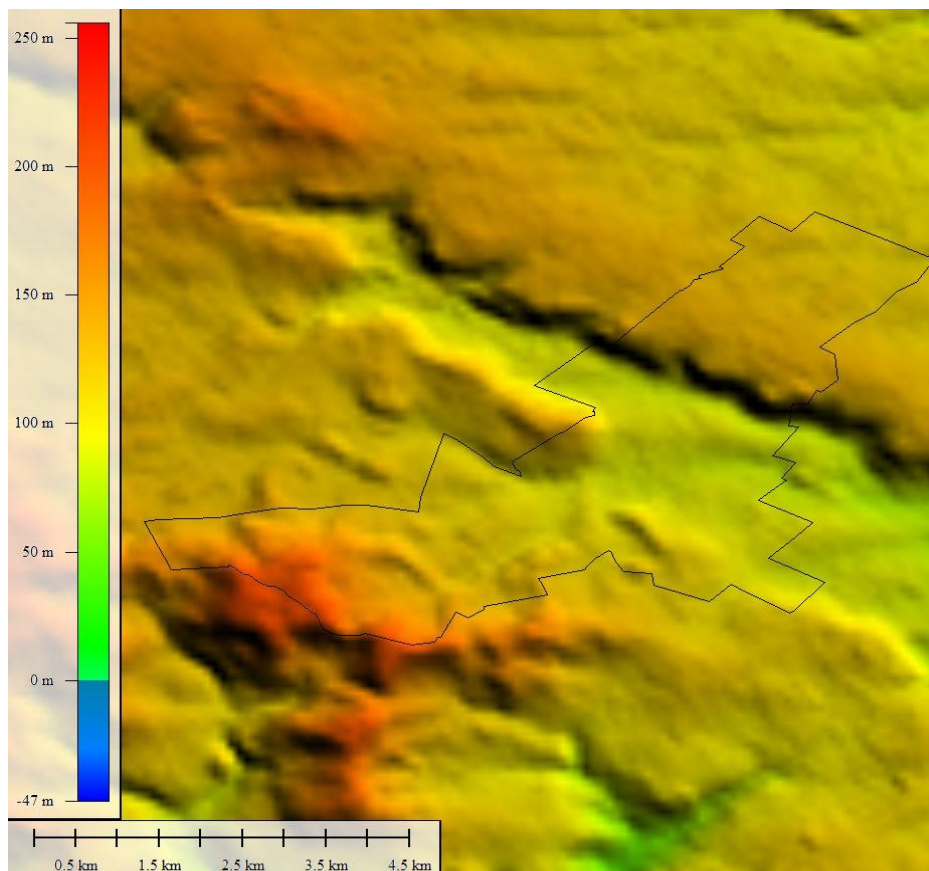
Figure 2.1 : Topographie de la commune d'Avernes (Source : NASA)
