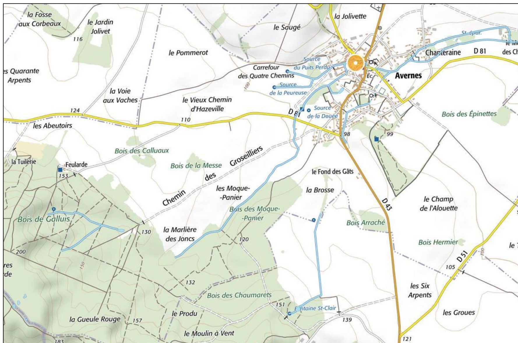
Figure 2.4 : Hydrographie du bassin versant de la Douée (IGN, Géoportail)
