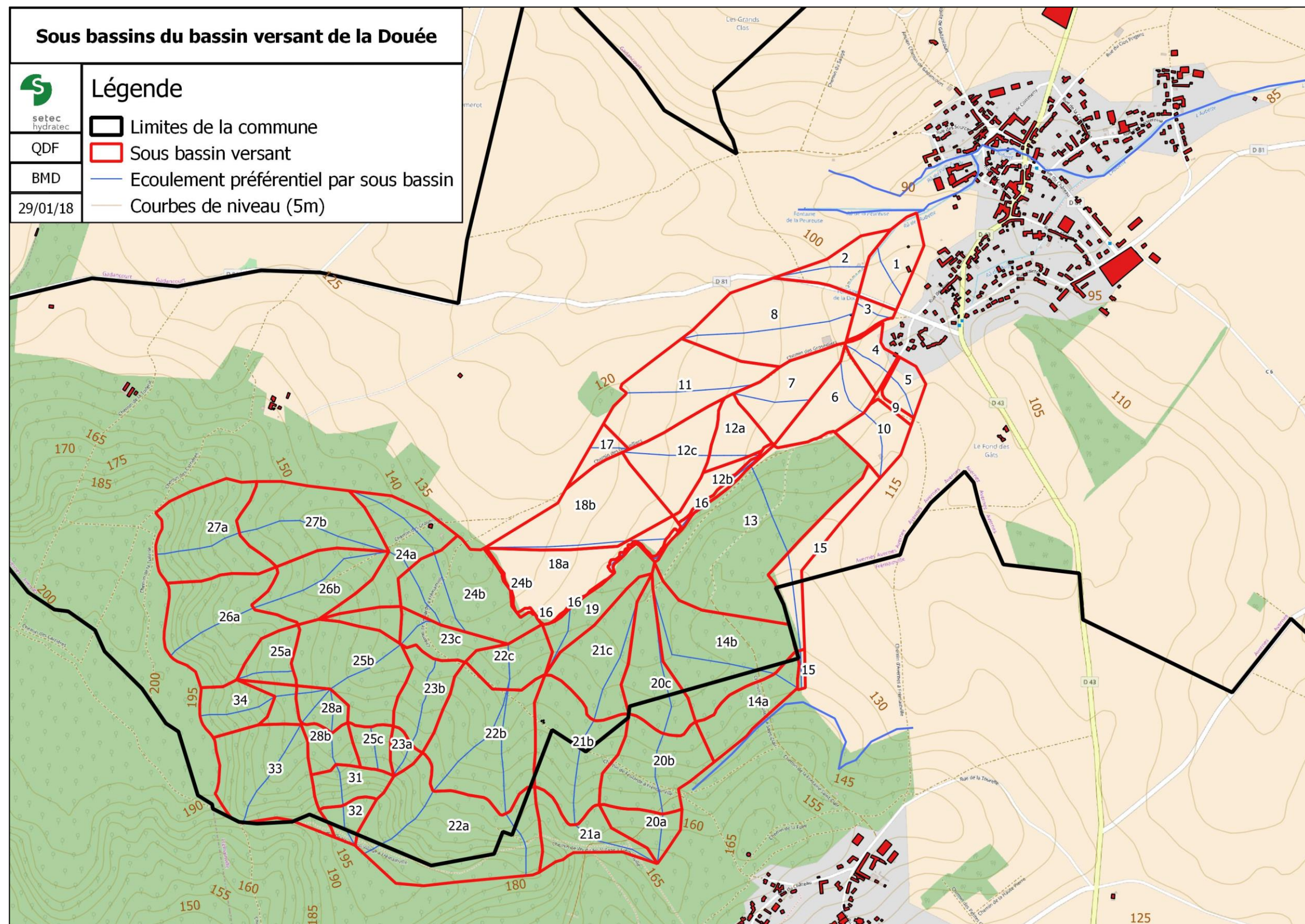
Figure 2.6 : Sous bassins du bassin versant de la Douée
