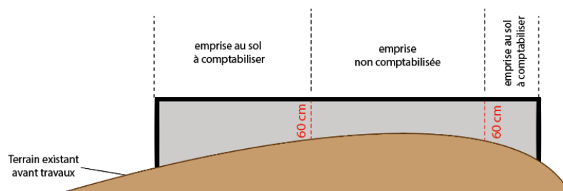
Exemple de l'emprise au sol d'une terrasse
