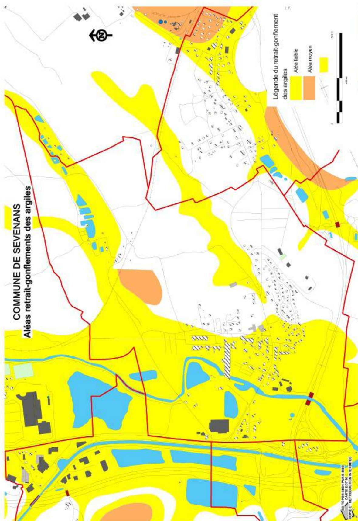
Illustration 5: Carte retrait-gonflement des argiles
