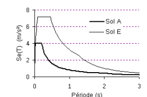
Exemple : spectre horizontal, zone de sismicité 4, catégorie d'importance II
