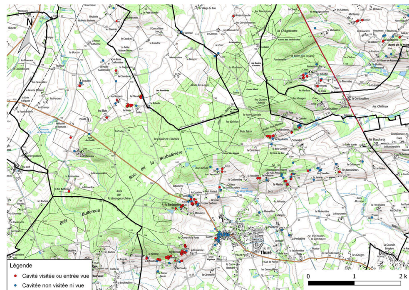
Carte localisant les cavités souterraines recensées par le BRGM sur la commune de Thuré. Source : Caractérisation des enjeux au droit des cavités souterraines dans 13 communes de la Vienne (86), BRGM/RP-66520-FR - Rapport final, 2017 .
