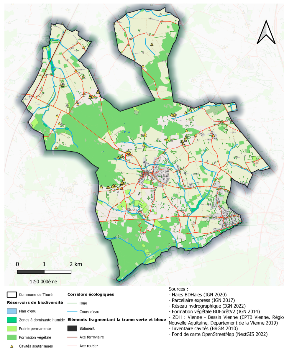
Carte de la trame verte et bleue de Thuré.
