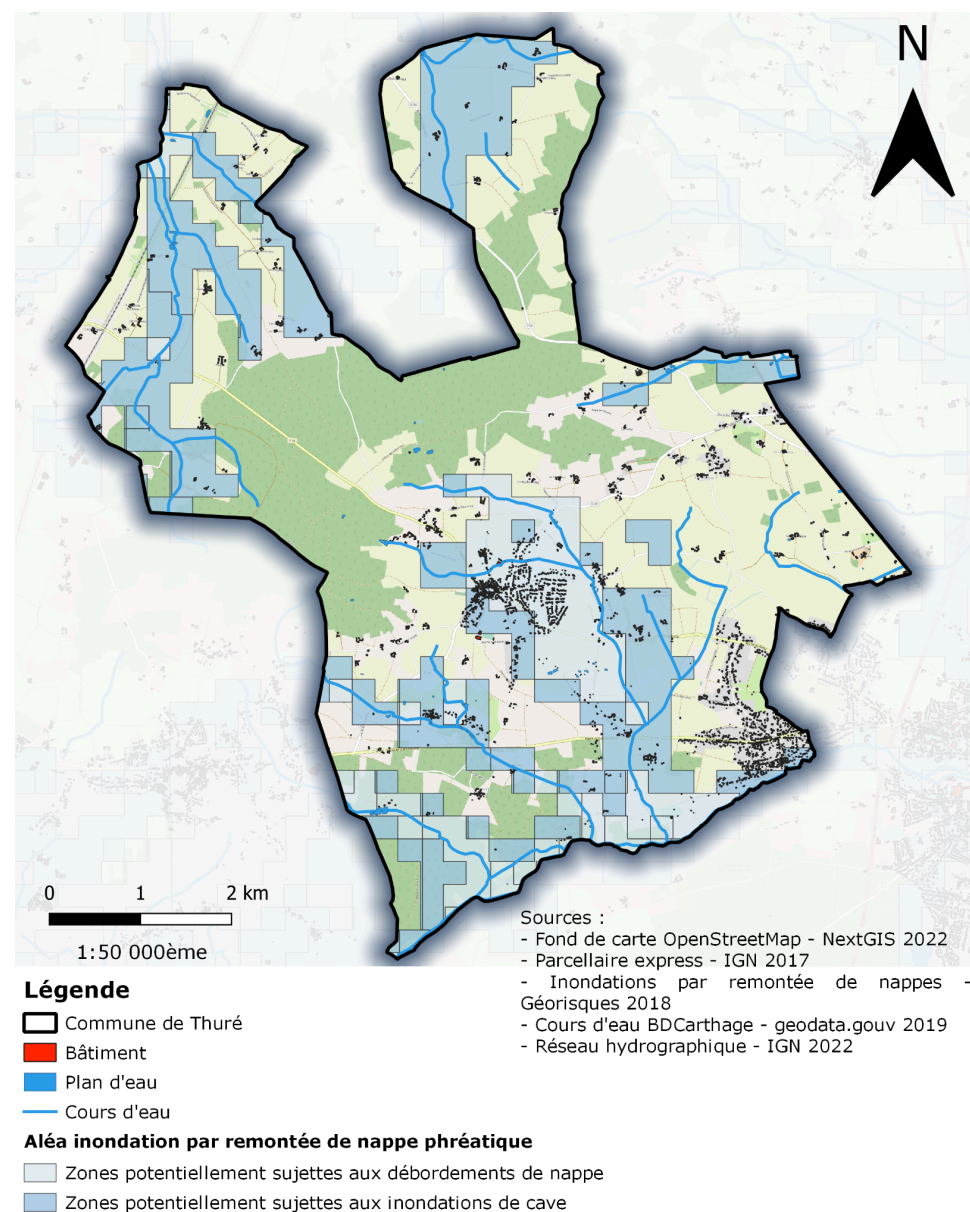
Carte de l'aléa inondation par remontée de nappe à Thuré.
