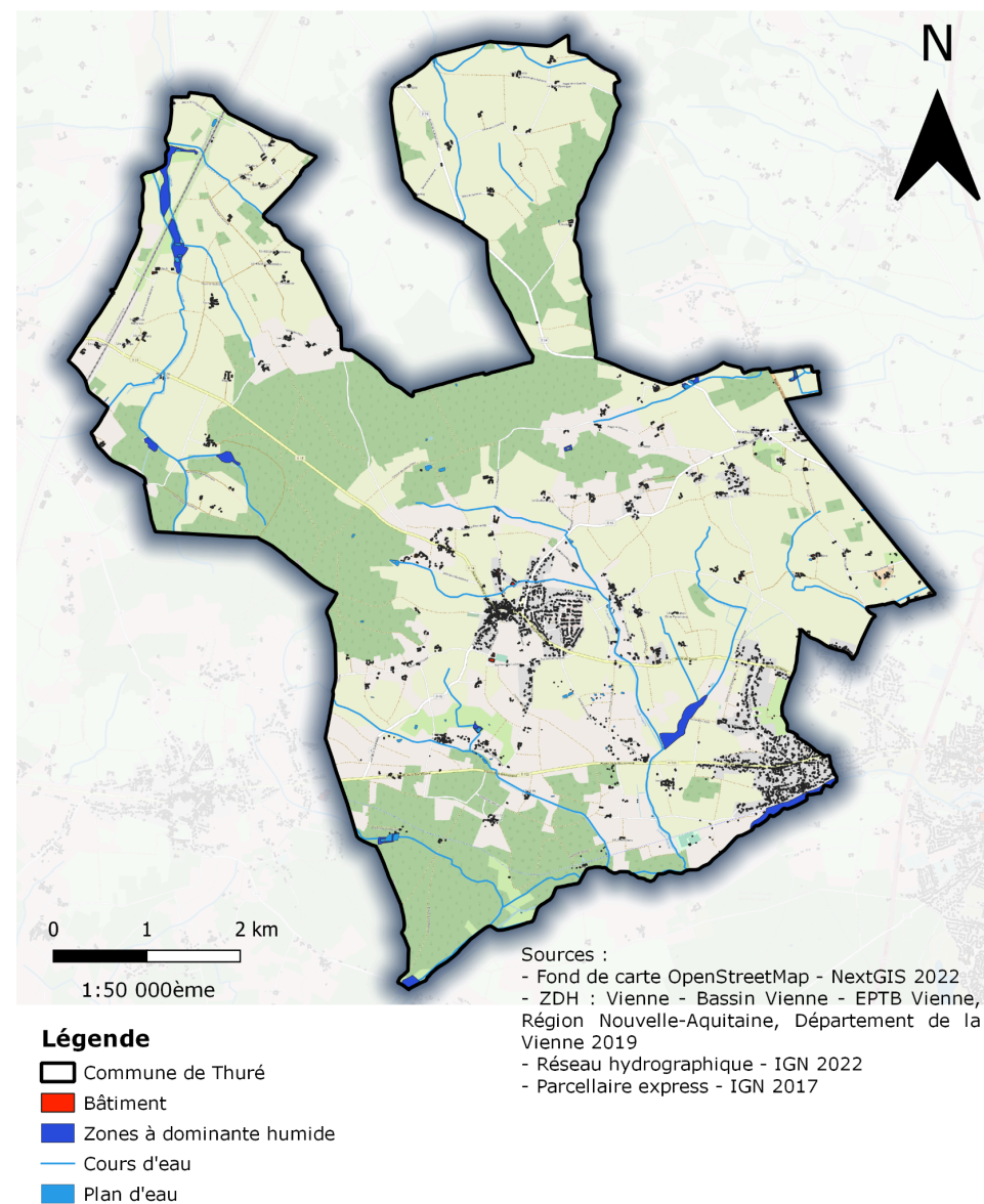
Carte des zones à dominante humide à Thuré.
