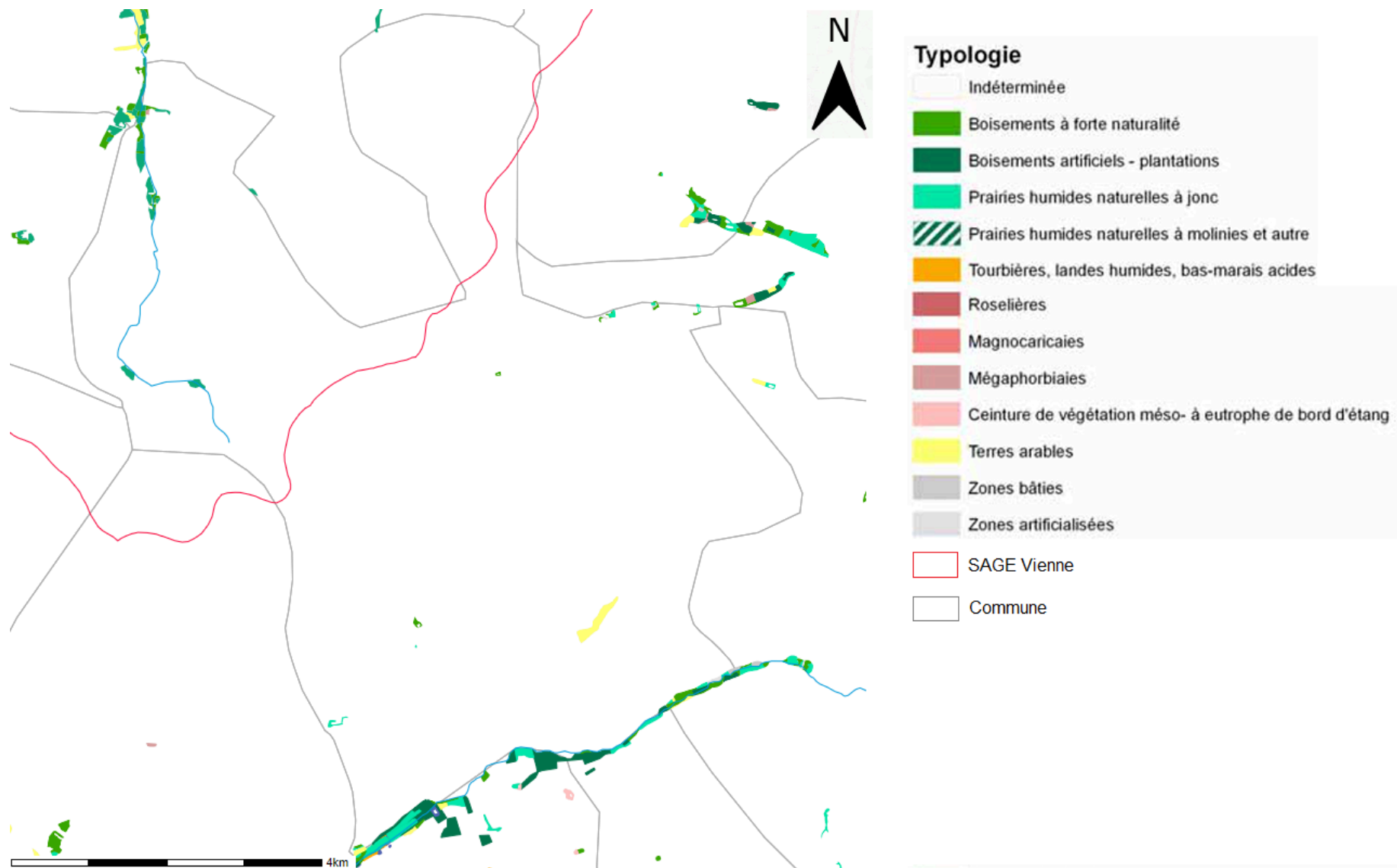
Carte des types de zones à dominante humide sur la commune de Thuré. Source : Prélocalisation des zones humides du bassin de la Vienne, EPTB Vienne 2019.
