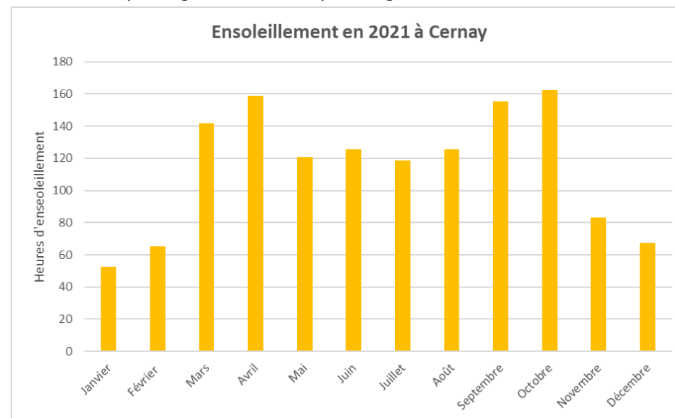
Graphique décrivant l'ensoleillement en heures par mois depuis la station de Cernay. Source : info-climat, 2021.
