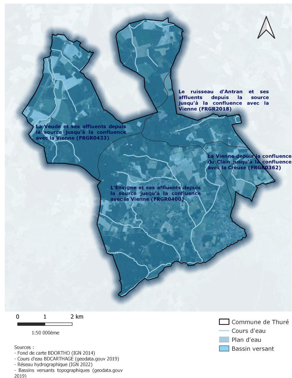
Carte des bassins versants topographique de Thuré
