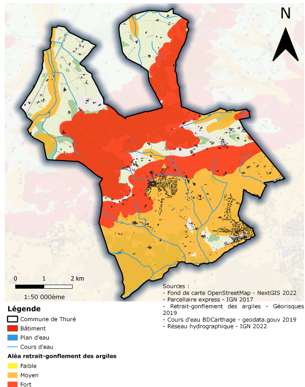
Carte retrait-gonflement des argiles de Thuré.
