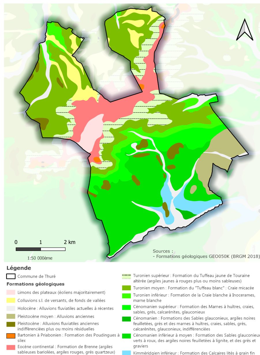
Carte géologique de Thuré
