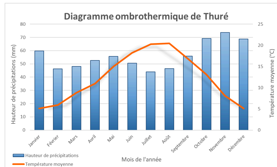
Diagramme ombrothermique de Thuré basé sur les statistiques météorologiques de la station de Thuré de 1981 à 2010. Sources : Infoclimat, Météo-France.
