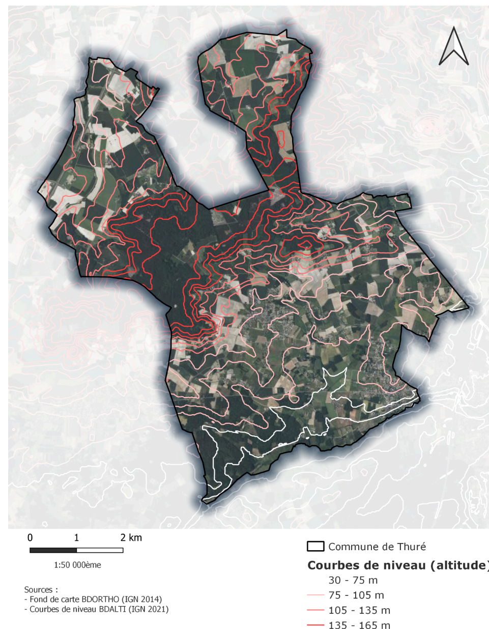
Carte topographique de Thuré
