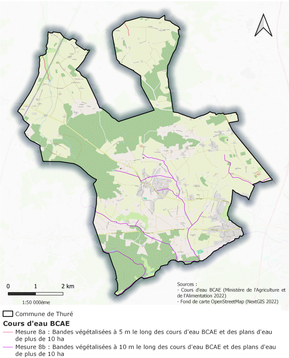
Carte des cours d'eau concernés par les règles des Bonnes Conditions Agricoles et Environnementales (BCAE) sur la commune de Thuré.
