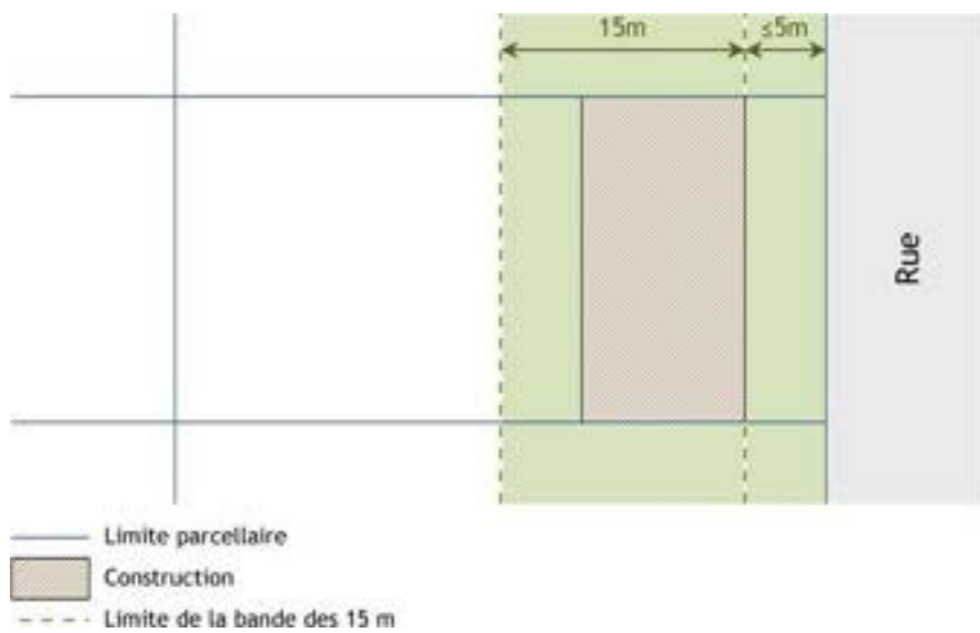
Schéma 5 : bande des 15 m pour l'implantation d'une maison en second rideau
