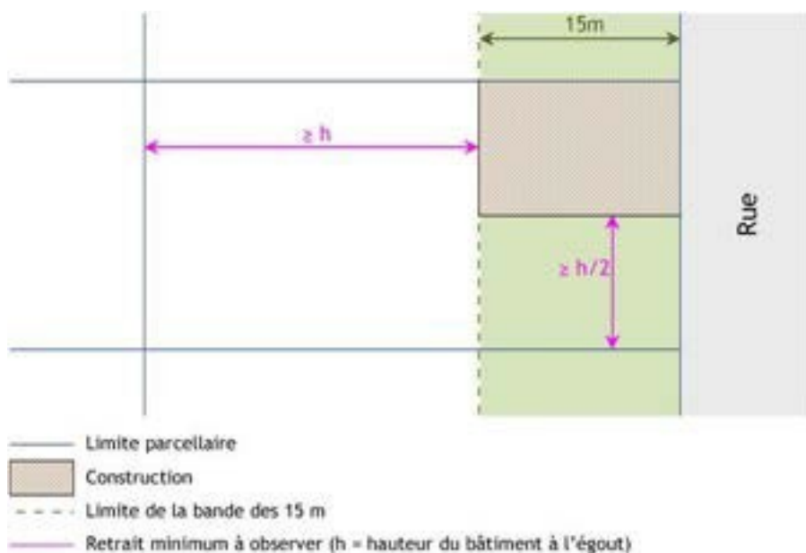
Schéma 7 : implantation par rapport aux limites séparatives (article 7) – cas d'un bâtiment de gabarit inférieur à R+1 ou de hauteur à l'égout inférieure ou égale à 6 m
