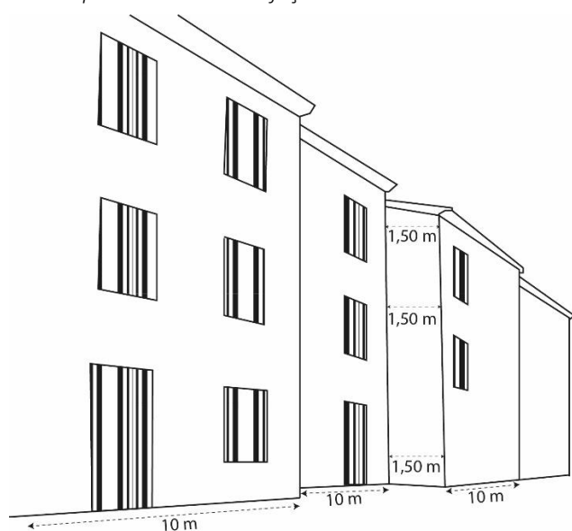
⊕ Croquis du décroché de façade :
