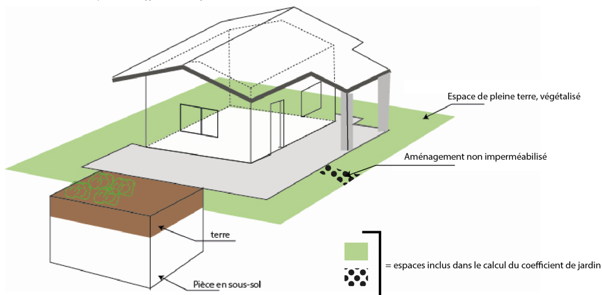
⊕ Schéma concept du coefficient de jardin
