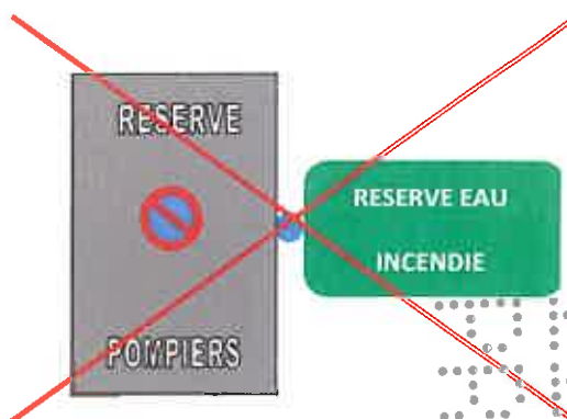
A PROSCRIRE. Emplacement non judicieux. Dans ce cas, l'équipement hydraulique n'est pas utilisable en raison de la rigidité des tuyaux d'aspiration. Il y a lieu soit de déplacer l'équipement hydraulique, soit de déplacer la plate forme d'aspiration.
