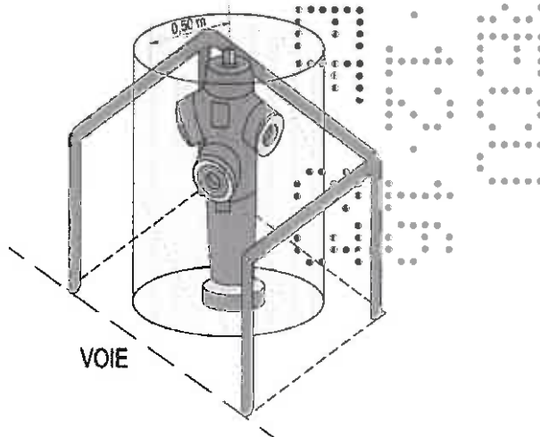
BARRIERE DE PROTECTION D'UN POTEAU D'INCENDIE - Schema de principe -
