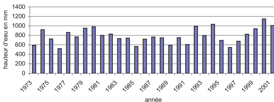
Evolution des précipitations de 1973 à 2001 à la station météorologique d'Abbeville
