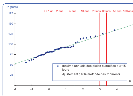
Ajustement de Gumbel sur 15 jours à la station de Cottency
