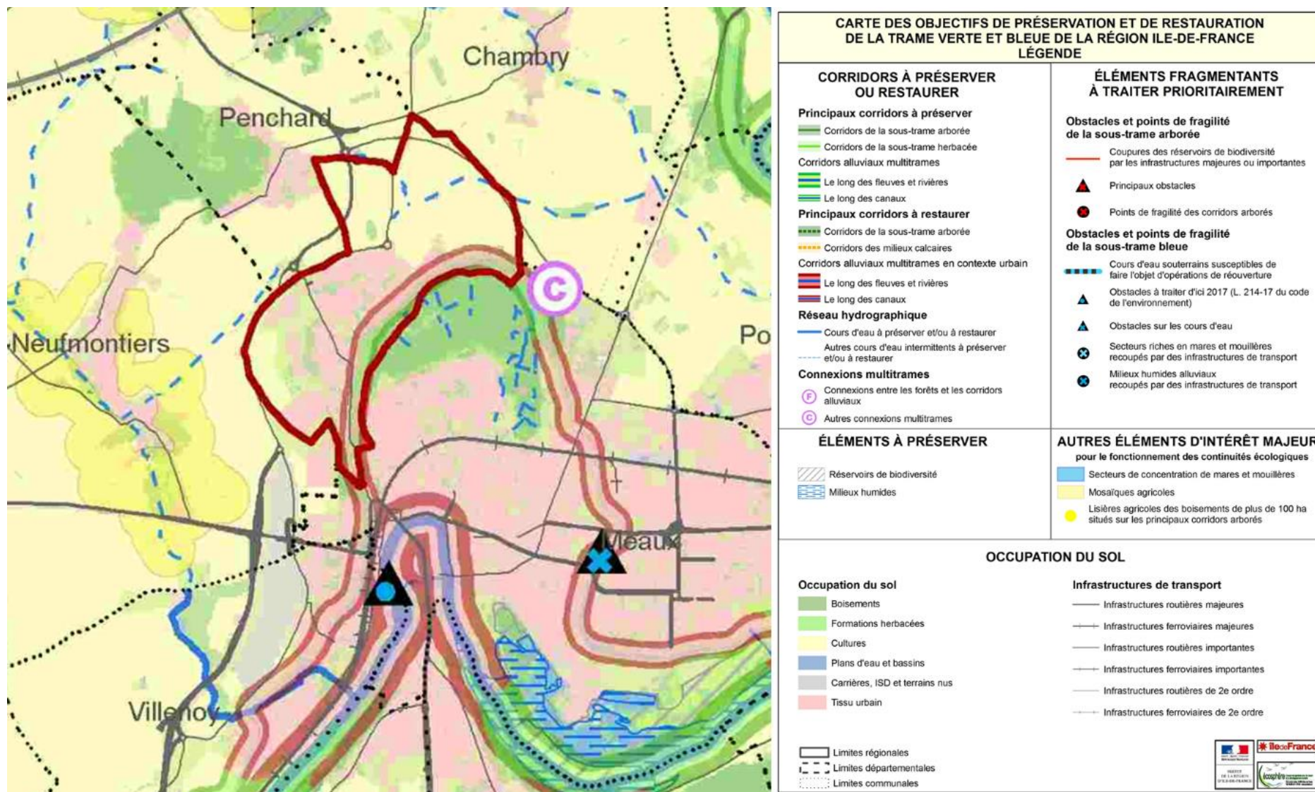
Figure 20 – Objectifs du SRCE (Source : SRCE, Natureparif )
