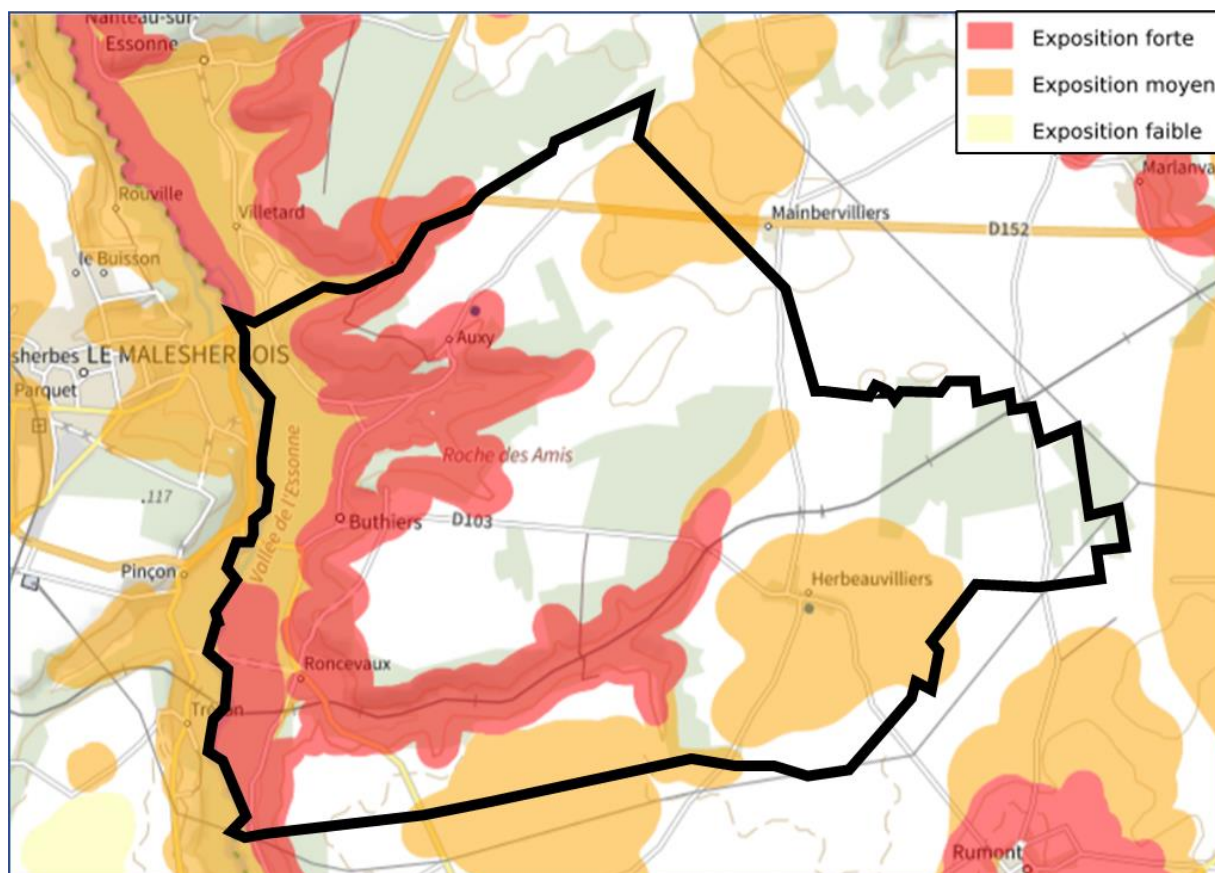
Risque de retrait et gonflement des argiles sur la commune de Buthiers (source : Géorisques)
