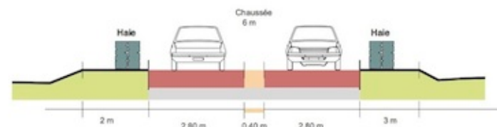
Coupe projet
