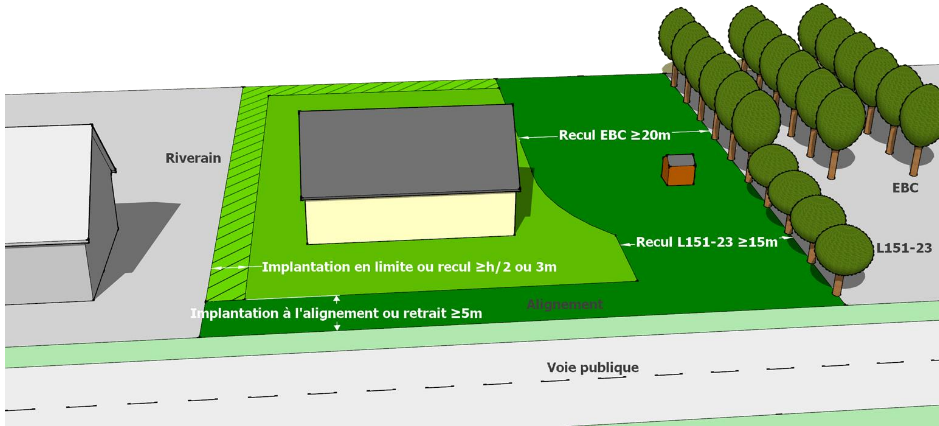
Illustration du cas général d'implantation des constructions (attention, d'autres implantations peuvent être imposées dans les dispositions spécifiques de zones)
