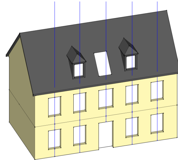
Principe d'implantation des châssis de toit et les lucarnes
