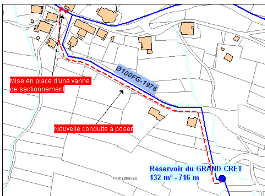
Figure 19 : isolement des secteurs de distribution du Plon et du Grand Crêt
