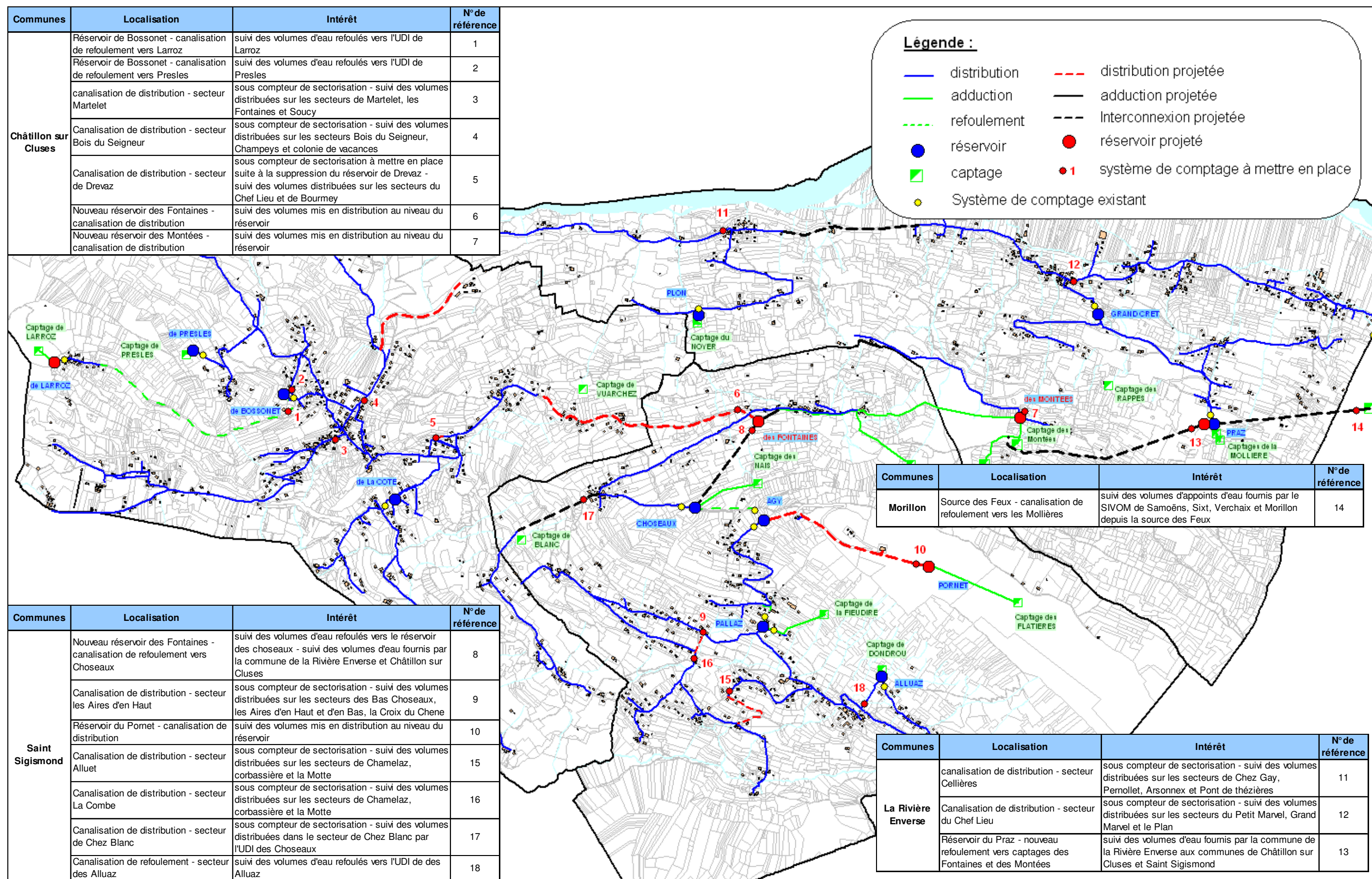
Figure 18 : localisation et description des systèmes de comptage à mettre en place
