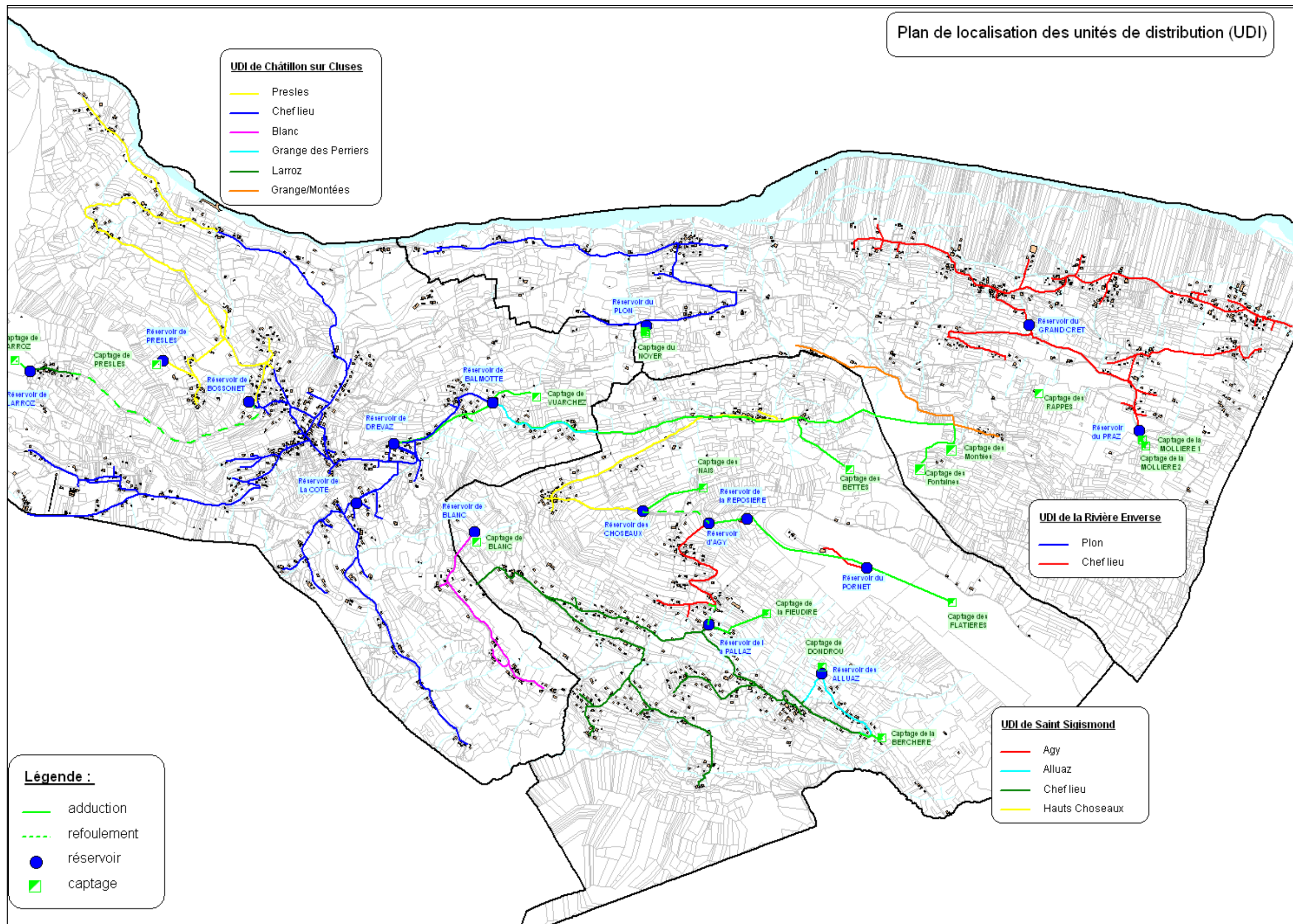
Figure 4 : schéma de localisation des unités de distribution (UDI)
