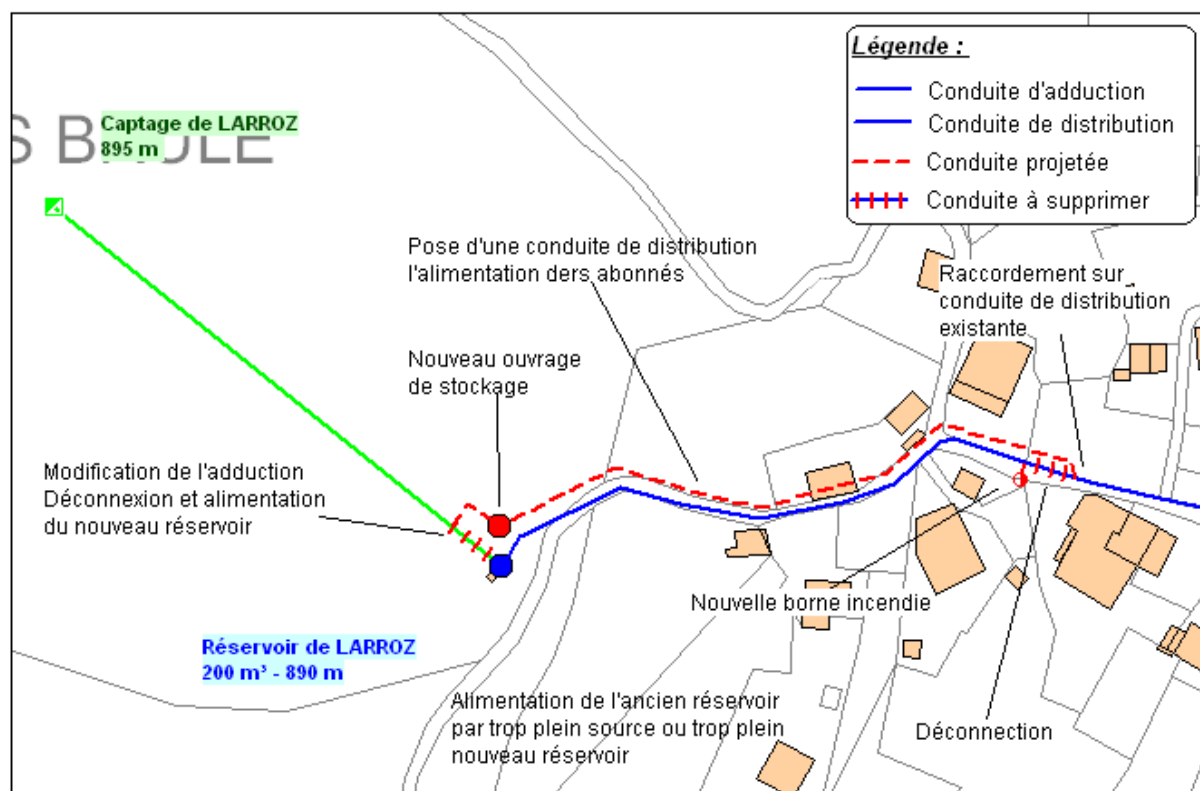
Figure 20 : mise en conformité de la défense incendie du secteur de distribution de Larroz
