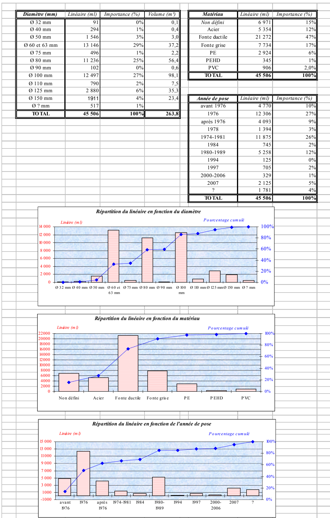
Graphique 4 : répartition du linéaire en fonction des diamètres, matériaux et années de pose des canalisations de distribution
