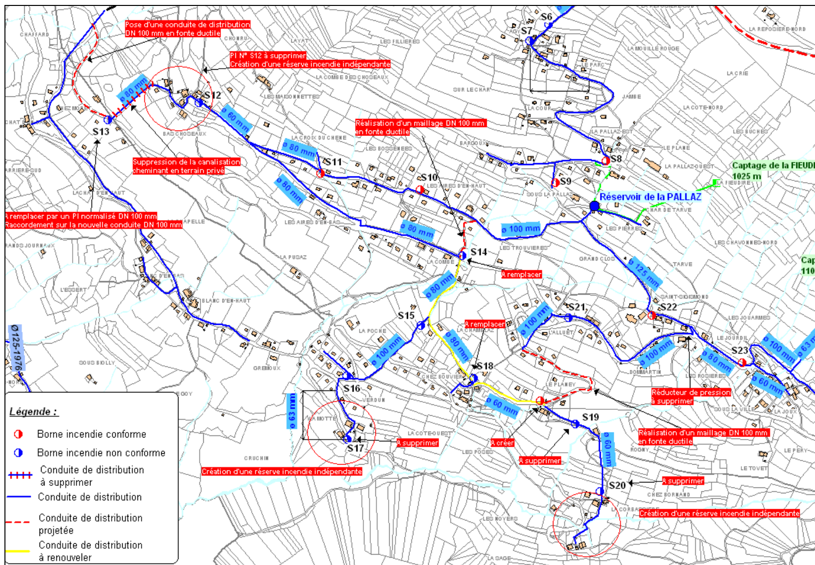
Figure 23 : localisation et description des actions à engager dans le cadre de la mise aux normes de la défense incendie de l'UDI de la Pallaz
