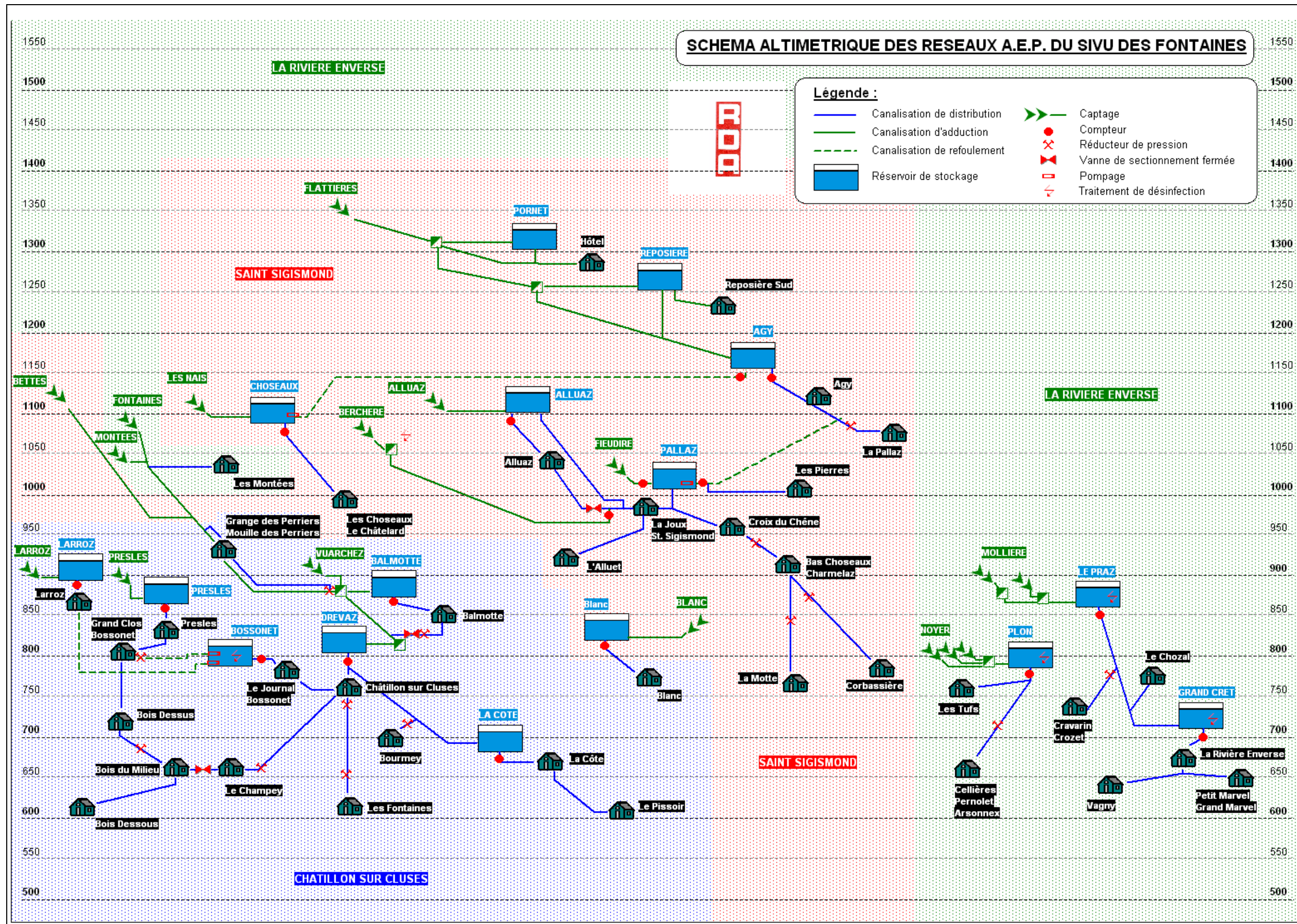
Figure 3 : schéma altimétrique du réseau AEP du SIVU des Fontaines
