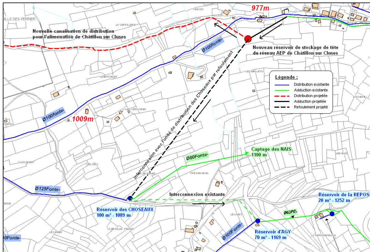
Figure 11 : interconnexion des réseaux de Châtillon sur Cluses et de Saint Sigismond - situation projetée
