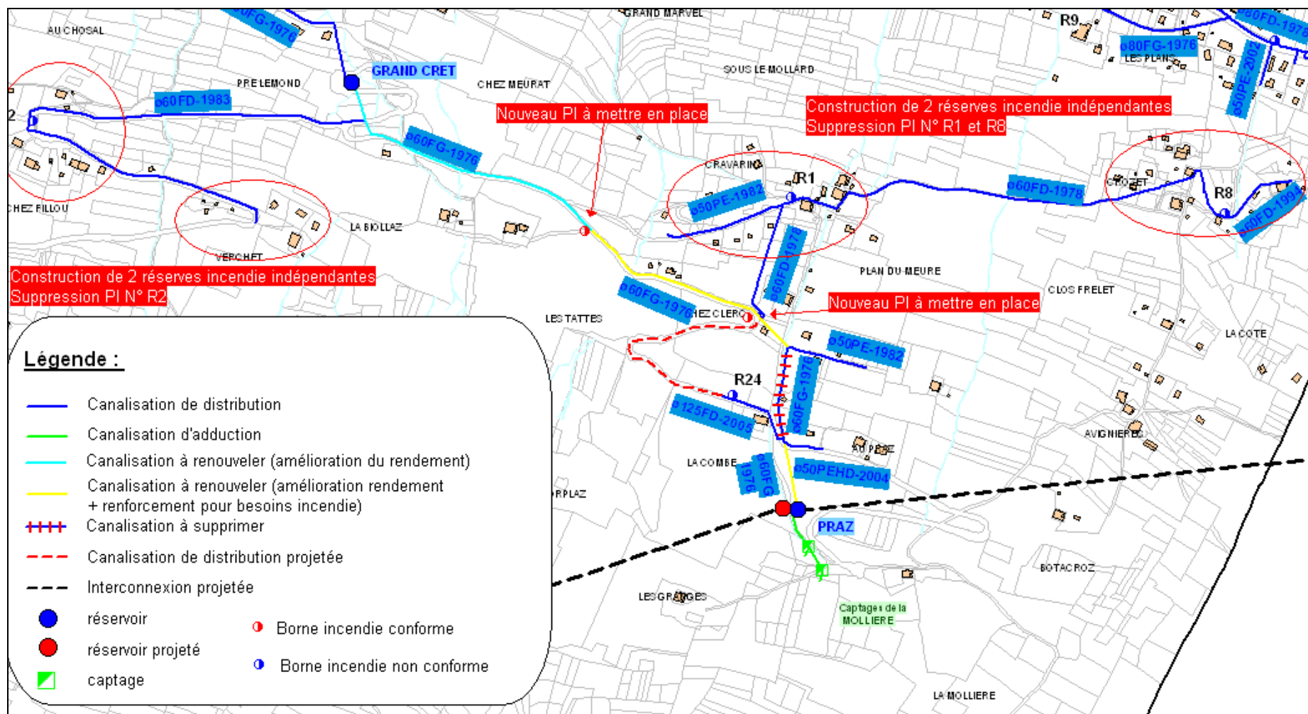
Figure 24 : localisation et description des actions à engager dans le cadre de la mise aux normes de la défense incendie de l'UDI du Praz
