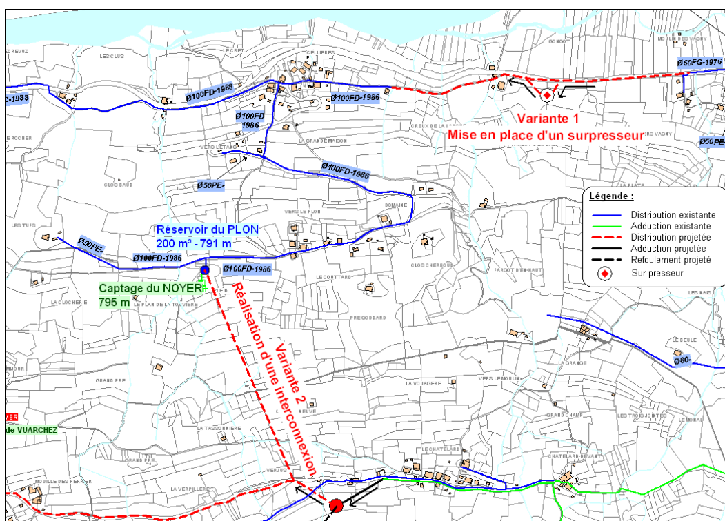
Figure 15 : sécurisation de l'alimentation en eau potable du secteur de distribution du Plon
