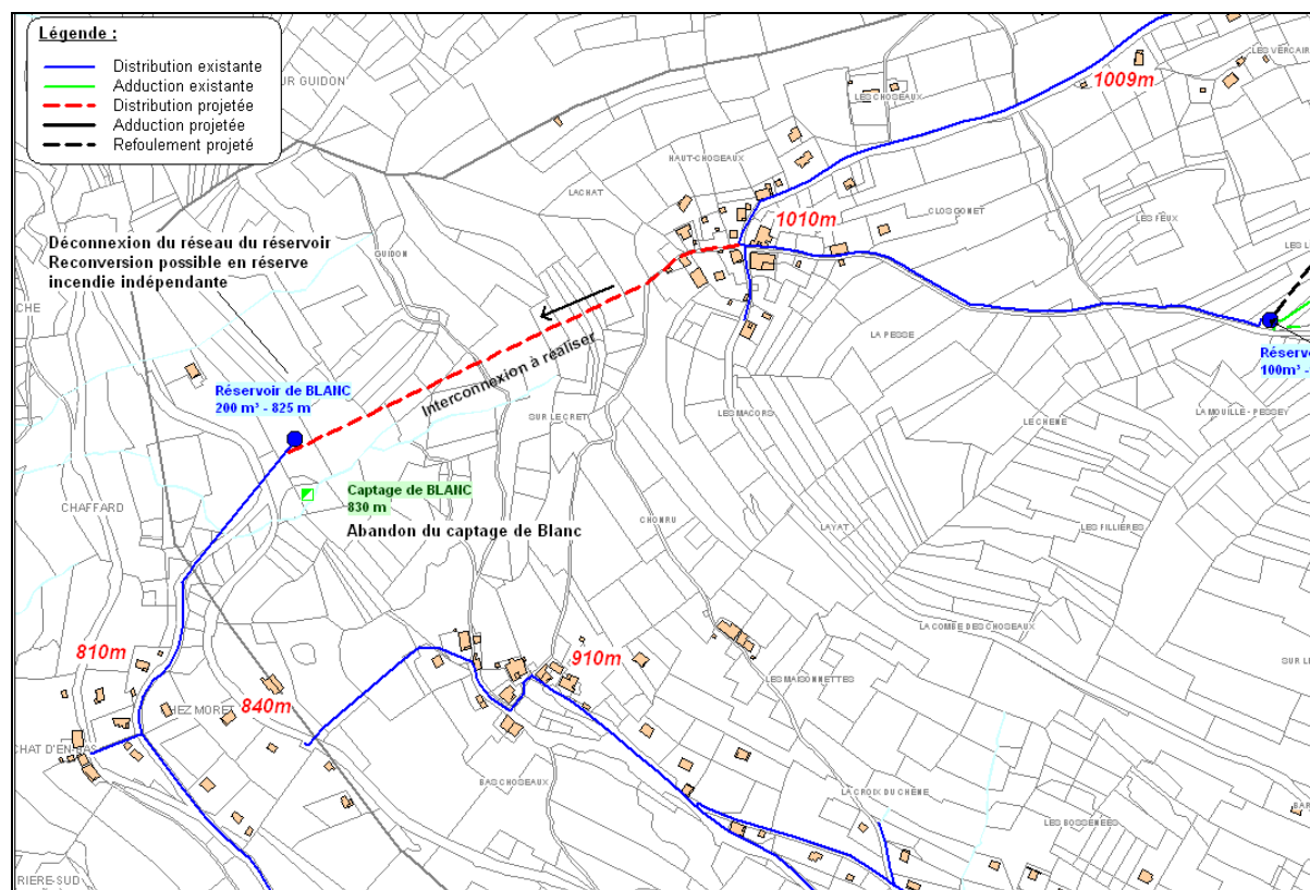
Figure 12 : interconnexion de l'unité de distribution de Chez Blanc avec celle des Choseaux
