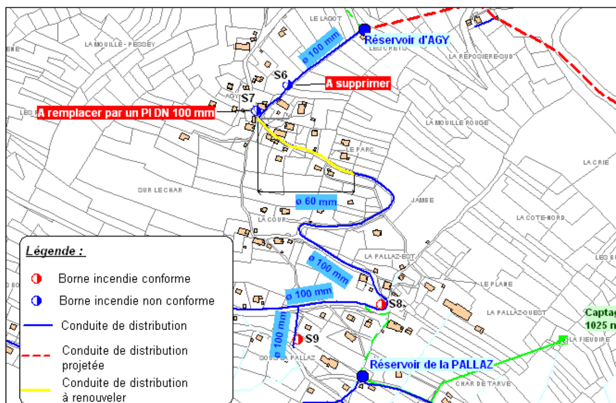
Figure 22 : localisation des actions à engager dans le cadre de la mise aux normes de la défense incendie de l'UDI d'Agly
