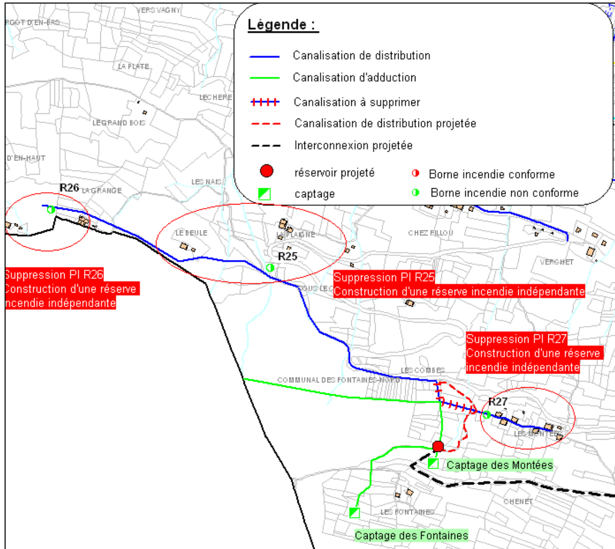
Figure 21 : localisation et description des actions à engager dans le cadre de la mise aux normes de la défense incendie des secteurs des Montées et de la Grange
