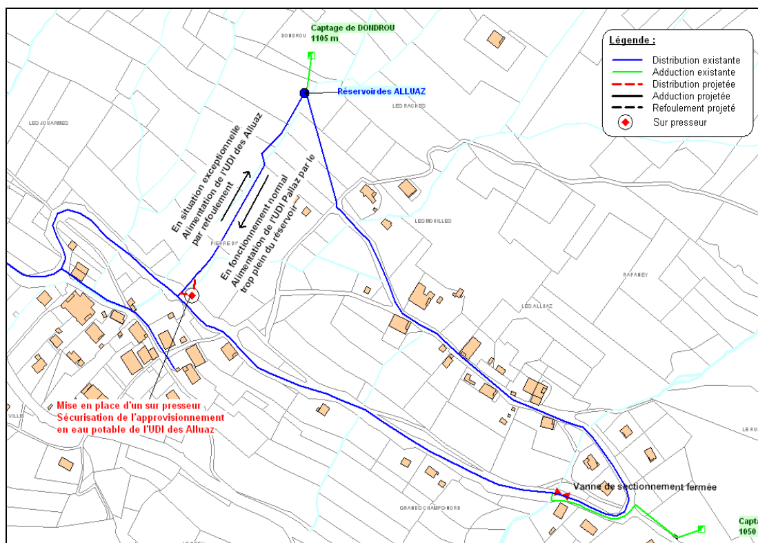
Figure 14 : sécurisation de l'approvisionnement en eau potable de l'unité de distribution des Alluaz - situation projetée
