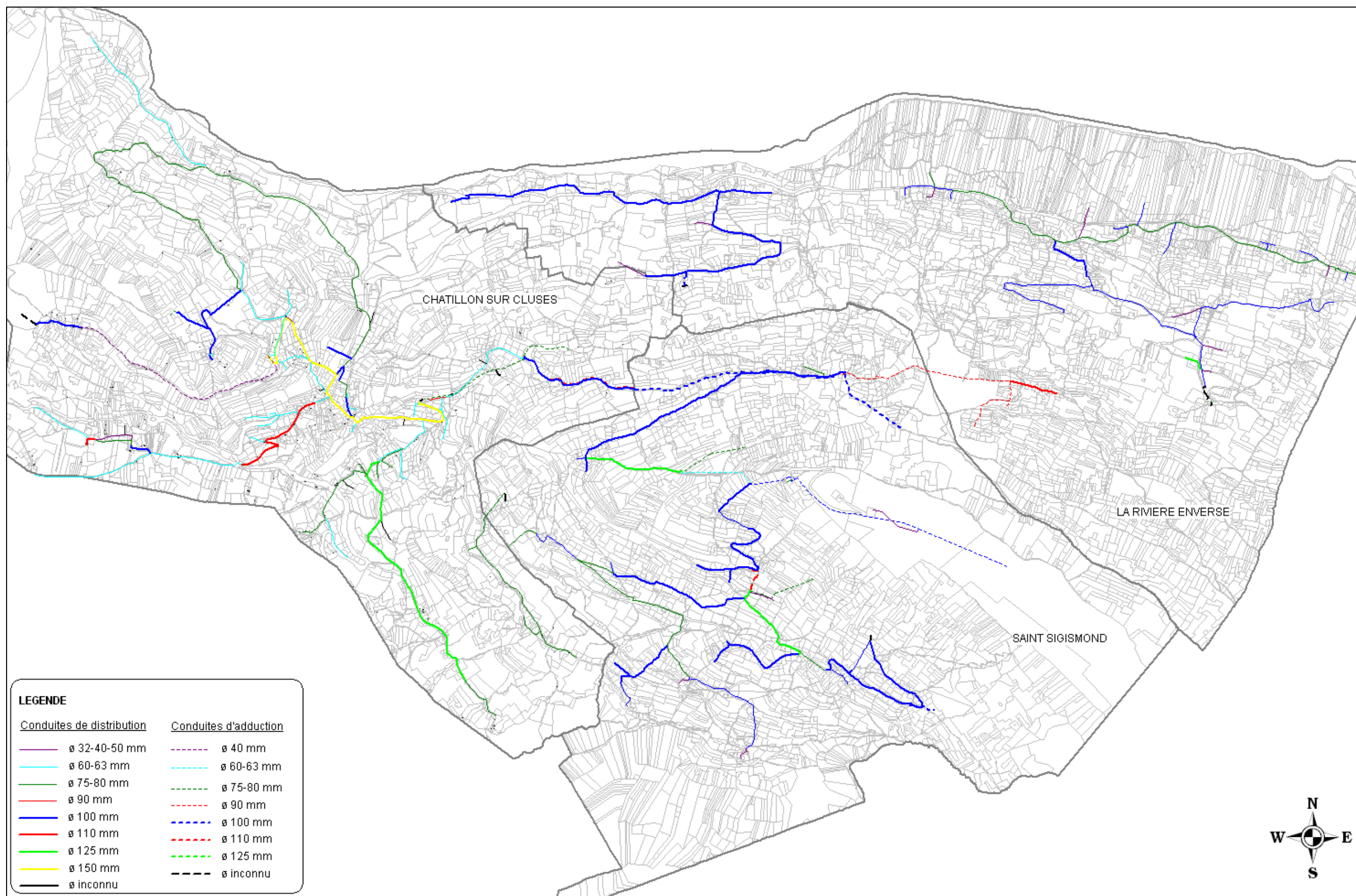
Figure 5 : répartition du linéaire de canalisations d'adduction, de refoulement et de distribution en fonction des diamètres
