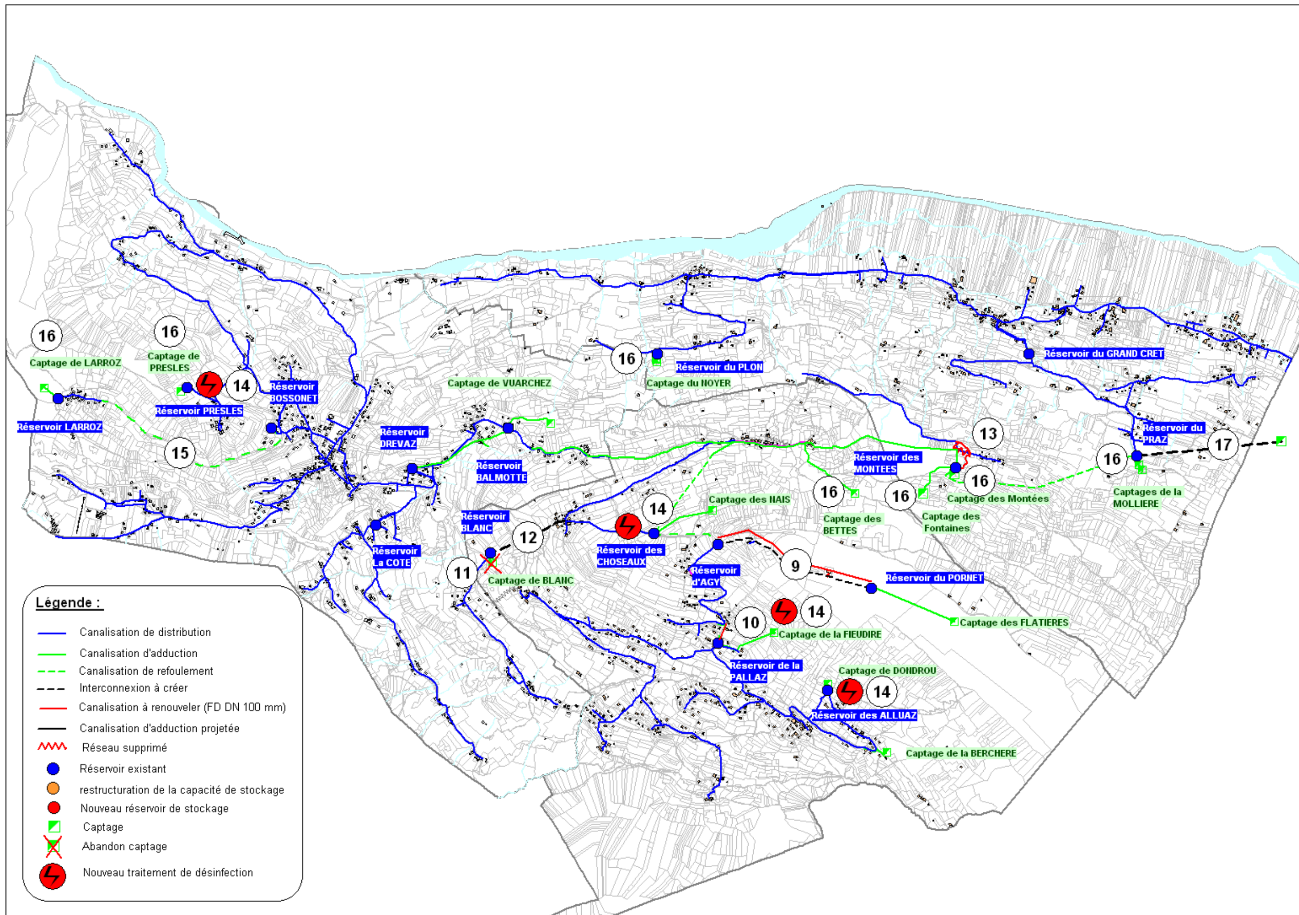
Figure 27 : localisation des actions à mener en priorité 1.2
