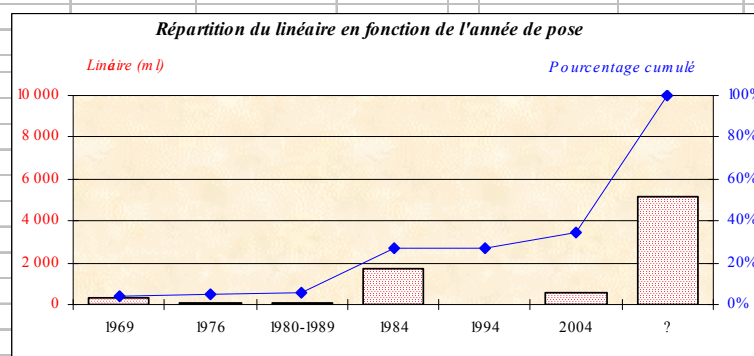
Graphique 3 : répartition du linéaire de canalisations d'adduction en fonction des diamètres, matériaux et années de pose
