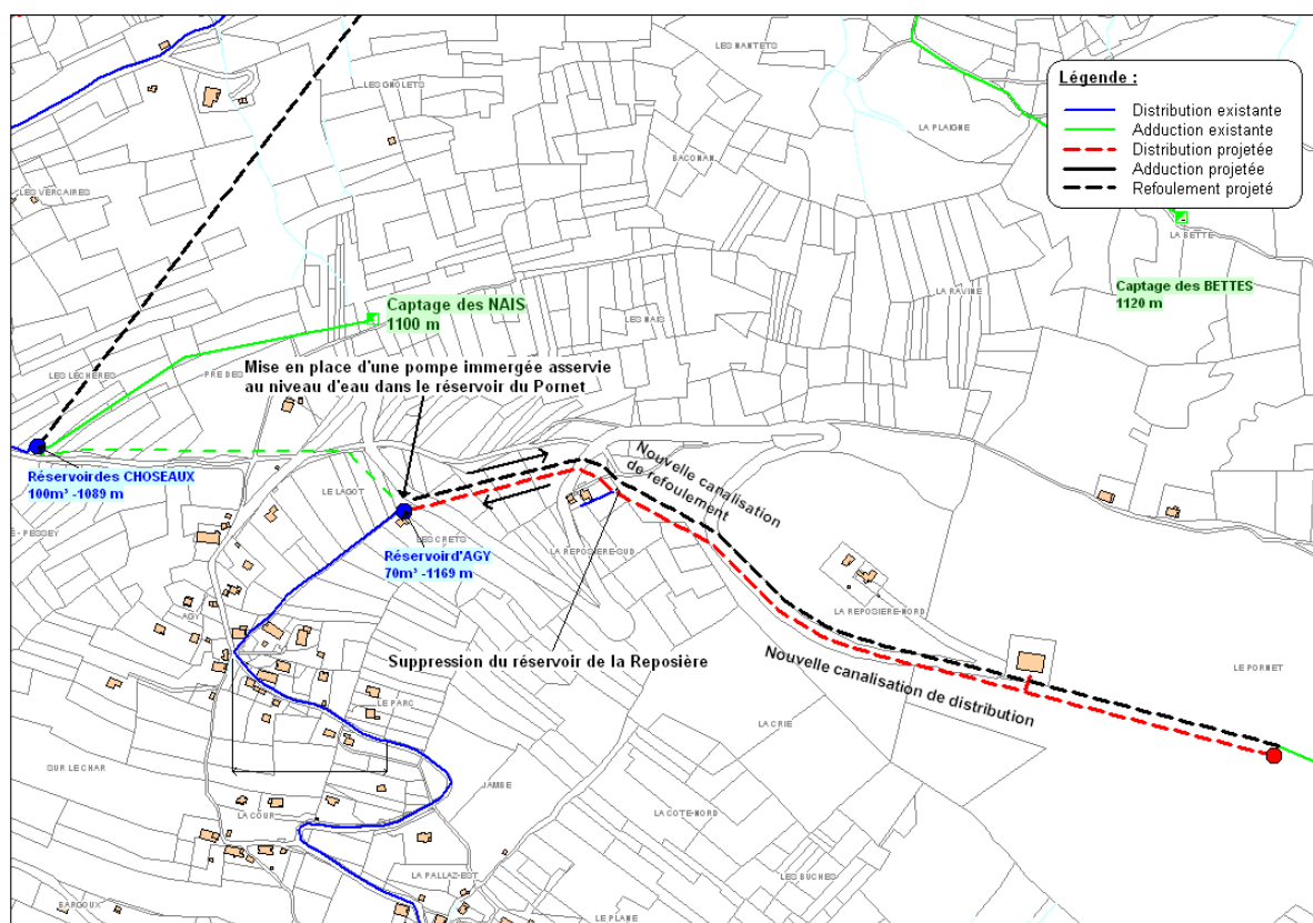
Figure 13 : sécurisation de l'approvisionnement en eau potable du secteur de distribution du Pornet- situation projetée
