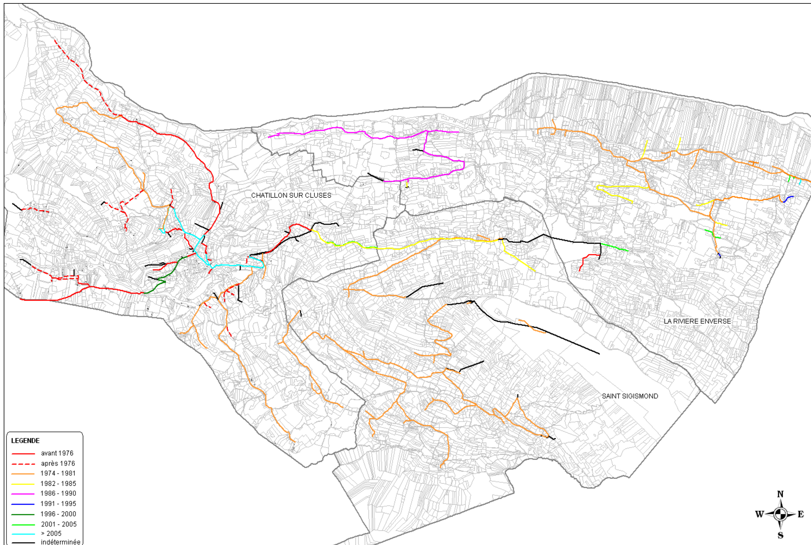
Figure 6 : répartition du linéaire de canalisations d'adduction, de refoulement et de distribution en fonction des années de mises en service
