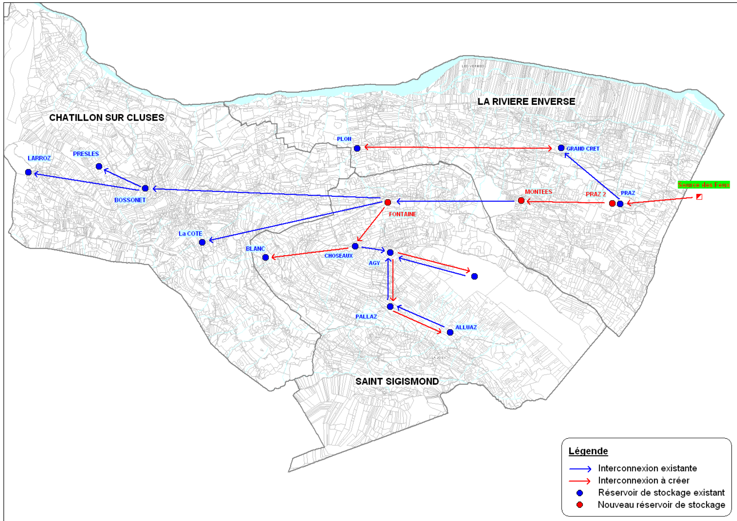
Figure 16 : interconnexions et sens de circulation de l'eau
