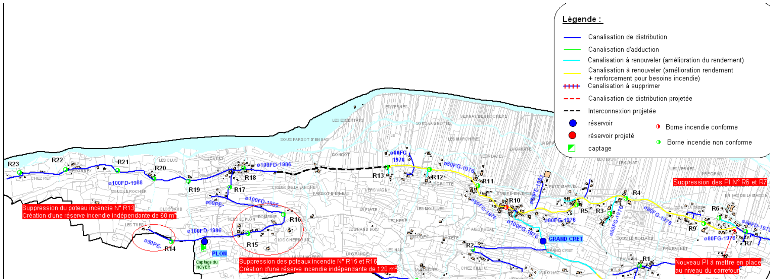
Figure 25 : localisation et description des actions à engager dans le cadre de la mise aux normes de la défense incendie des secteurs du Plon et du Grand Crêt
