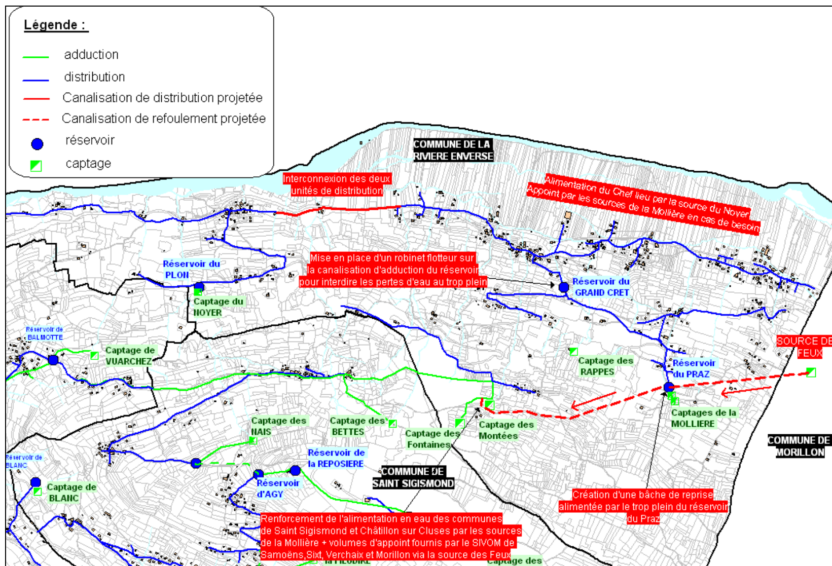
Figure 9 : aménagements à prévoir sur le territoire communal de la Rivière Enverse pour assurer l’approvisionnement des communes de Saint Sigismond et Châtillon sur Cluses
