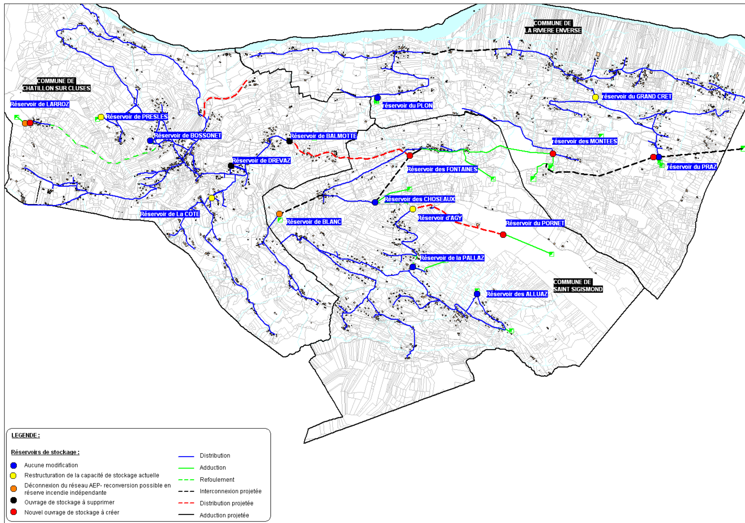
Figure 10 : restructuration de la capacité de stockage - situation projetée
