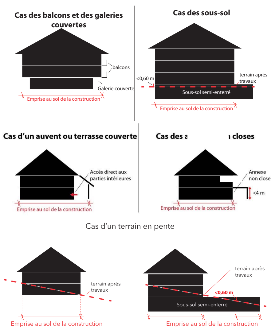
Schéma explicatif
