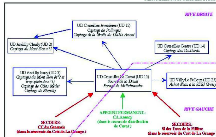
Synoptique simplifié du réseau d'eau potable Source : annexes sanitaires
