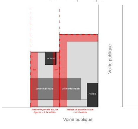
Art. 1AUB7 – Implantations du bâtiment principal
