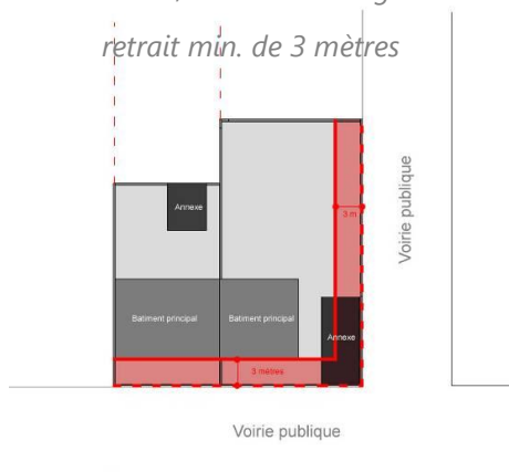
Art. UB6 - Implantation des constructions en retrait de 3 mètres ; Annexes à l’alignement ou en
