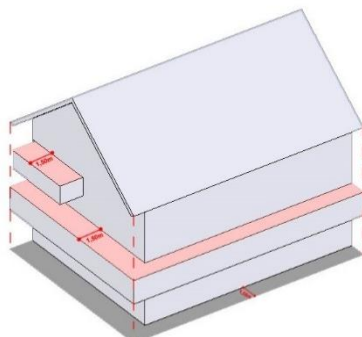
Les saillies en façade sont limitées à 1,50 mètres et doivent être couvertes par la toiture
