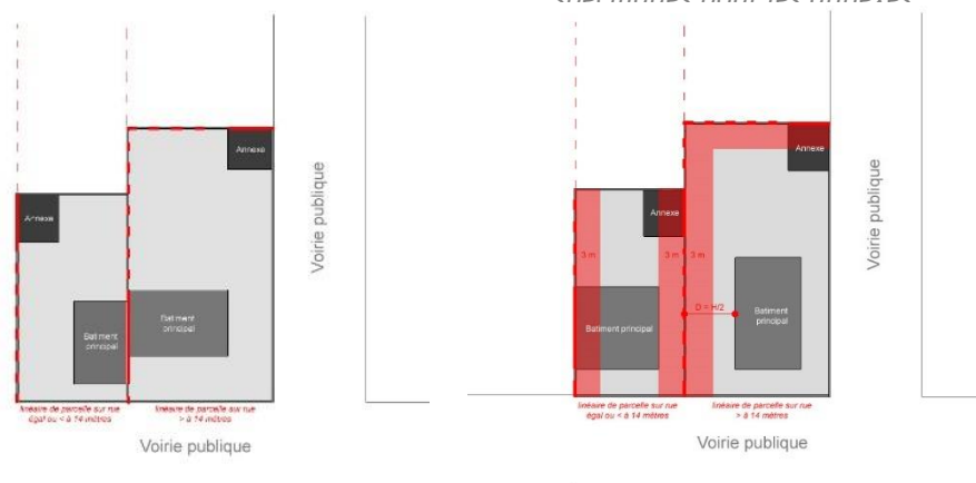
Art. 1AUB7– Implantations spécifiques pour les annexes
