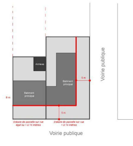
Art. 1AUa6 – implantation en retrait de 5 mètres
