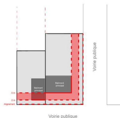
Art. AHa6 – Implantations autorisées
