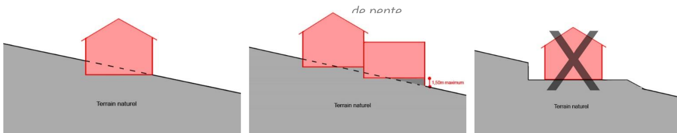
Mode d'implantation des constructions sur les terrains > 10%
