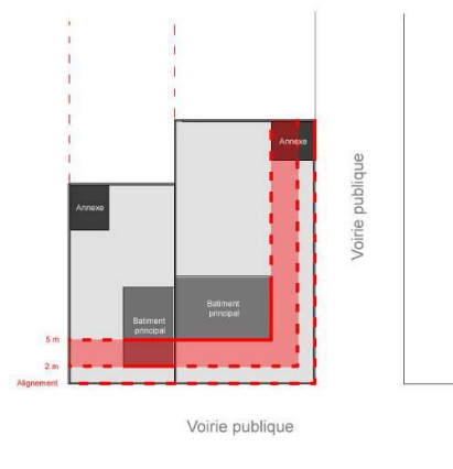
Art. UB6 – Implantations autorisées
