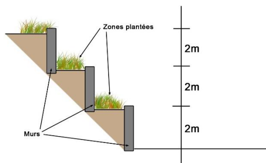
Les murs de soutènement en enrochement ou gabions
