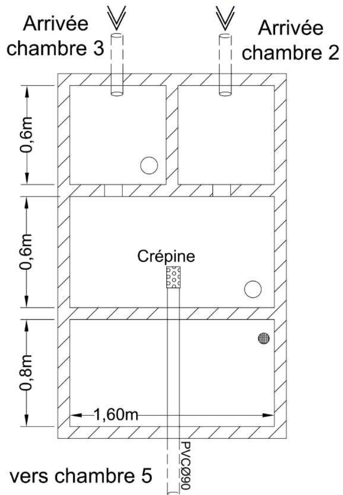
Schéma de l'ouvrage
