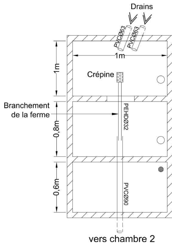
Schéma de l'ouvrage
