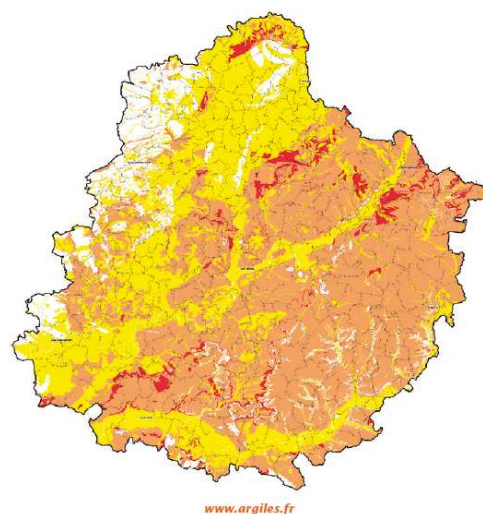
Carte départementale de l'aléa retrait gonflement des argiles
