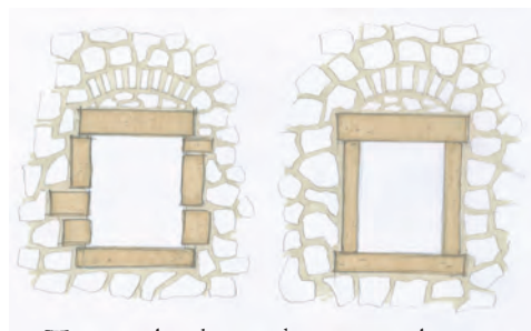
Exemple de jambages et linteaux en pierre ou en bois
