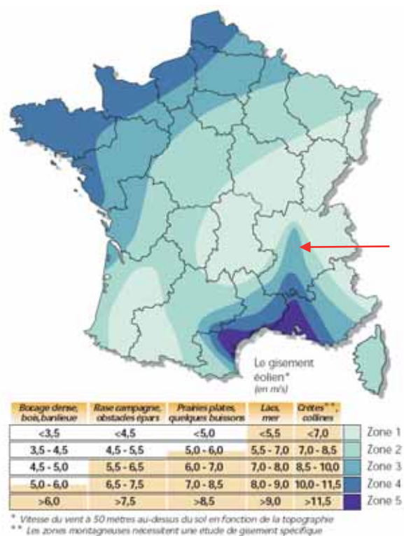
Le gisement éolien en France en m/s. Source SFE
