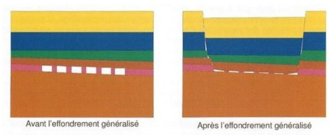
Figure 3 : Effondrement généralisé
