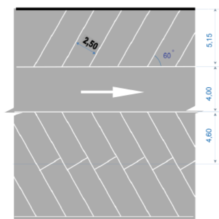
Stationnement en épi à 60°
