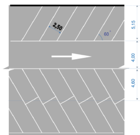
Stationnement en épi à 60°
