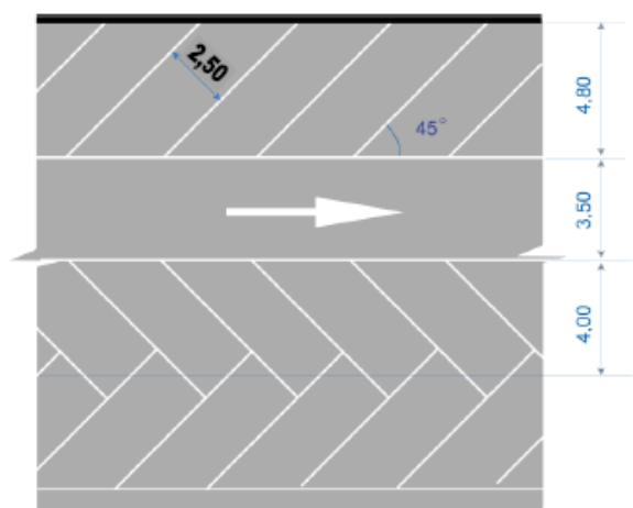
Stationnement en épi à 45°
