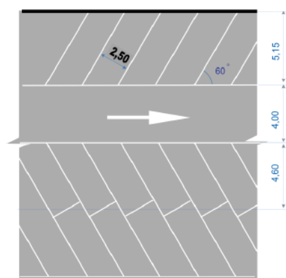
Stationnement en épi à 60°
