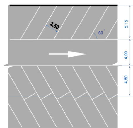
Stationnement en épi à 60°
