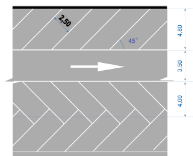
Stationnement en épi à 45°
