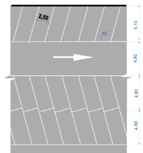
Stationnement en épi à 75°
