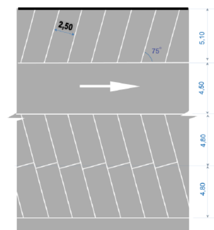
Stationnement en épi à 75°
