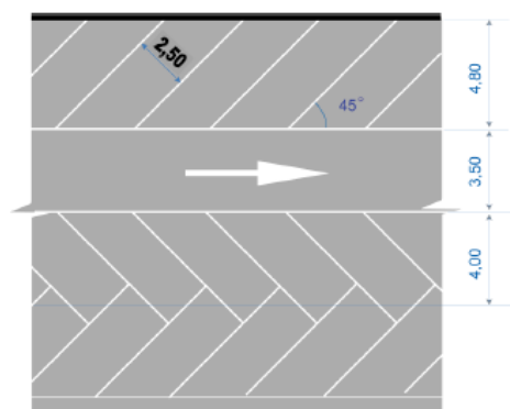
Stationnement en épi à 45°
