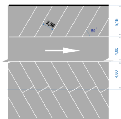
Stationnement en épi à 60°
