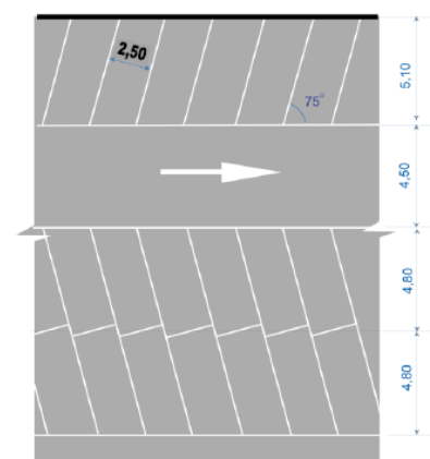
Stationnement en épi à 75°
