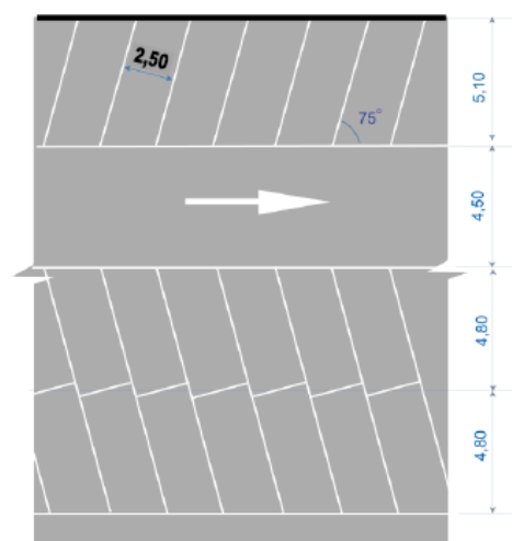
Stationnement en épi à 75°
