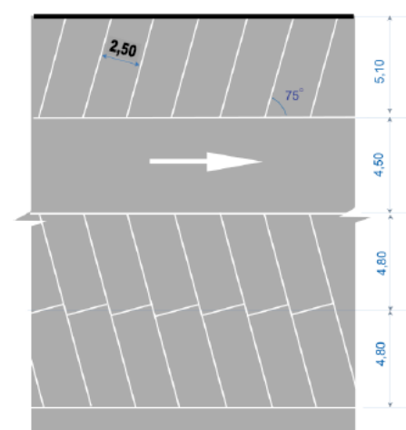
Stationnement en épi à 75°
