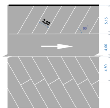
Stationnement en épi à 60°
