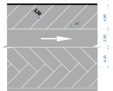
Stationnement en épi à 45°
