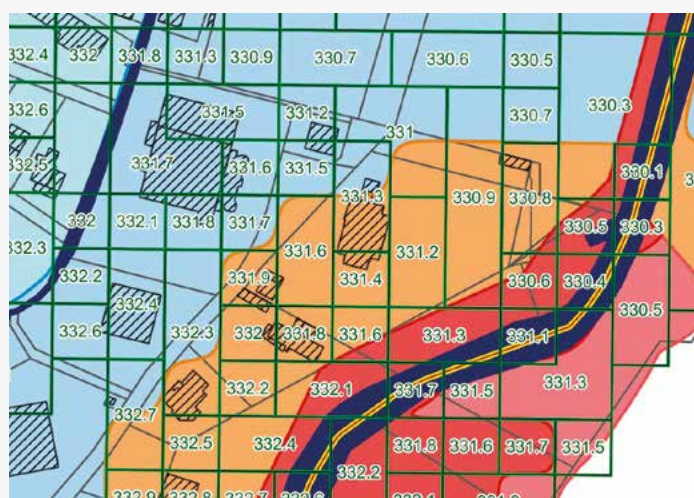
Figure 6 : Extrait de la planche 03 (les CPHE* représentées n'incluent pas la revanche de 0,30 mètre)
