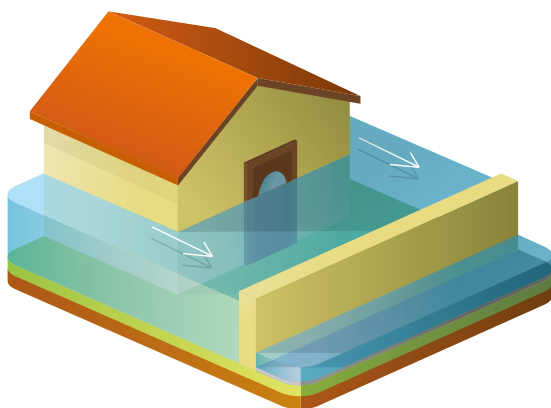
Figure 3 : Exemple de clôture qui n'assure pas la transparence hydraulique.
