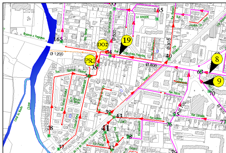
Figure 2-27 : Localisation du poste de relèvement PR2
