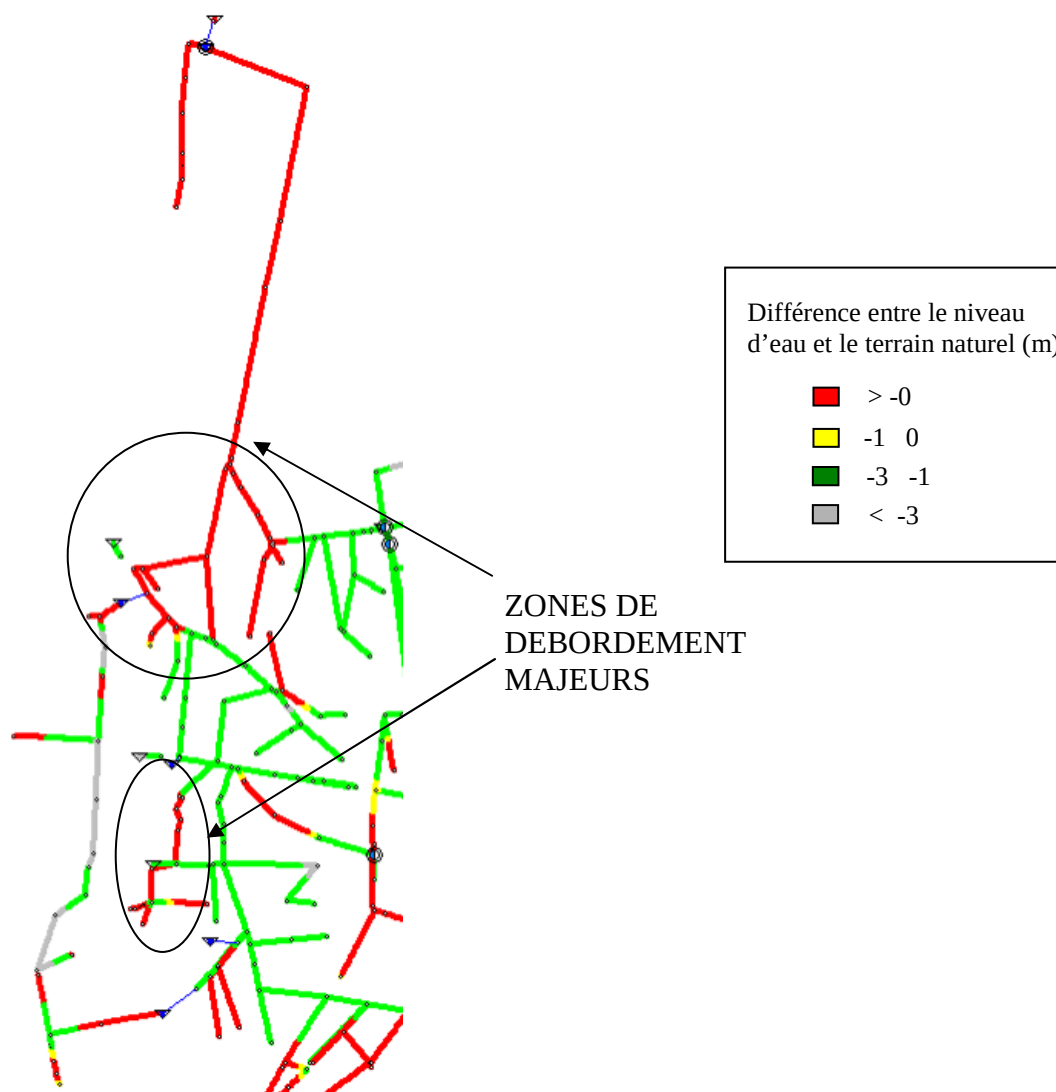
Figure 7-1 : Simulation d'une pluie décennale en fermant les déversoirs d'orage
