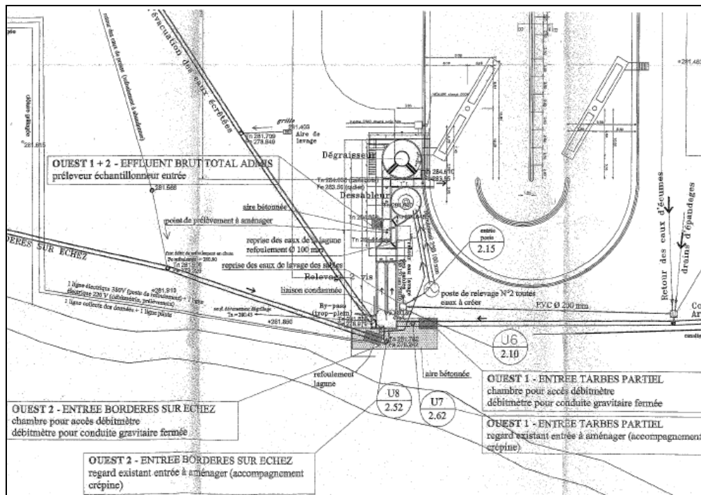
Figure 2-14 : Plan descriptif des ouvrages à l'entrée de la STEP de Tarbes Ouest
