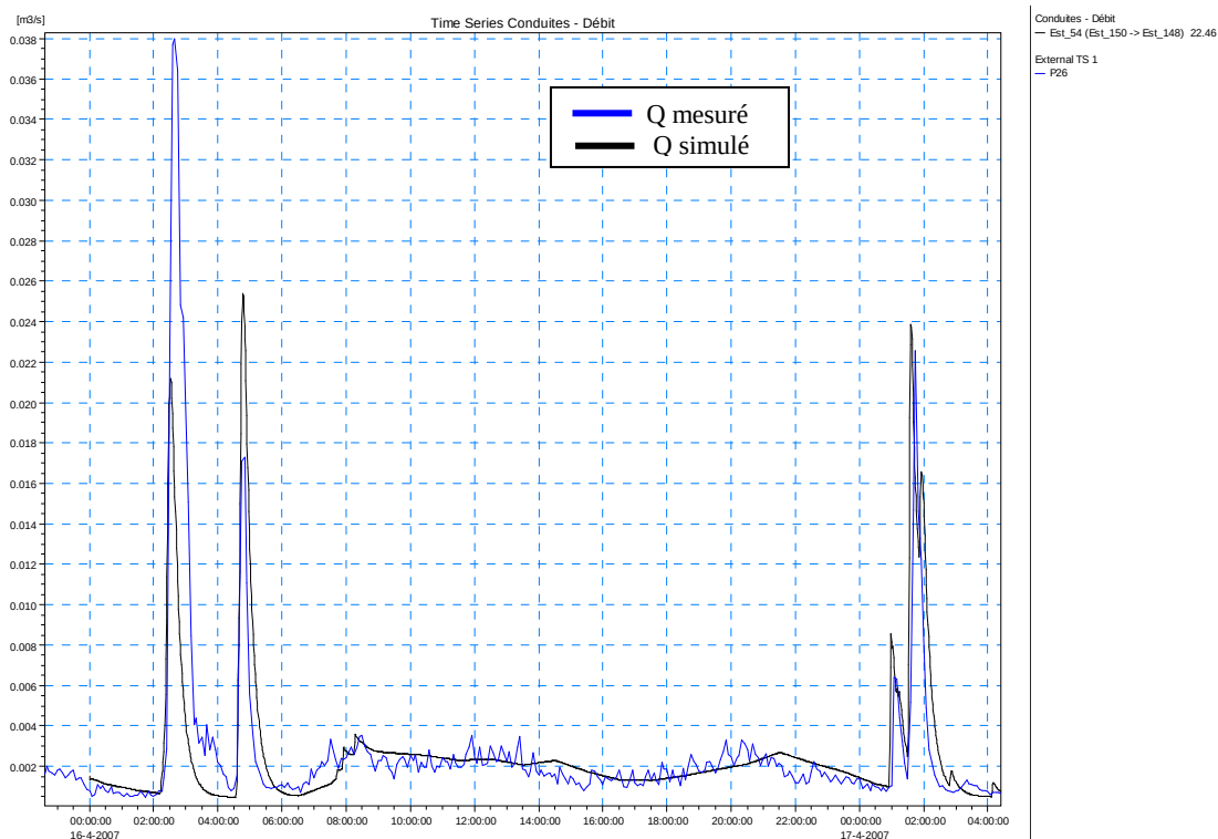
Figure 3-9 : Débit au point P26 le 17/04/2007
