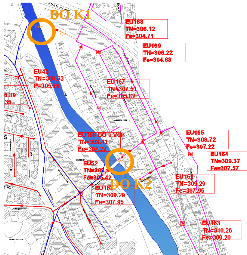
Figure 2-17 : Localisation des déversoirs DOK1 et DOK2
