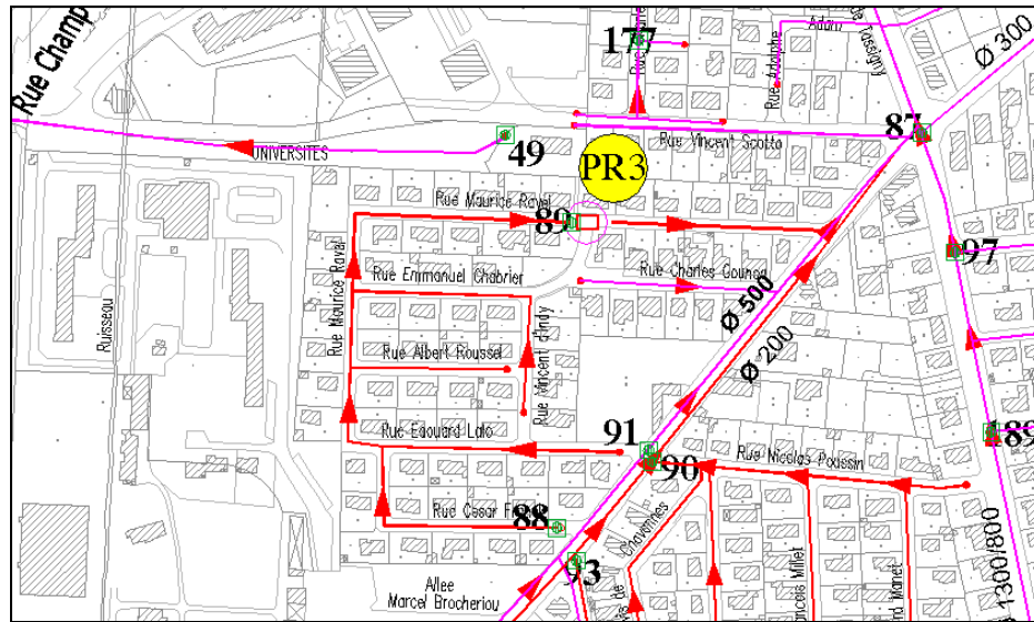
Figure 2-28 : Localisation du poste de relèvement PR3
