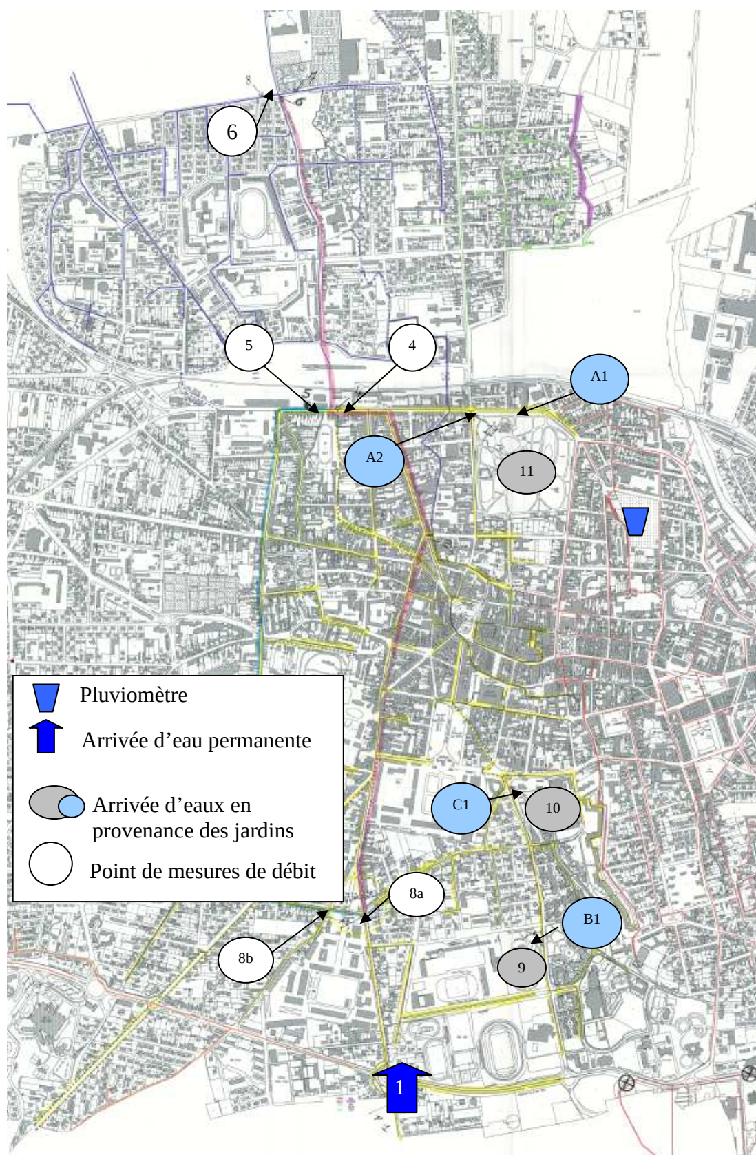
Figure 2-36: Localisation des points de mesures sur le réseau pluvial
