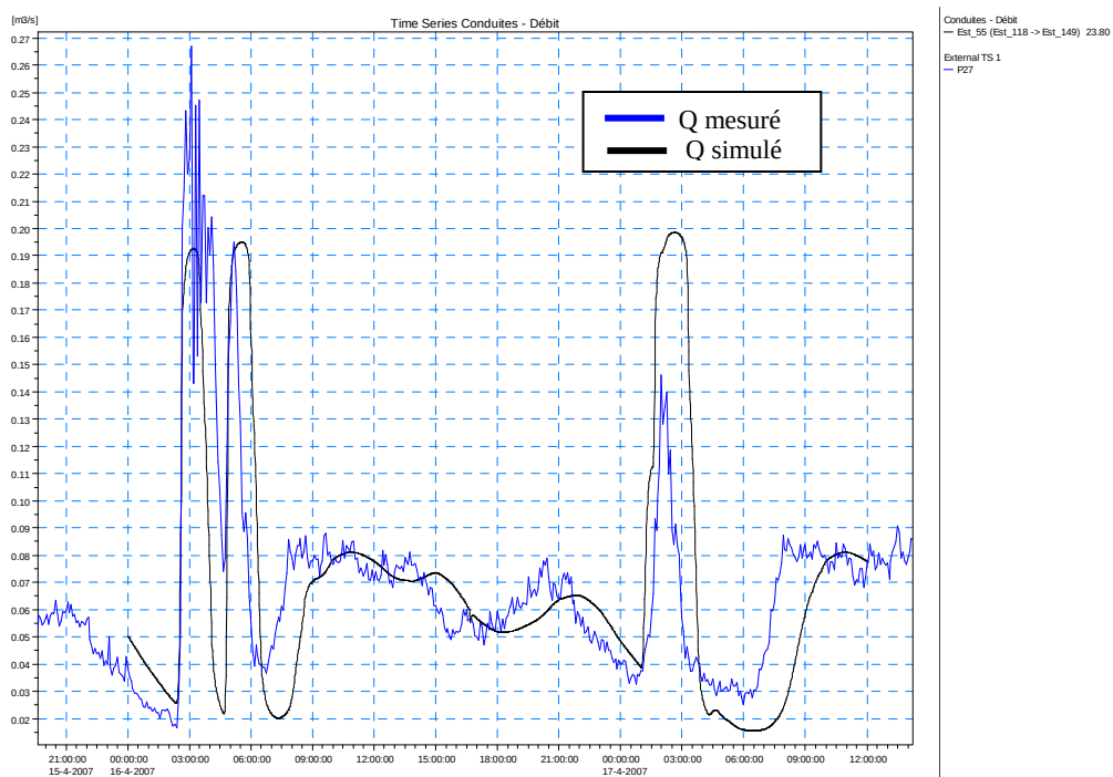
Figure 3-8 : Débit au point P27 le 17/04/2007
