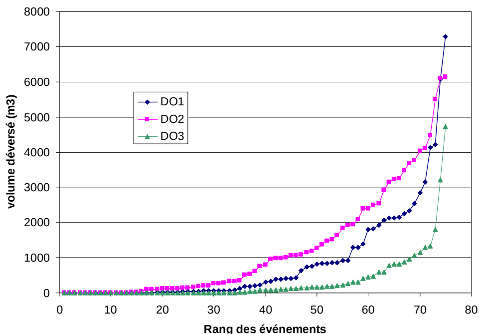
Figure 6-8 : Volume rejeté par déversoir selon le nombre d'événements pluvieux
