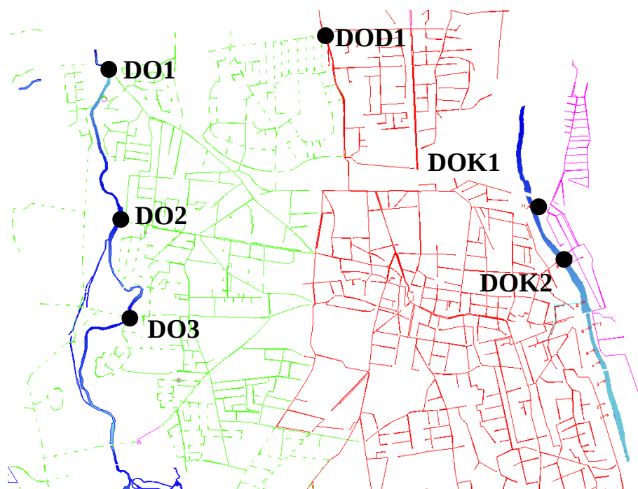
Figure 6-2 : Localisation des déversoirs instrumentés pour la mesure en continu sur le réseau d'assainissement
