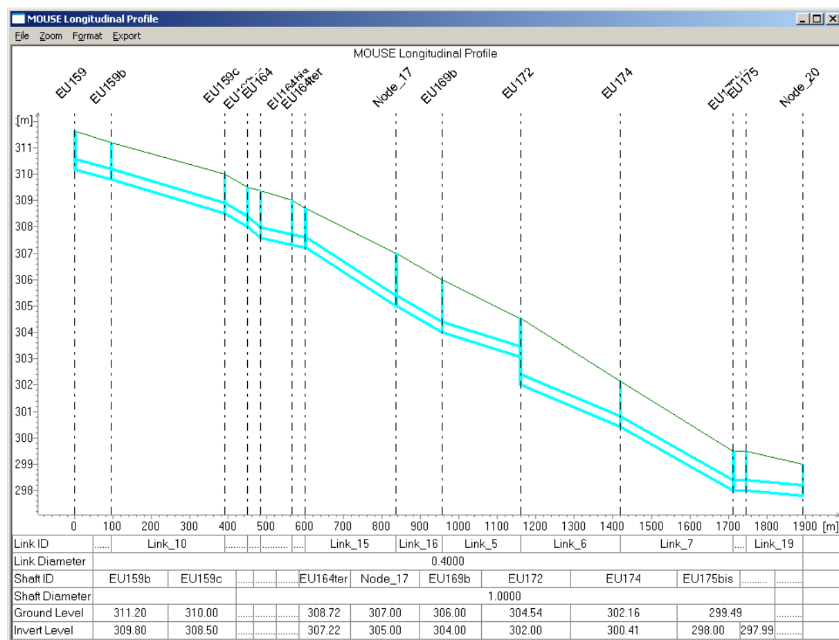
Figure 5-2 : Profil 1 : DN400 de l'avenue de la Marne à l'exutoire
