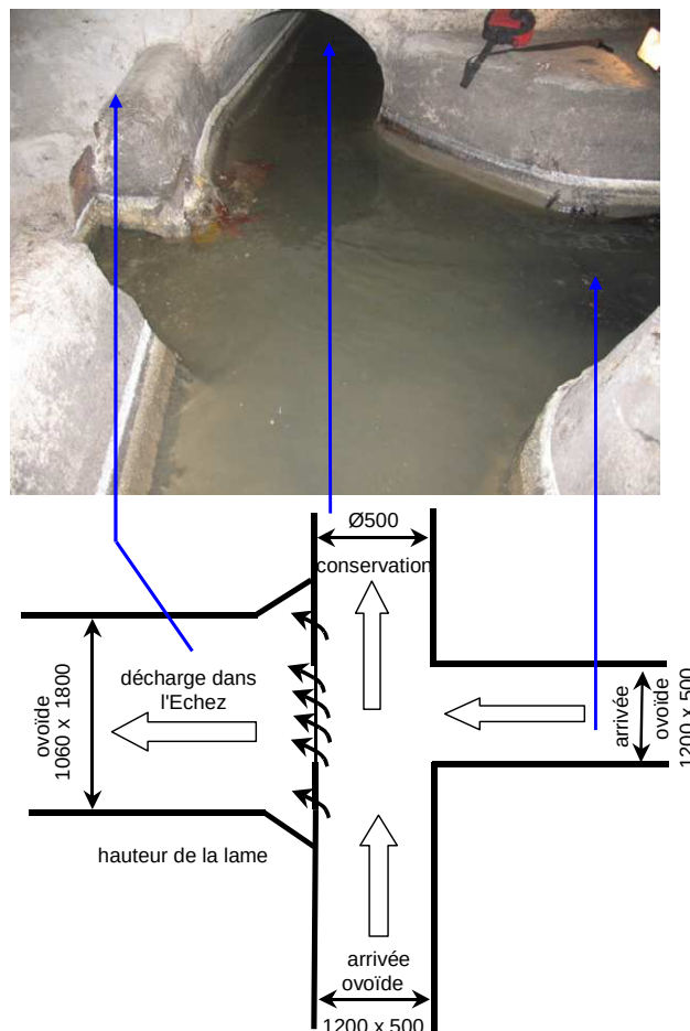
Figure 2-13 : Photographie et schéma du déversoir d'orage DO3
