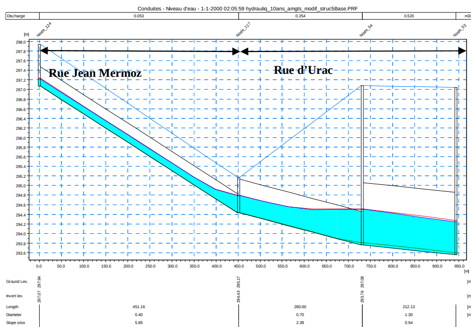
Figure 4-8 : Ligne d'eau suite à la simulation de l'aménagement B rue d'Urac
