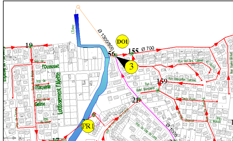
Figure 2-8 : Localisation du déversoir d'orage DO1
