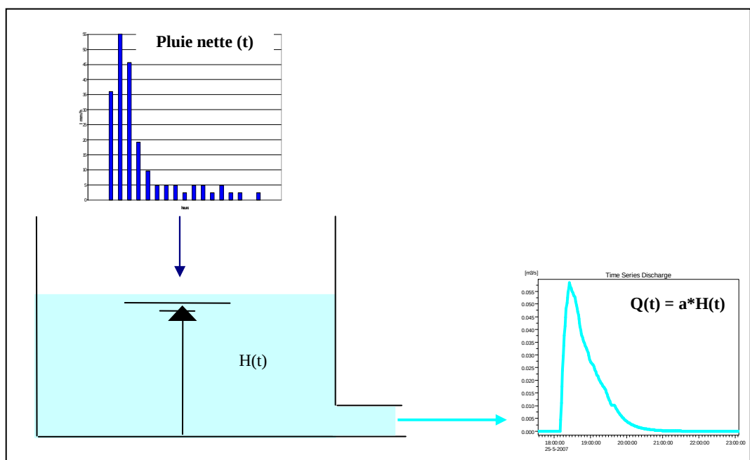
Figure 2-2 : Modèle du réservoir linéaire
