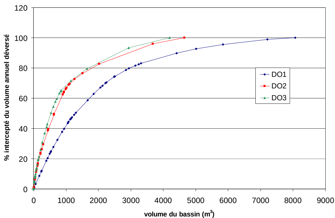
Figure 7-6 : Courbe d'efficacité de bassins placés à chacun des déversoirs d'orage (rehaussés) DO1, DO2, DO3.
