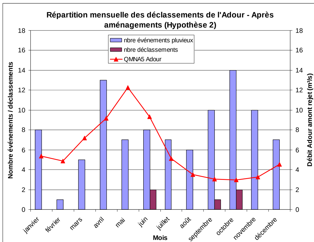
Figure 7-20 : Répartition mensuelle des déclassements de l'Adour – Rejets pluviaux – Base QMNA5
