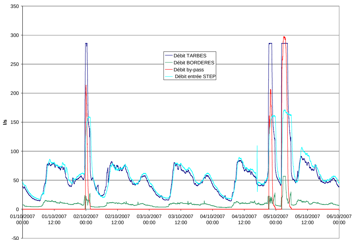
Figure 3-1 : Mesures de l'exploitant en entrée de la station de Tarbes Ouest
