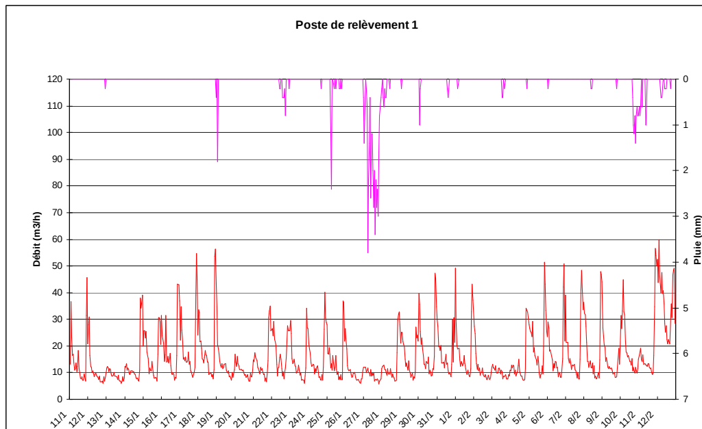
Figure 2-26 : Fonctionnement du PR1 du 11/01 au 12/02/07
