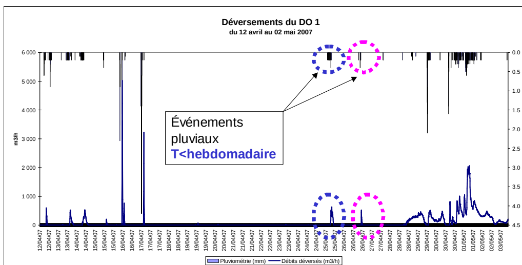
Figure 6-3 : Enregistrement des déversements au DO1
