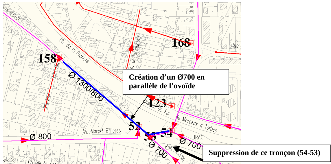
Figure 4-7 : Proposition B d'aménagement rue d'Urac
