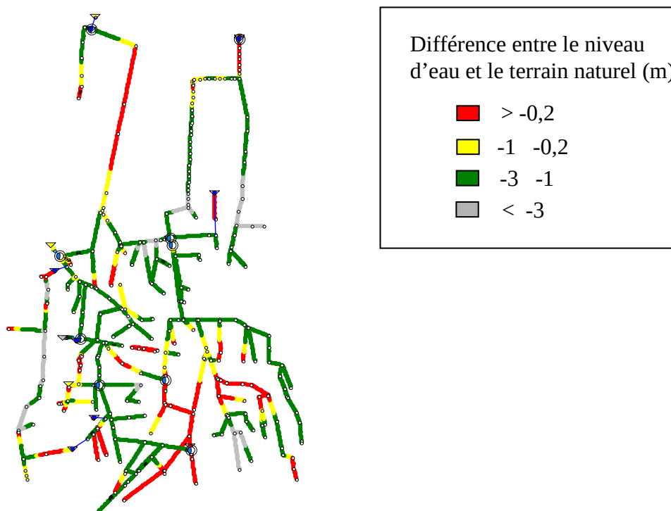
Figure 4-2 : Niveau de remplissage maximal des conduites – Pluie décennale – Situation future de référence
