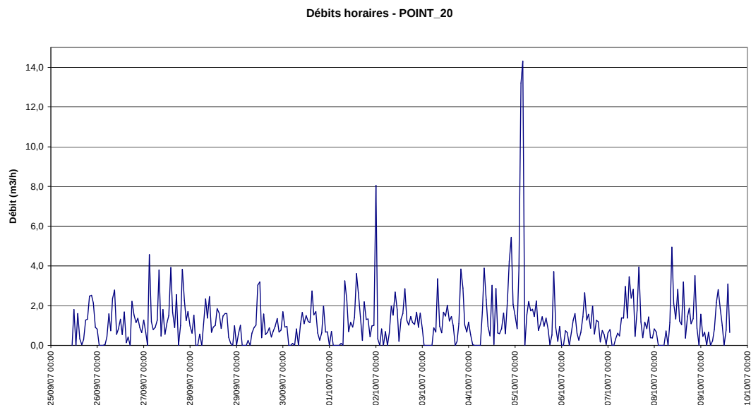
Figure 2-33 : Débits mesurés sur le point 20 lors de la deuxième campagne de mesures
