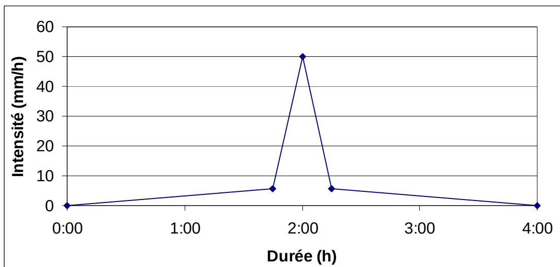
Figure 4-1 : HyétoGramme – Pluie de projet décennale
