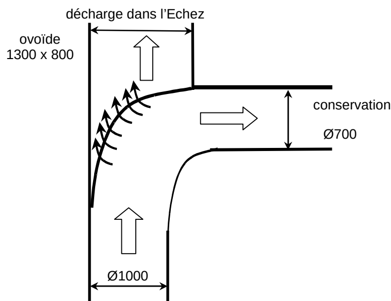
Figure 2-9 : Schéma de fonctionnement du DO1
