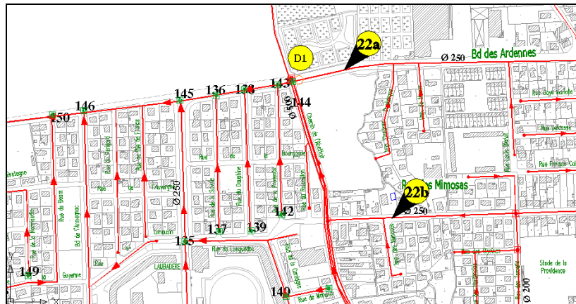
Figure 2-19 : Localisation du répartiteur de débit D1
