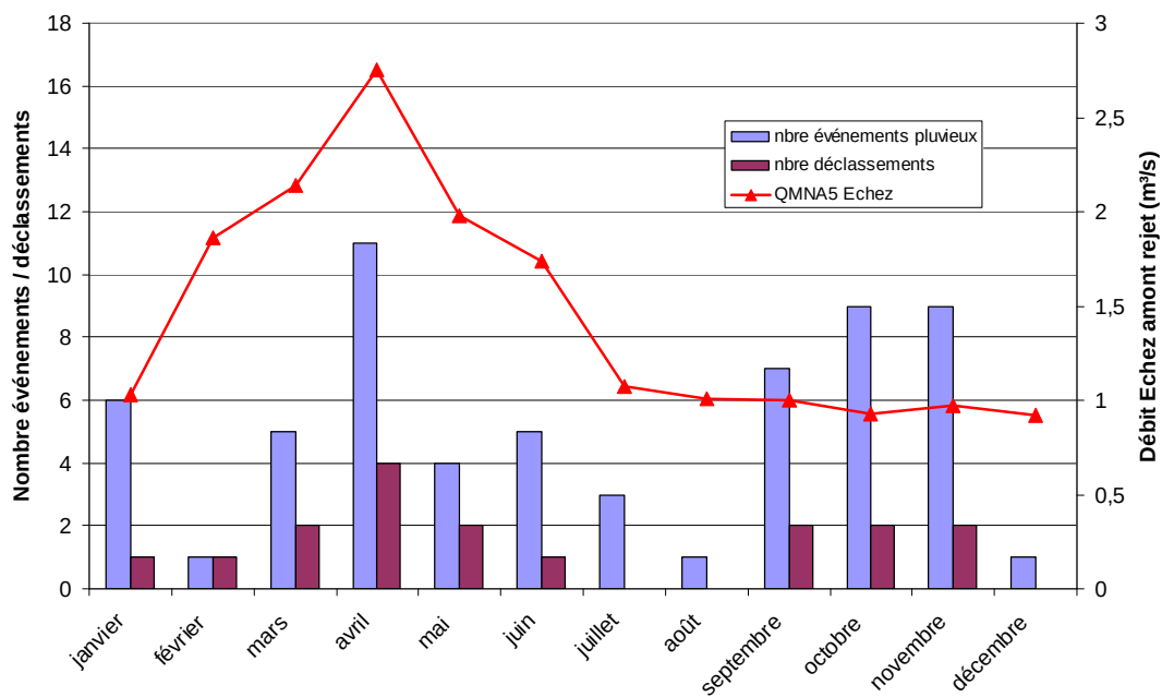
Figure 7-11 : Répartition mensuelle des déclassements de l'Echez – Rejets unitaires – Base QMNA5
