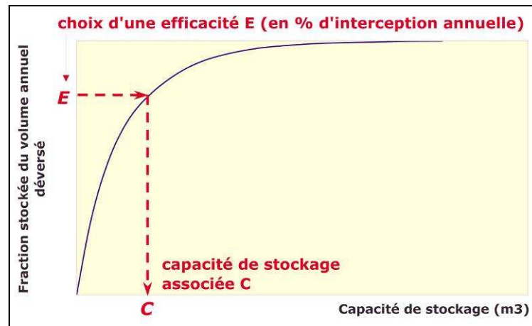
Figure 7-5 : Exemple : Lien efficacité-capacité de l'ouvrage de stockage-dépollution
