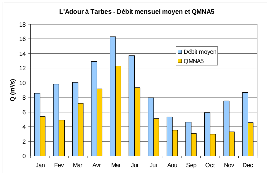
Figure 7-16 : Débits de l'Adour à Tarbes
