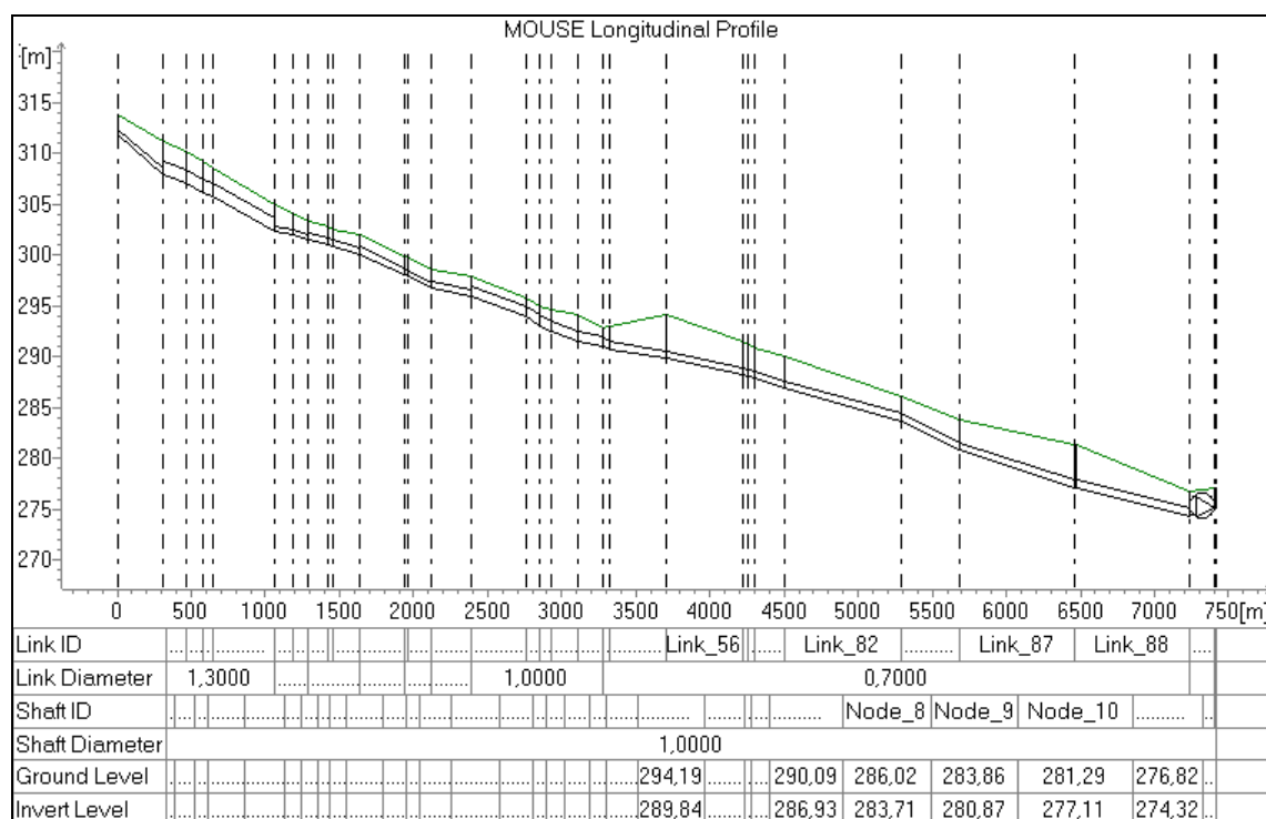
Figure 2-5 : Profil en long d'un collecteur modélisé sous MikeUrban (collecteur principal réseau Ouest, du regard 100 à la STEP)
