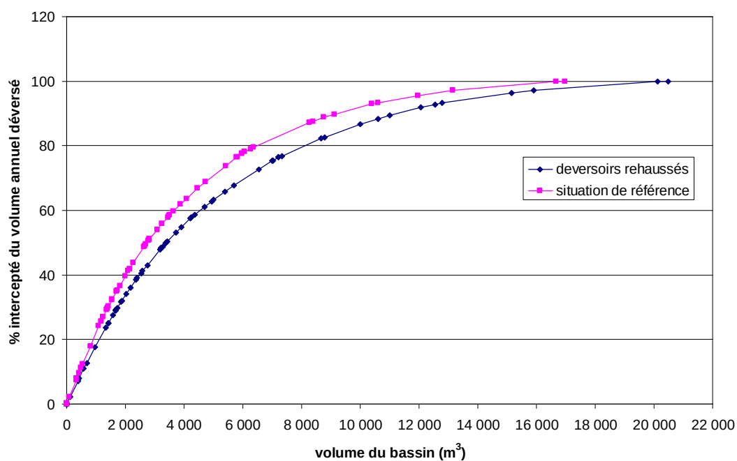
Figure 7-7 : Effets de l'augmentation du niveau des seuils des déversoirs sur l'efficacité de stockage au by pass de la station d'épuration en situation de référence et en situation de référence avec déversoirs rehaussés.
