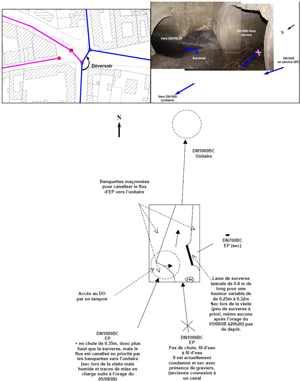
Figure 2-24 : Localisation de la surverse rue Sainte Catherine
