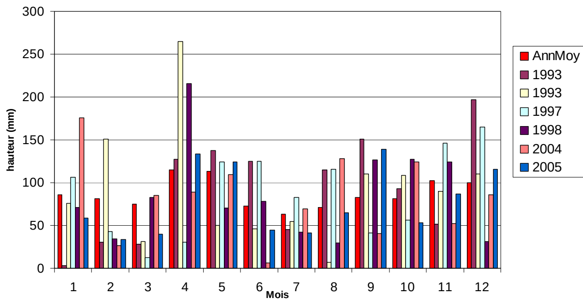
Figure 6-7 : hauteur de pluie mensuelle pour année moyenne
