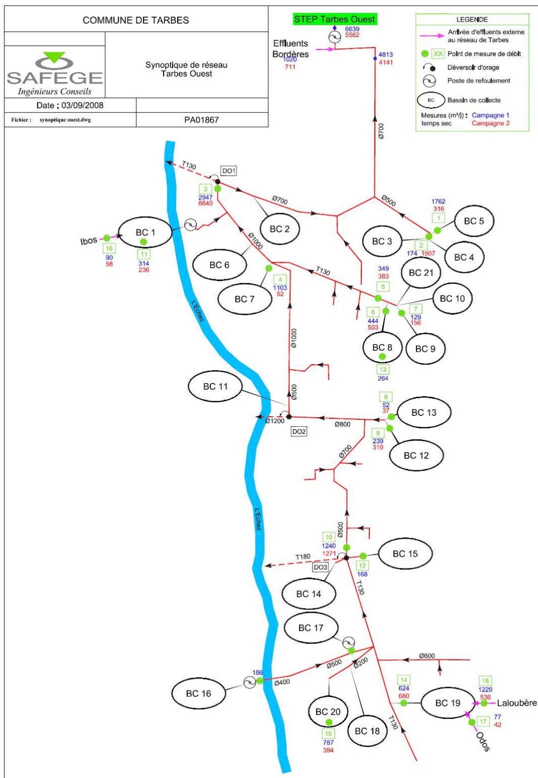
Figure 2-6 : Schématisation des bassins versants pour la construction du modèle hydraulique
