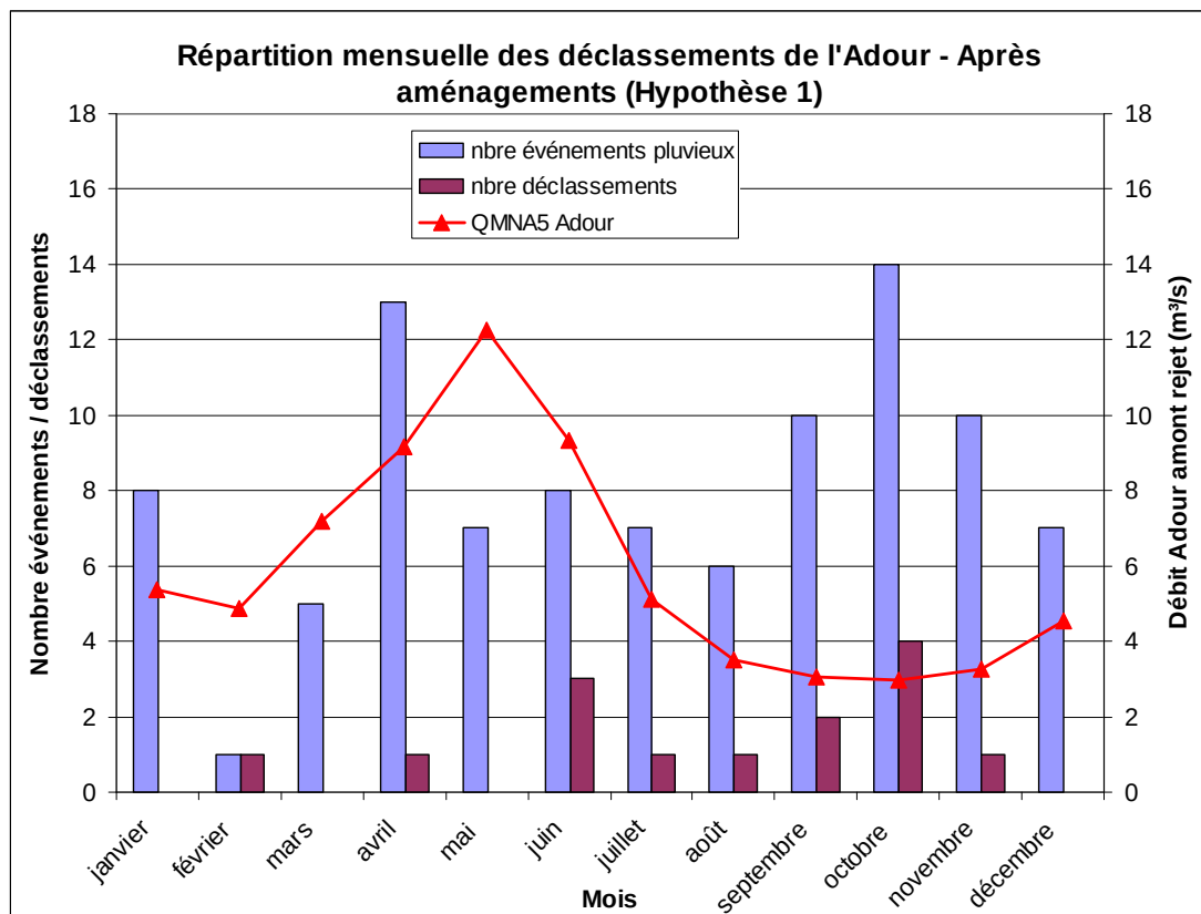
Figure 7-19 : Répartition mensuelle des déclassements de l'Adour – Rejets pluviaux – Base QMNA5
