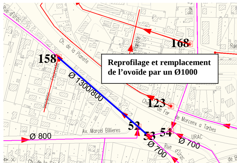
Figure 4-5 : Proposition A d'aménagement rue d'Urac
