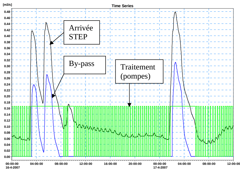
Figure 6-10 : Figure Résultats de la modélisation de l'entrée de la station de Tarbes Ouest, pluie du 16-17/04/09
