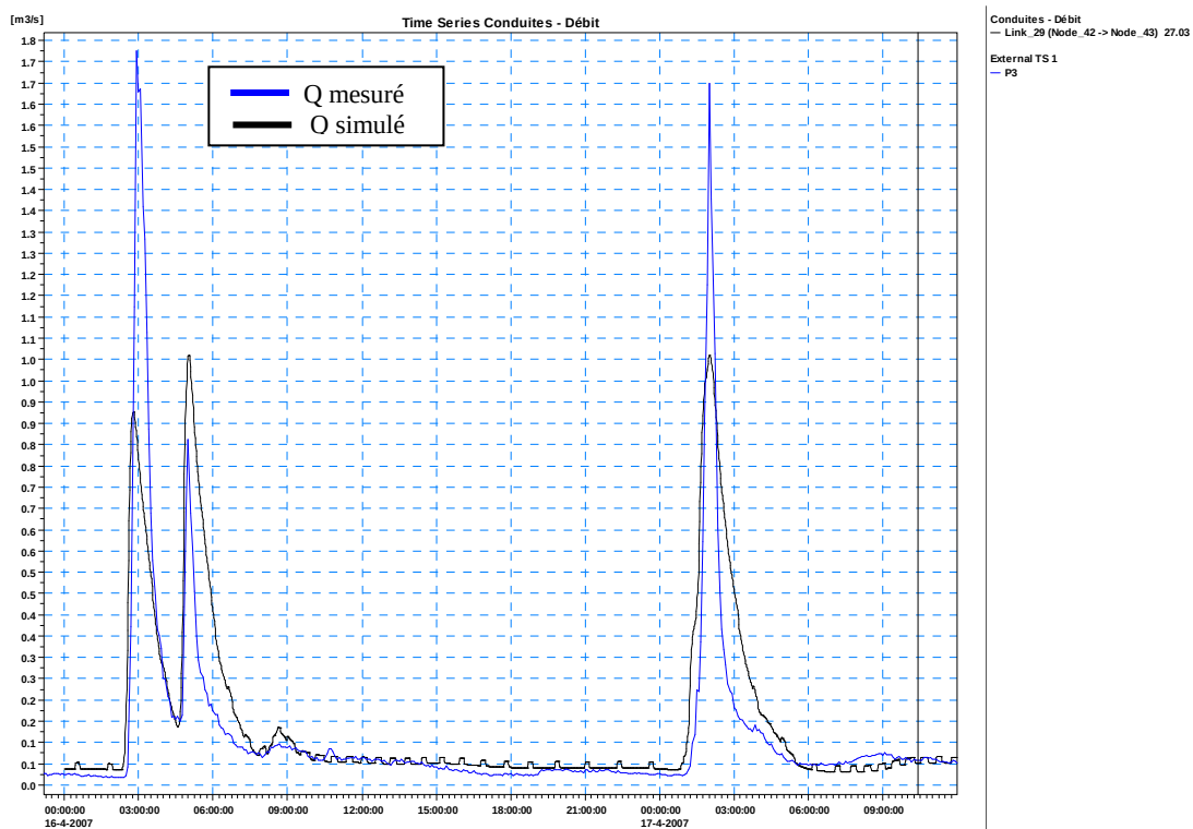
Figure 3-2 : Point P3 , débit lors de la pluie du 16-17/04/07
