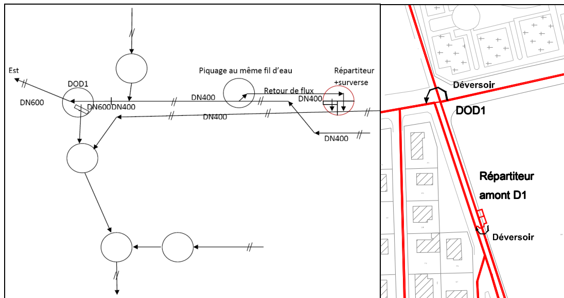
Figure 2-21 : Localisation du répartiteur amont D1
