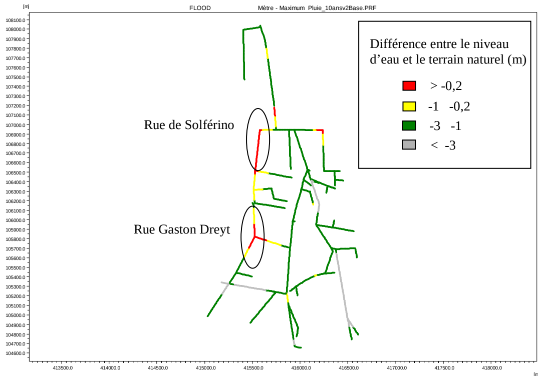
Figure 4-9 : Carte des risques de débordements du réseau pluvial - Pluie décennale
