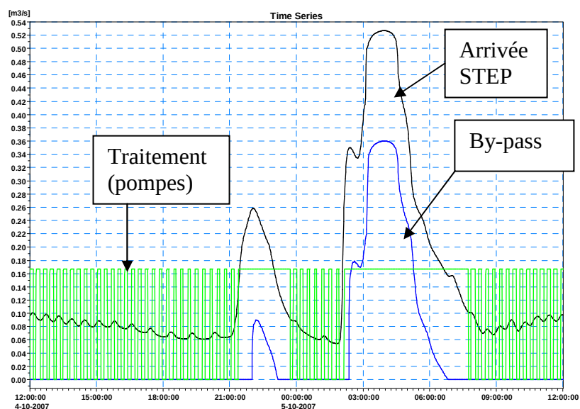
Figure 6-11 : Résultats de la modélisation de l'entrée de la station de Tarbes Ouest, pluie du 16-17/04/09
