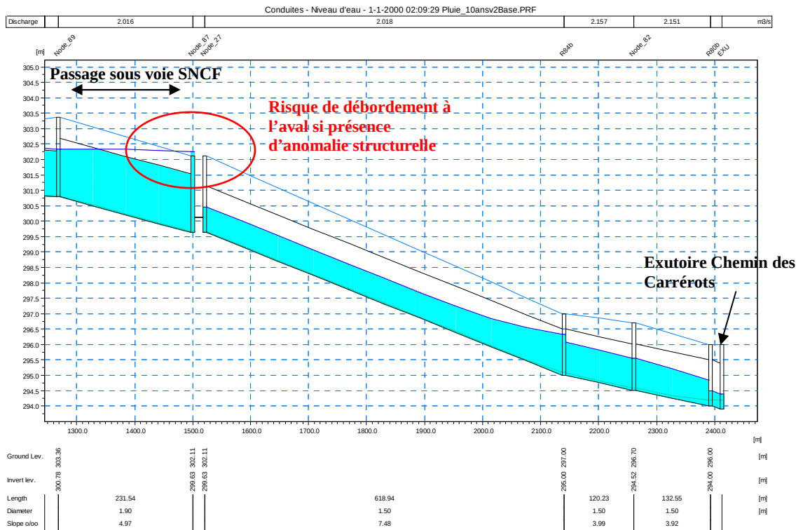
Figure 4-10 : Carte des risques de débordements du réseau pluvial - Pluie décennale
