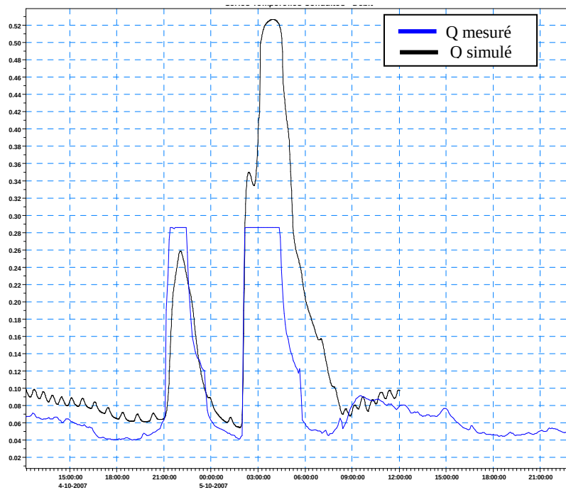
Figure 3-4 : Débit au point en entrée de station Tarbes Ouest le 10/04/2007 (plateau dans la courbe des débits correspondant à une saturation du débitmètre en entrée de station confirmée par l'exploitant)
