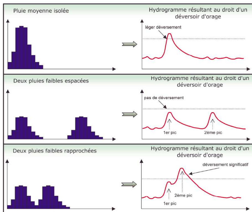
Figure 7-13 : Illustration de l'effet de pluies successives sur les déversements
