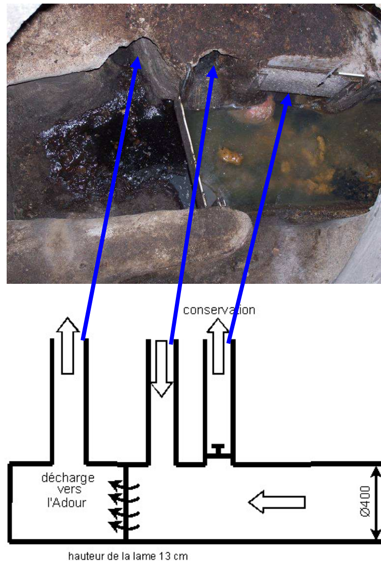
Figure 2-18 : Photographie et schéma du déversoir d'orage DOK2
