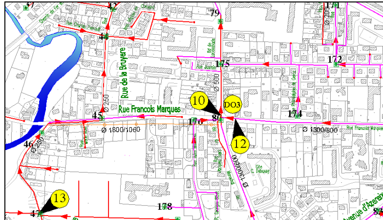
Figure 2-12 : Localisation du déversoir d'orage DO3
