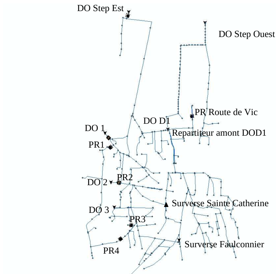
Figure 2-7 : Localisation des ouvrages modélisés (hors Adour Alaric)
