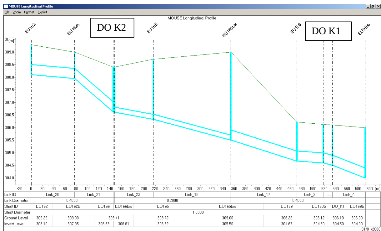
Figure 5-2 : Profil 1 : DN400 de l'avenue de la Marne à l'exutoire
