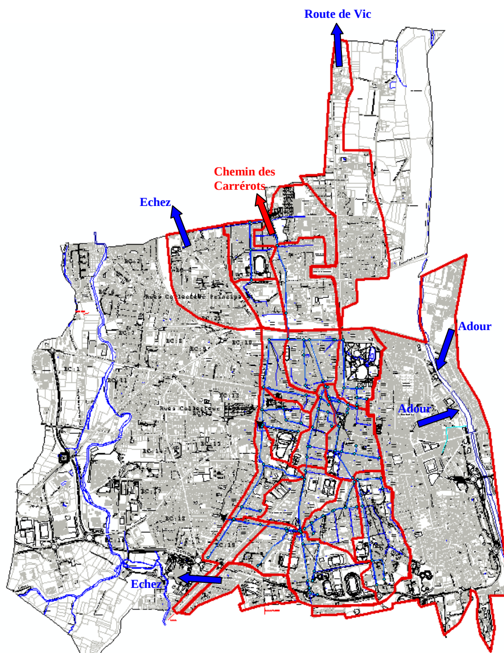
Figure 2-35 : Bassins versants et exutoires pluviaux (vue en plan MIKE URBAN)
