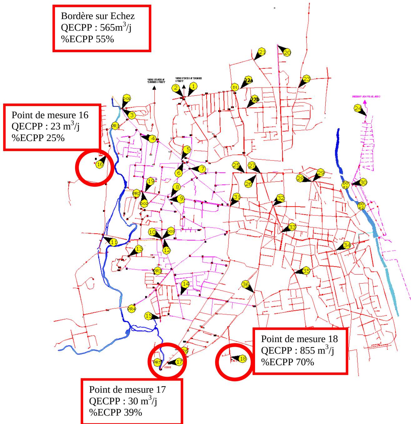
Figure 10-2 : Localisation entrées d'eaux claires parasites en provenance des communes voisines
