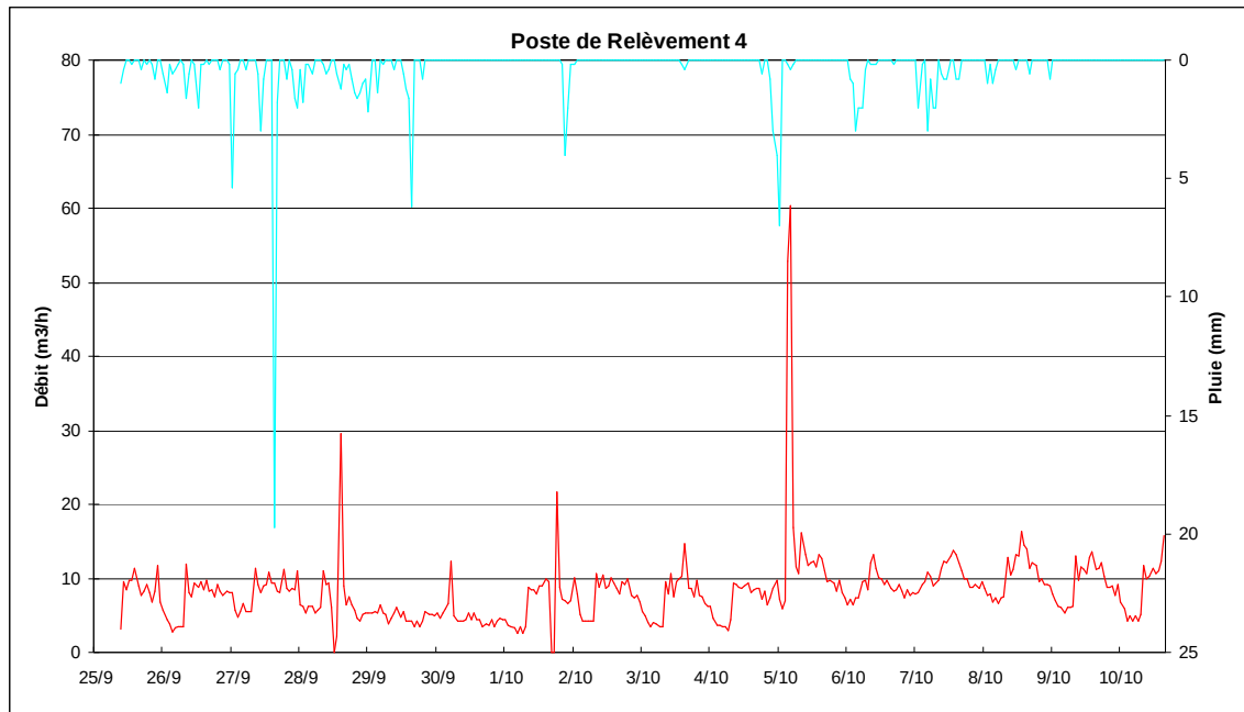
Figure 2-30 : Fonctionnement du poste PR4 du 25/09 au 10/10/2007
