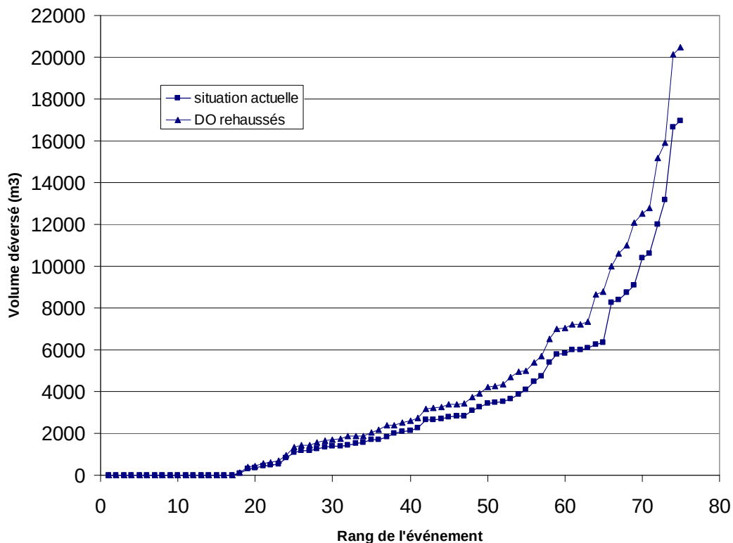
Figure 7-3 : Effets de l'augmentation du niveau des seuils des déversoirs sur les volumes déversés par événement pluvieux au by pass de la station d'épuration
