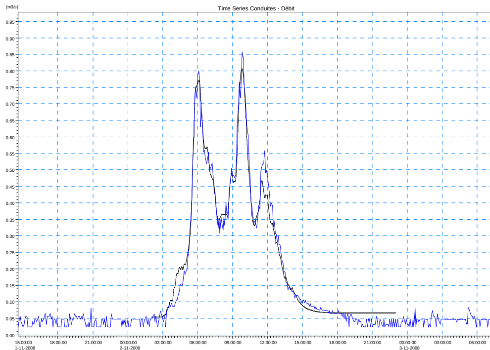
Figure 3-10 : Courbe de calage – Point P6 – pluie du 2/11/08
