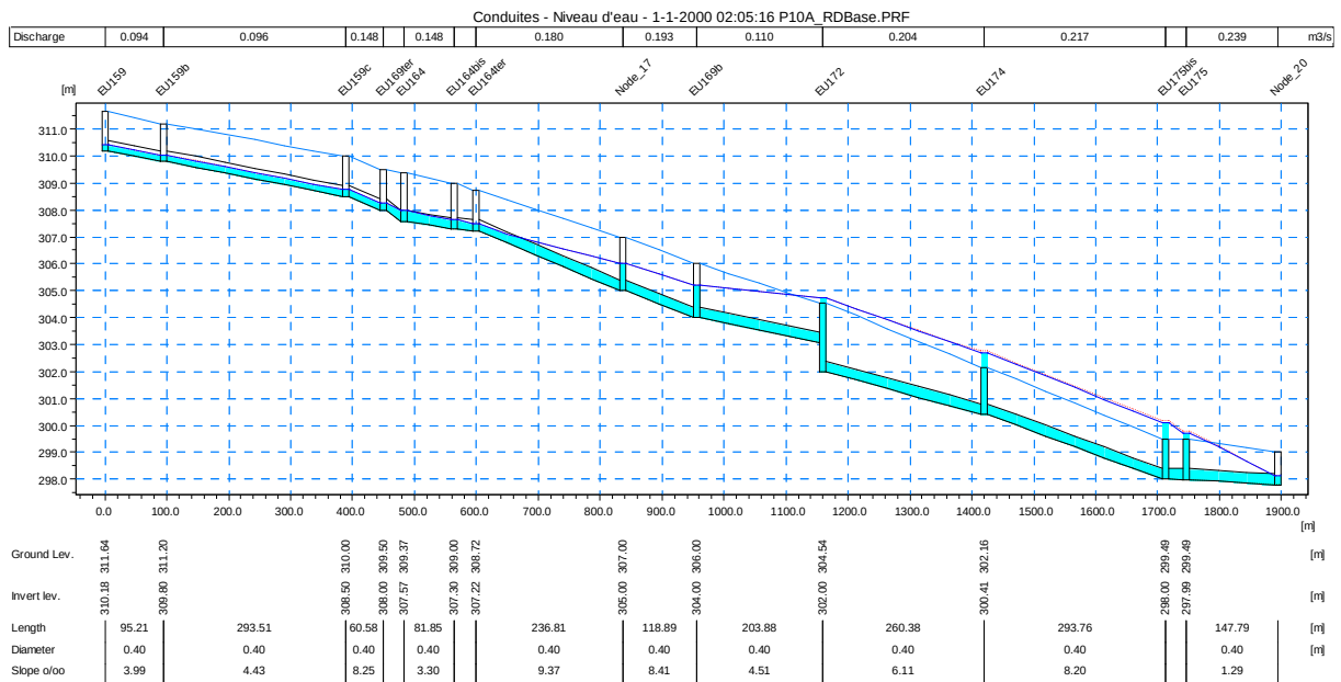
Figure 5-2 : Ligne d'eau EU162 au passage sous la SNCF pour la pluie de période de retour 10 ans
