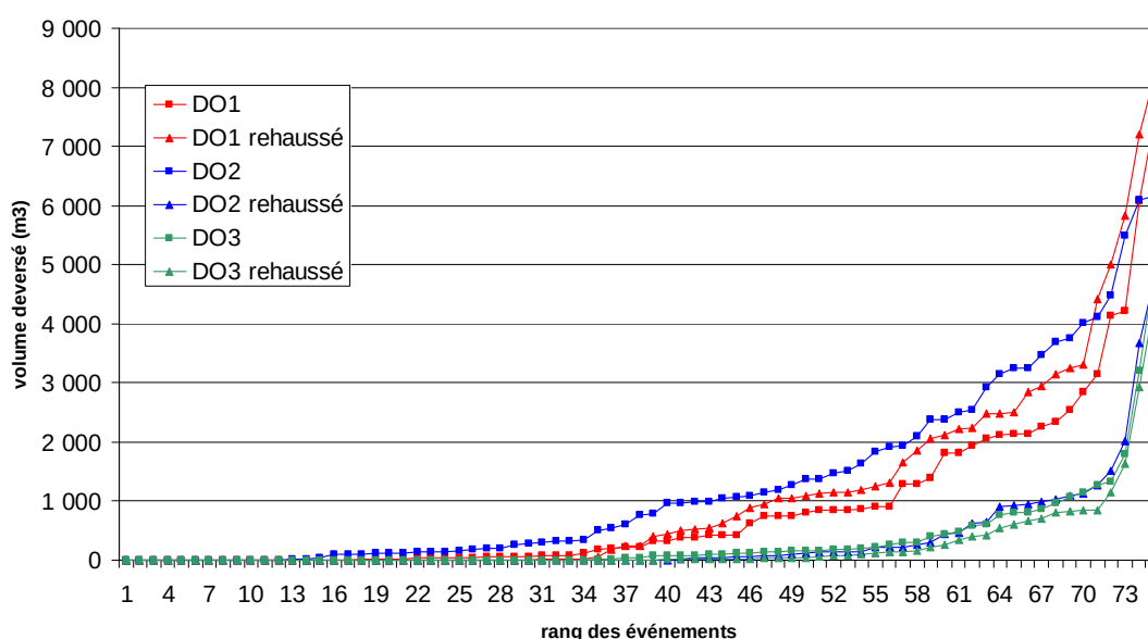
Figure 7-2 : Effets de l'augmentation du niveau des seuils des déversoirs sur les volumes déversés par événement pluvieux
