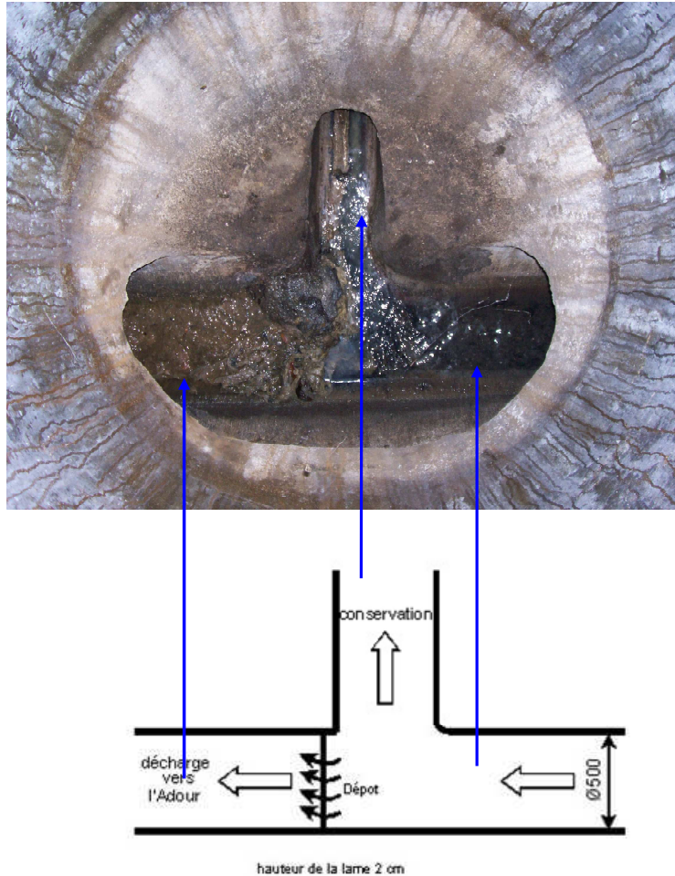
Figure 2-16 : Photographie et schéma du déversoir d'orage DOK1
