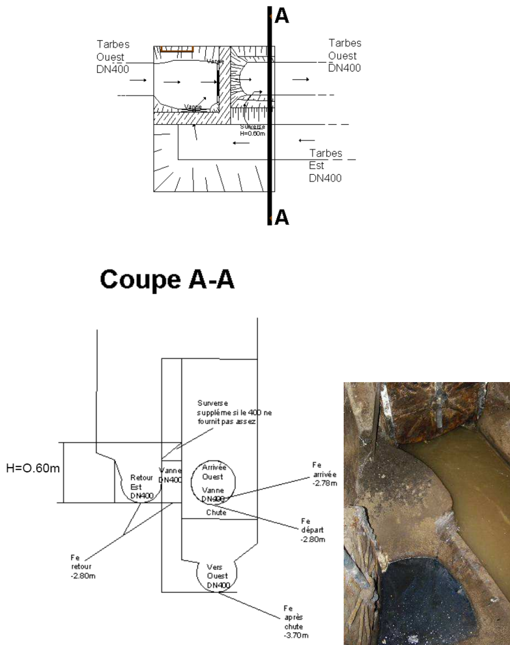
Figure 2-22 : Plans du répartiteur amont D1
