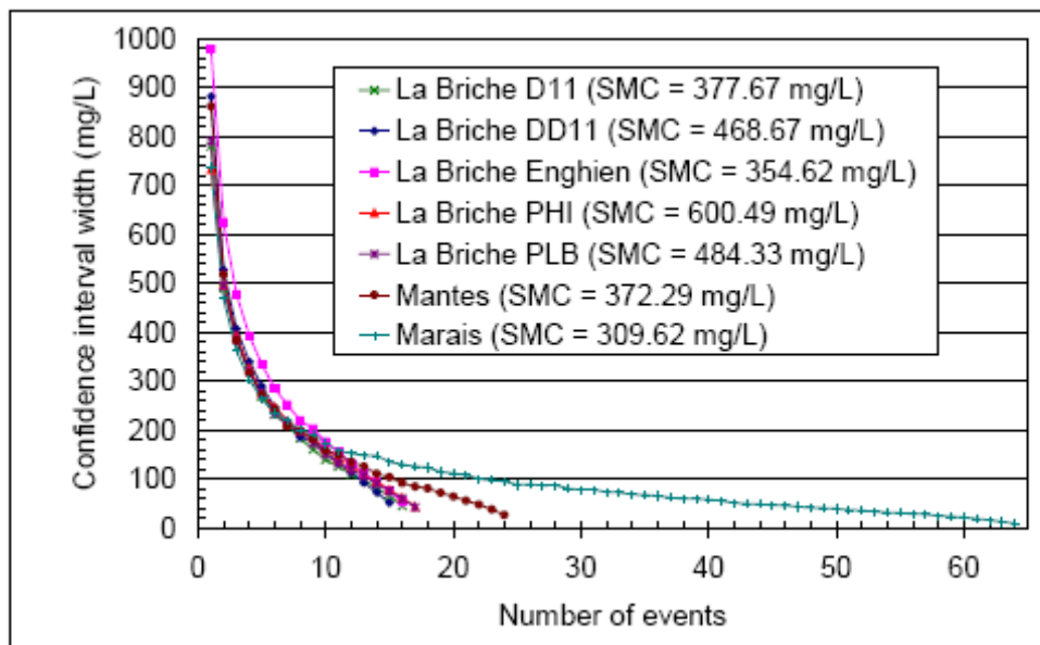
Figure 7-9 : Incertitude sur les concentrations moyennes en fonction du nombre d'événements sur 7 réseaux unitaires. Extrait de : Uncertainty in site mean pollutant concentration according to the number of measured events, Chebbo, Novatech 2004
