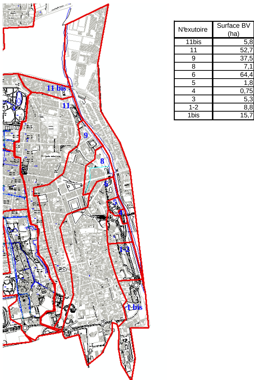
Figure 7-15 : Découpage des BV Adour rive gauche
