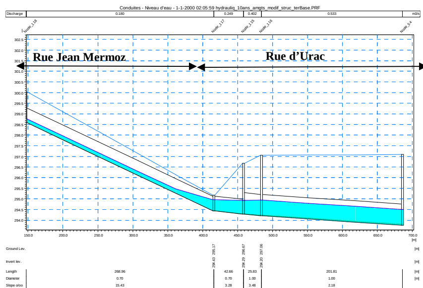
Figure 4-6 : Ligne d'eau suite à la simulation de l'aménagement A rue d'Urac
