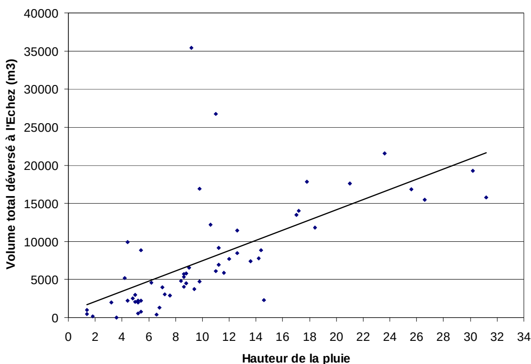
Figure 7-12 : Volumes déversés à l'Echez par le réseau unitaire et hauteurs des pluies correspondantes pour l'année 1998
