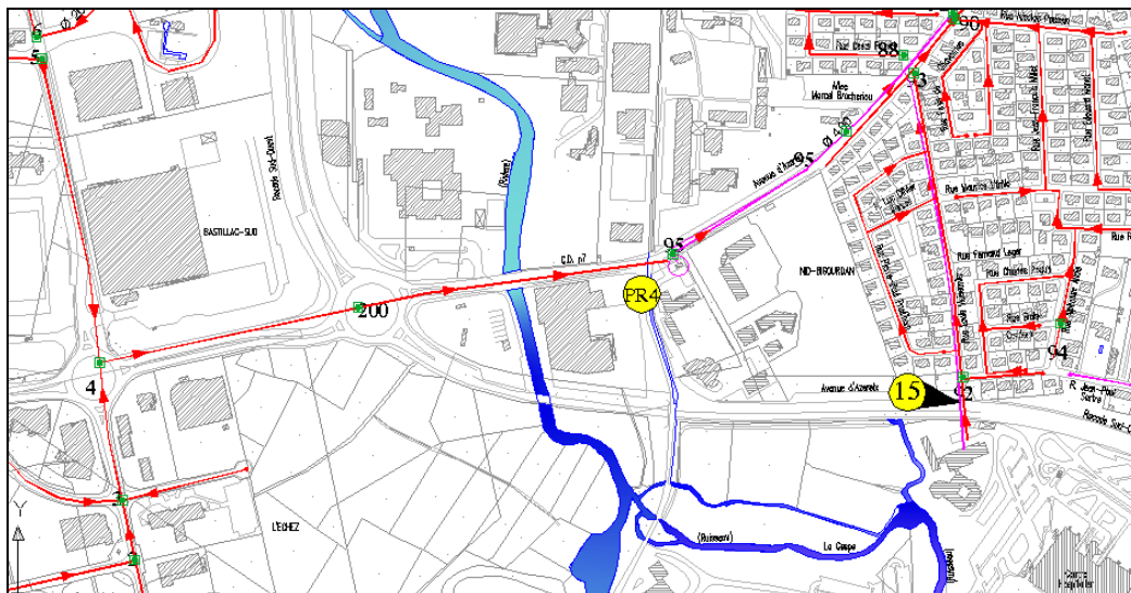
Figure 2-29 : Localisation du poste de relèvement PR4
