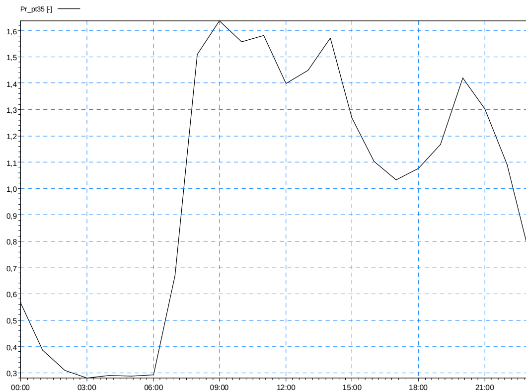
Figure 2-34 : Exemple de profil de temps sec : débit du BV P, déduit du point de mesures
