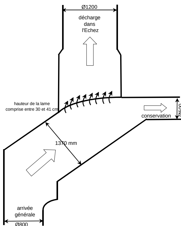
Figure 2-11 : Photographie et schéma du déversoir d'orage DO2
