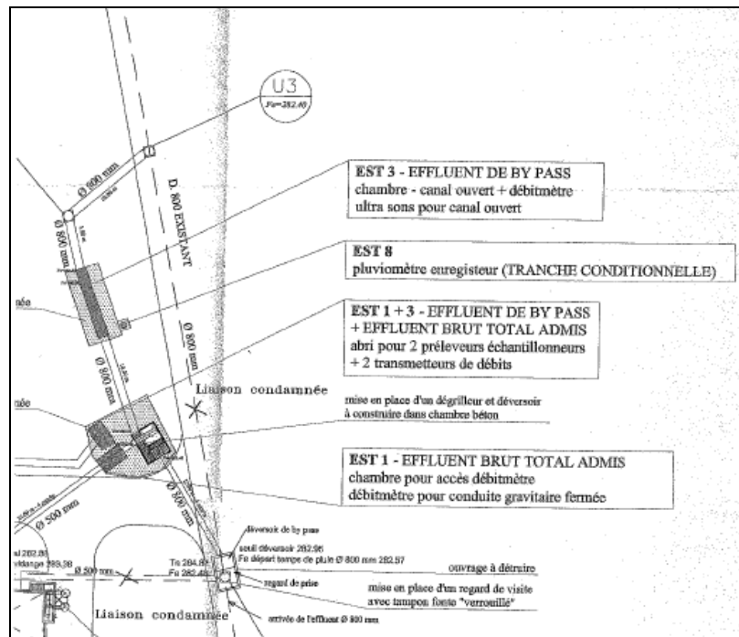
Figure 2-15 : Plan descriptif des ouvrages à l'entrée de la STEP de Tarbes Est
