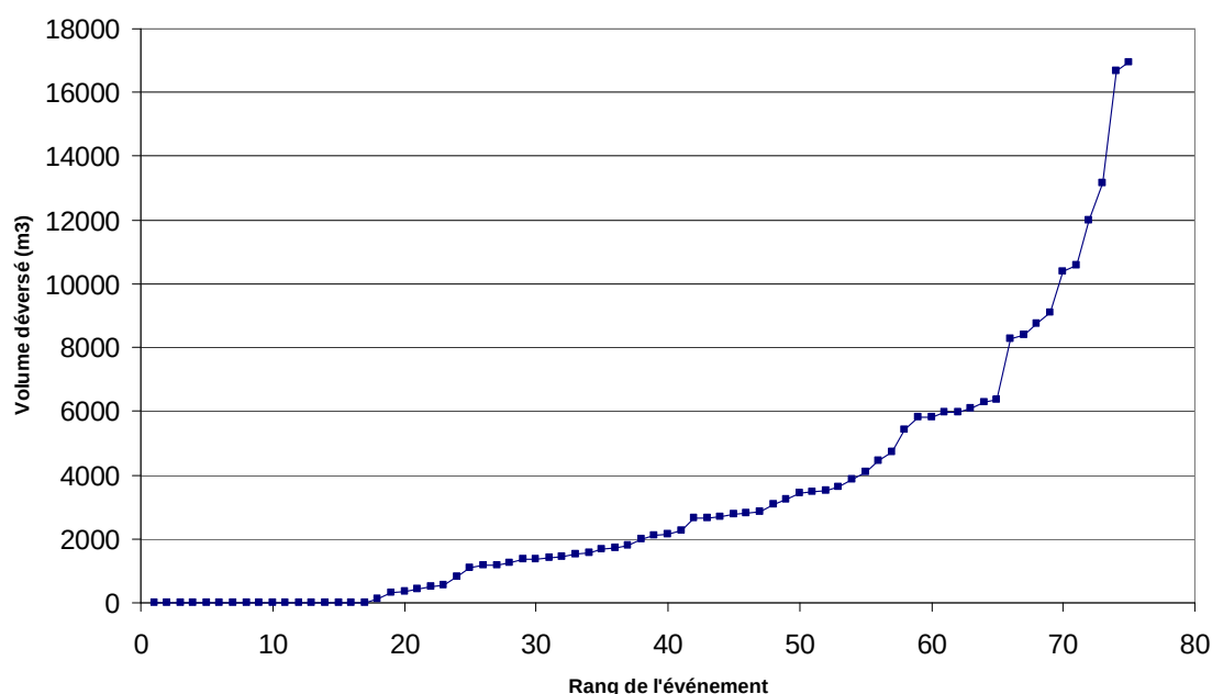
Figure 6-9 : Volume rejeté par le by pass de la station d'épuration de Tarbes Ouest selon le nombre d'événements pluvieux
