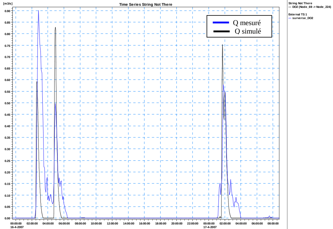
Figure 3-3 : Point DO2, débit lors de la pluie du 16-17/04/07
