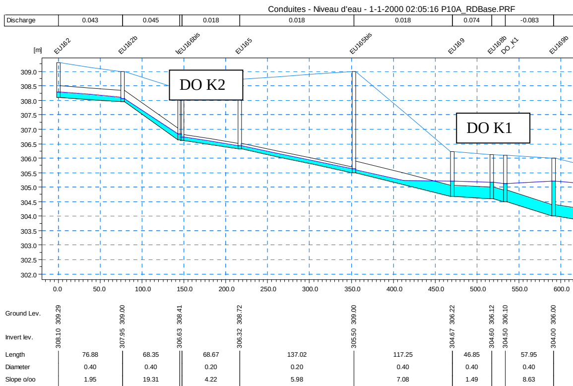
Figure 5-2 : Ligne d'eau de l'avenue de la Marne à l'exutoire pour la pluie de période de retour 10 ans
