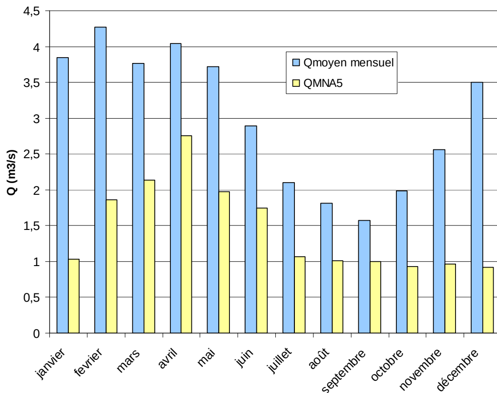
Figure 7-8 : Débits de l'Adour à Tarbes (source banque hydro)
