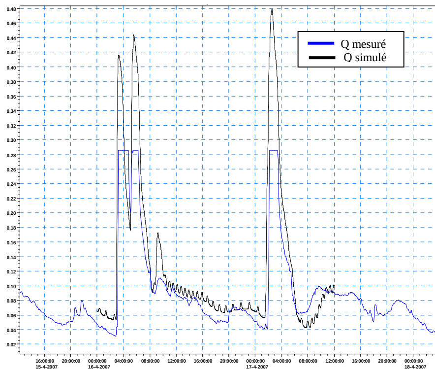
Figure 3-5 : Débit au point en entrée de station Tarbes Ouest le 16-17/04/200
