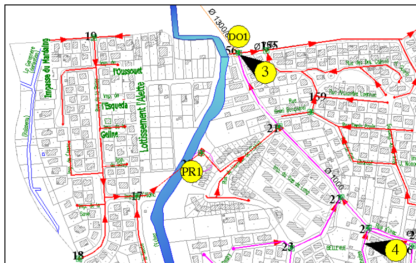
Figure 2-25 : Localisation du poste de relèvement PR1
