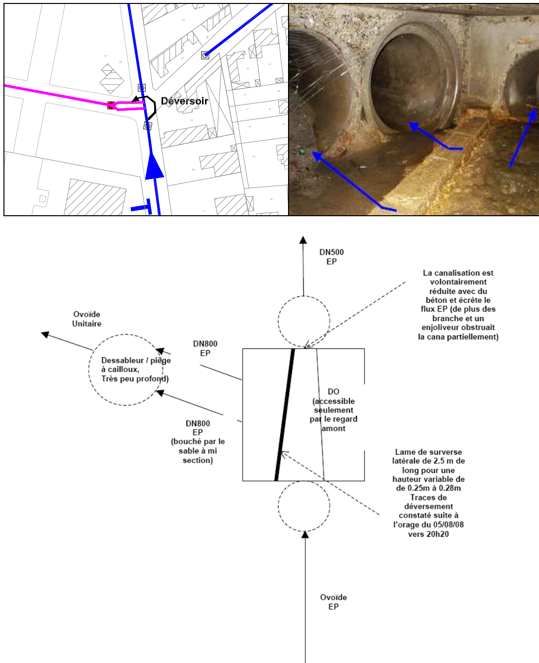
Figure 2-23 : Localisation de la surverse place du général Faulconnier
