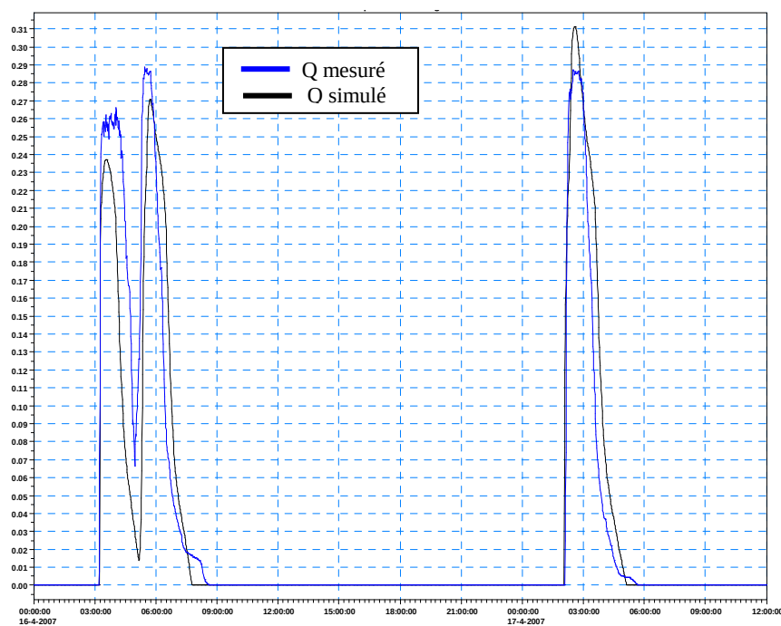
Figure 3-6 : Débits déversés par le by pass de la station de Tarbes ouest le 16-17/04/07
