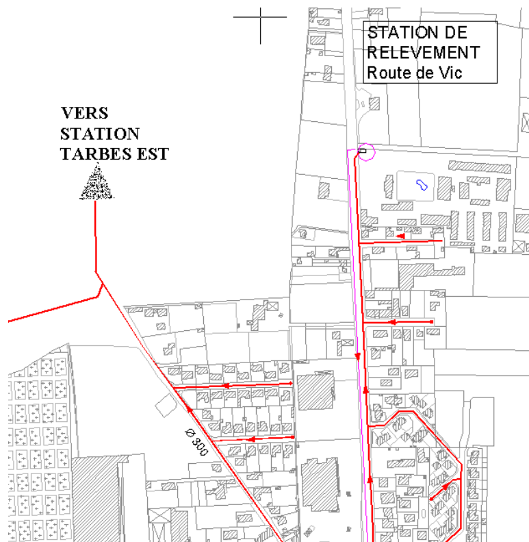
Figure 2-32 : Localisation du PR Route de Vic
