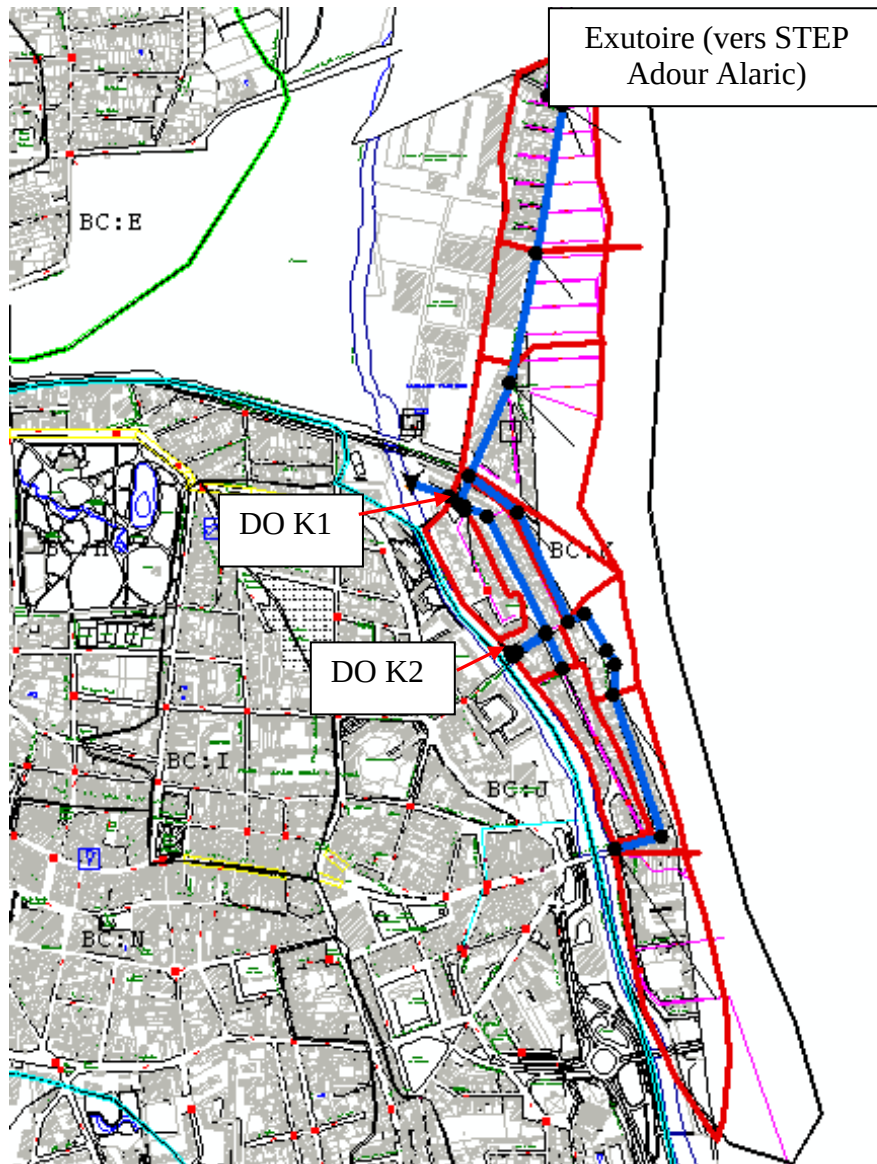
Figure 5-1 : Vue en plan du réseau modélisé (réseau + BV)
