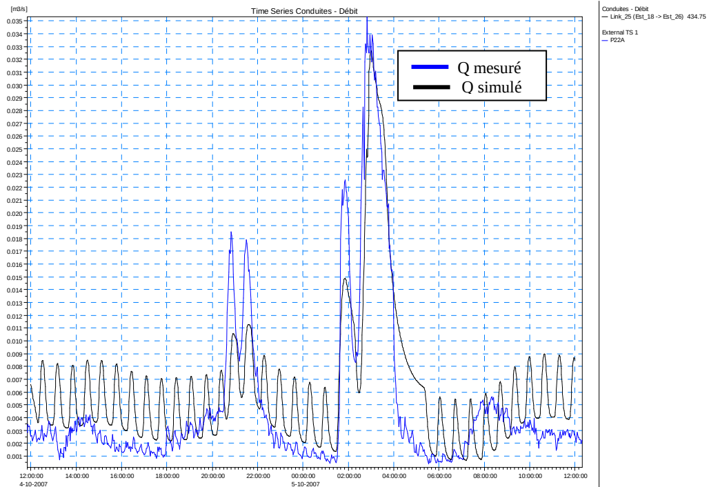
Figure 3-7 : Débit au point P22A le 10/04/2007
