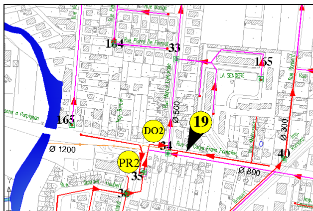
Figure 2-10 : Localisation du déversoir d'orage DO2
