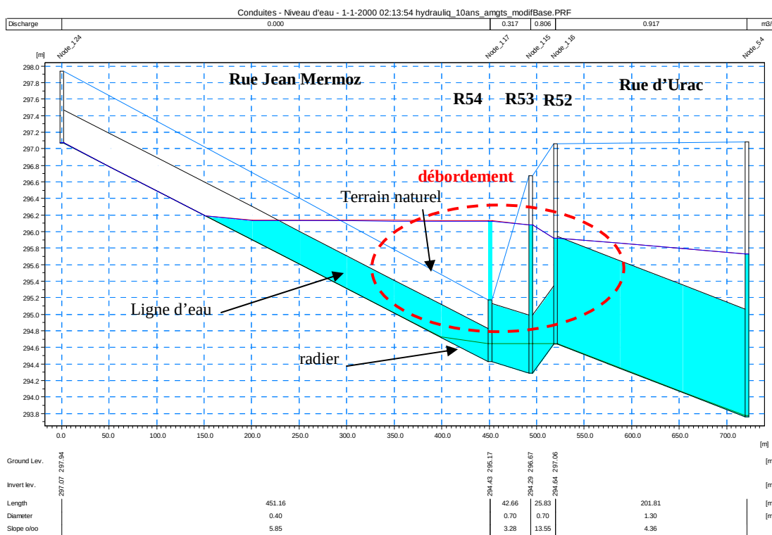
Figure 4-4 : Ligne d'eau rue d'Urac pour la pluie décennale
