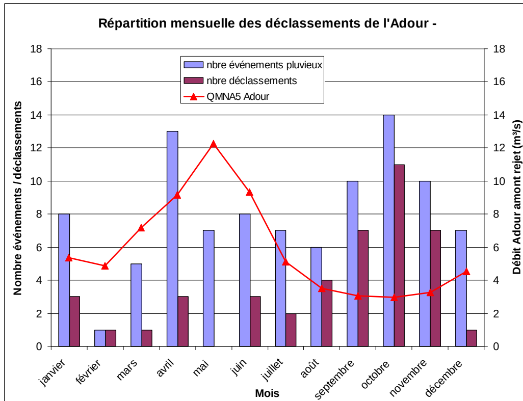
Figure 7-17 : Répartition mensuelle des déclassements de l'Adour – Rejets pluviaux – Base QMNA5
