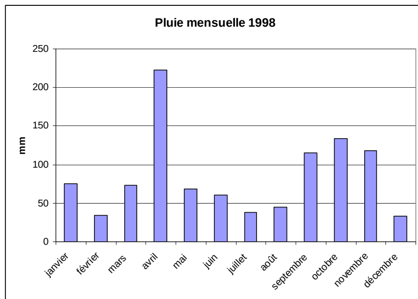
Figure 7-14 : Hauteurs de pluie mensuelles pour le calcul des déclassements de l'Adour
