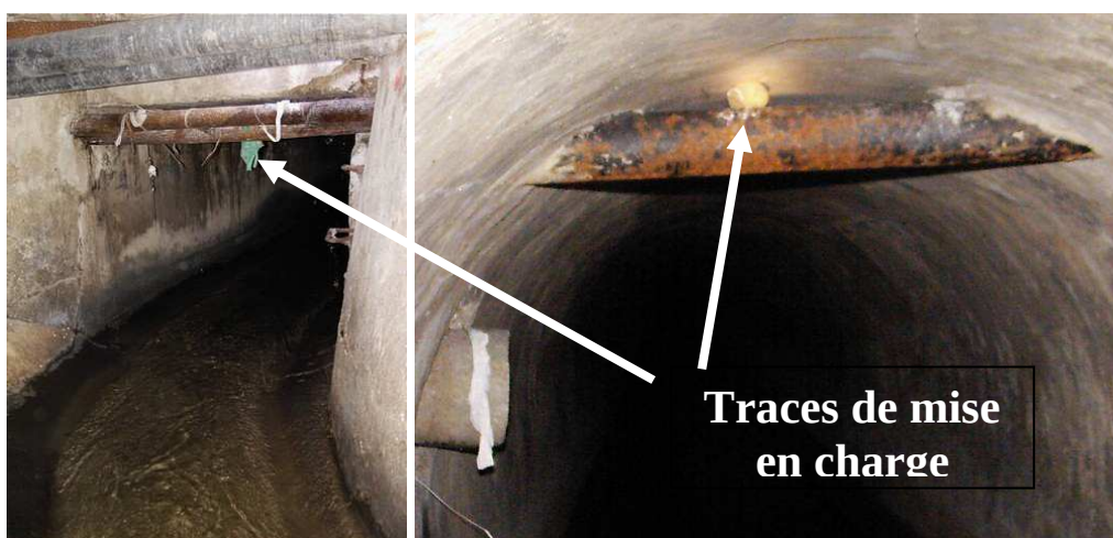
Figure 4-11 : Illustration de la mise en charge dans l'ovoïde à l'amont de la traversée de la voie SNCF
