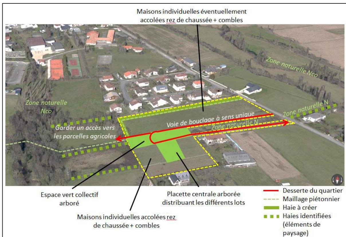
Figure 18 – Principe des aménagements projetés - Rue du Bois
