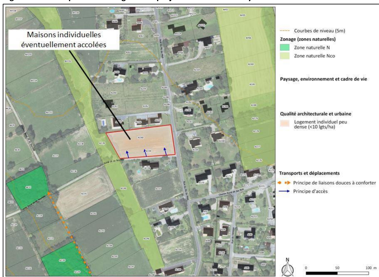
Figure 20 – Principe des aménagements projetés - Chemin de Beyrède
