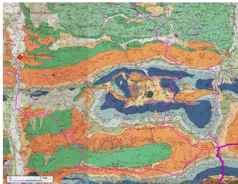
A TITRE ILLUSTRATIF, EXTRAIT DE LA CARTE GEOLOGIQUE DU BRGM CONCERNANT LE TERRITOIRE DE LOUVIE-JUZON
