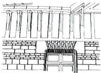
Débords de toit en bois protégeant une partie de mur enduit en ciment avec des faux pans de bois et des jambettes peints. Ouverture sur une façade en moellon calcaire équarri, soulignée par des modénatures en brique et fermée par des volets persiennés métalliques
