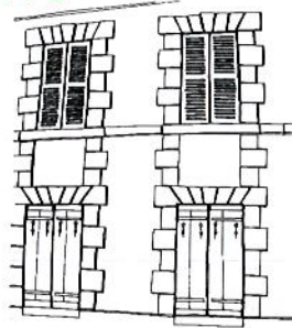
A l'étage, volets en bois persiennés en totalité, au rez-de-chaussée, volets en bois plein avec jour de ventilation
