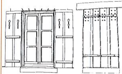
Volets en bois plein constitués de lames verticales assemblées par des barres horizontales métalliques ou en bois, avec des jours de ventilation
