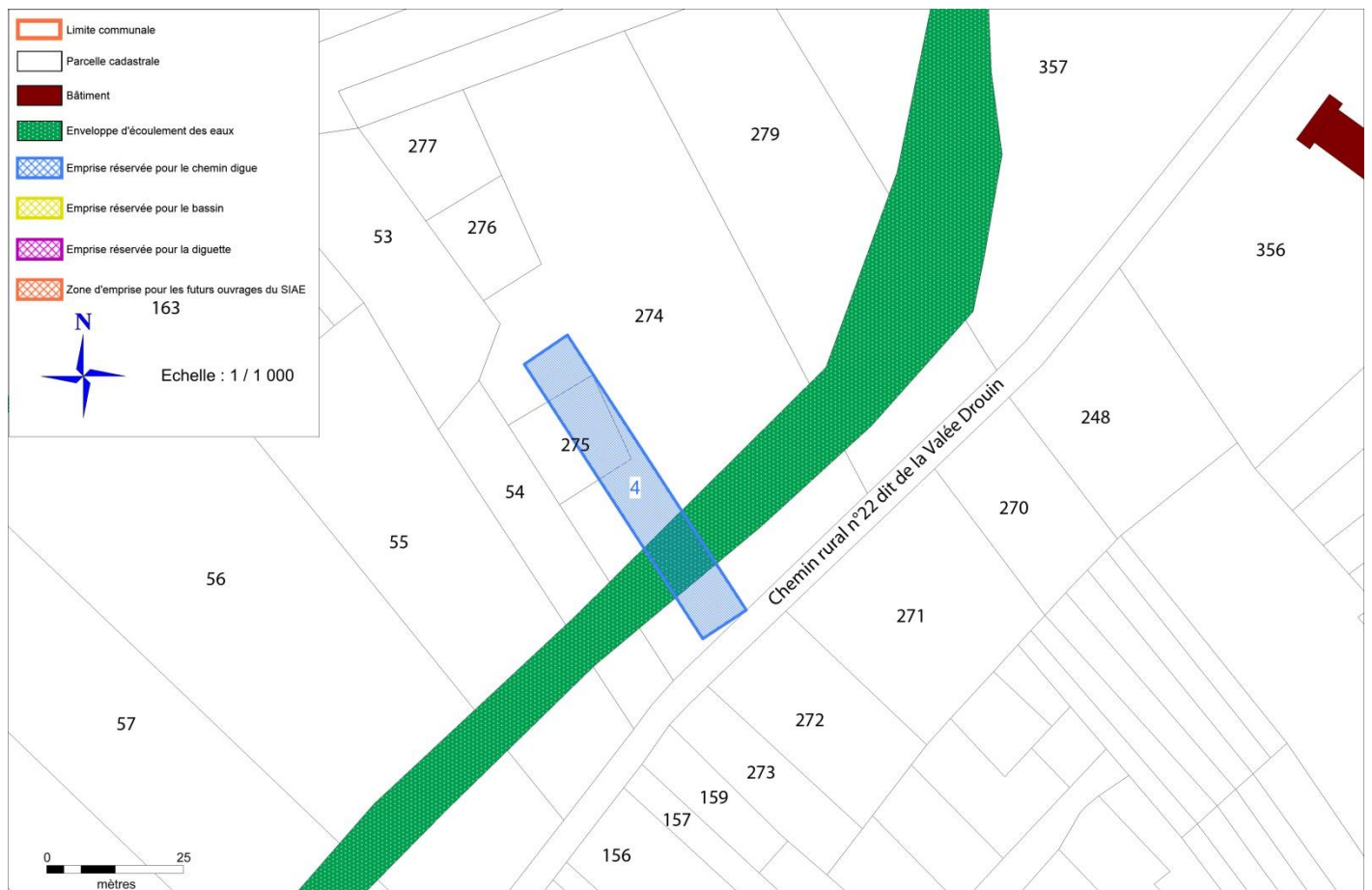
Figure 10 : Emplacement réservé : Chemin Digue n°4, parcelles n° 274 et 275
