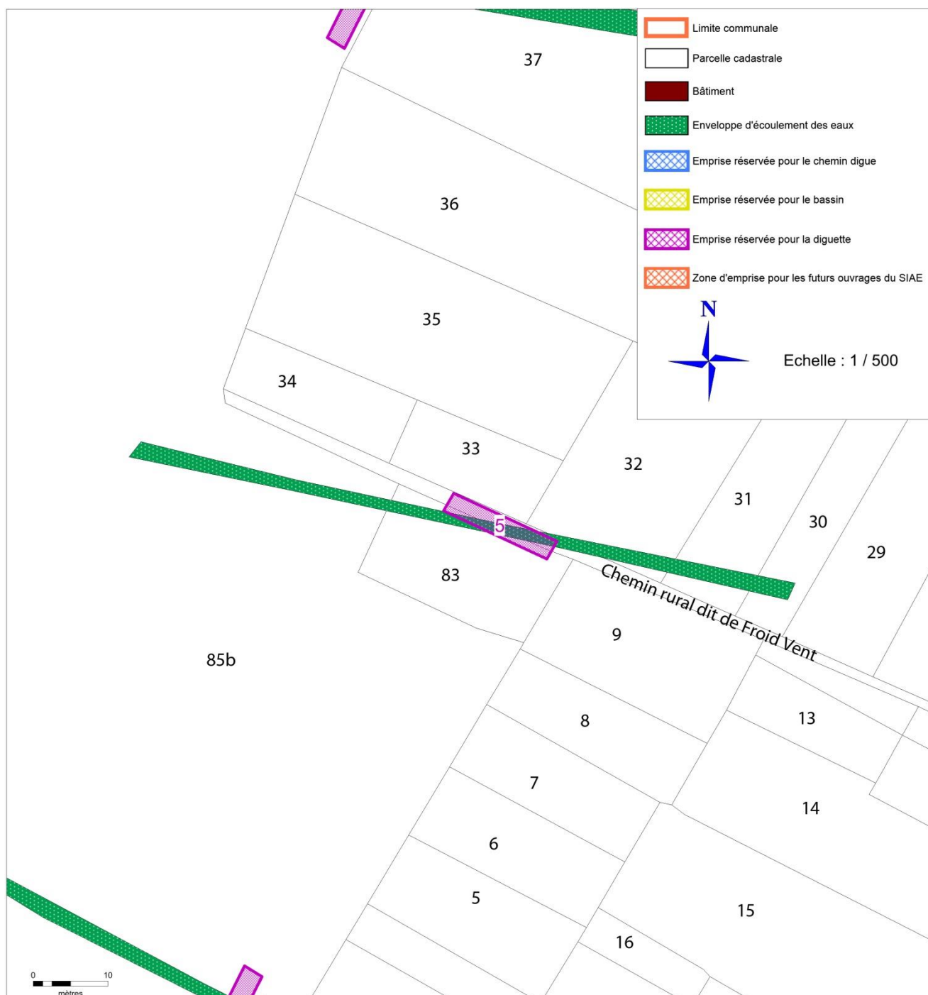
Figure 18 : Emplacement réservé : Diguette n°5, parcelle n°83
