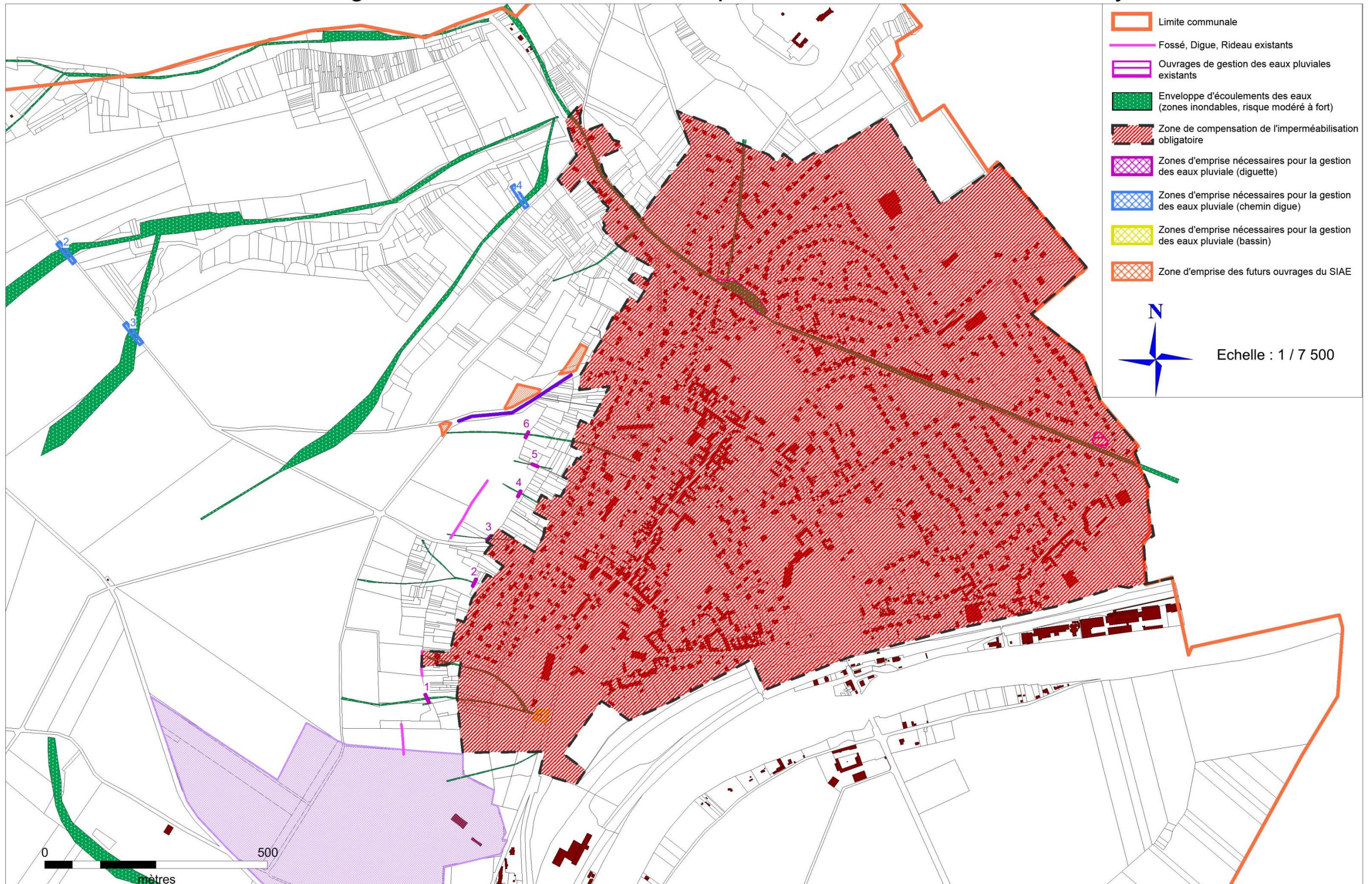
Carte 2 du zonage d'assainissement des eaux pluviales de la commune de Précy-sur-Oise
