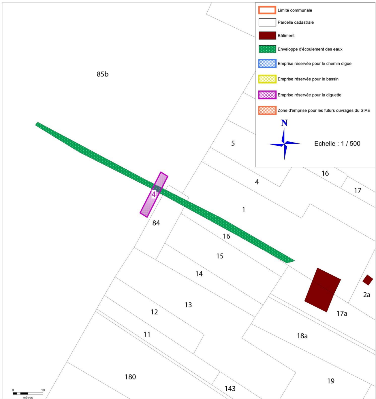
Figure 17 : Emplacement réservé : Digue n°4, parcelle n°85 b
