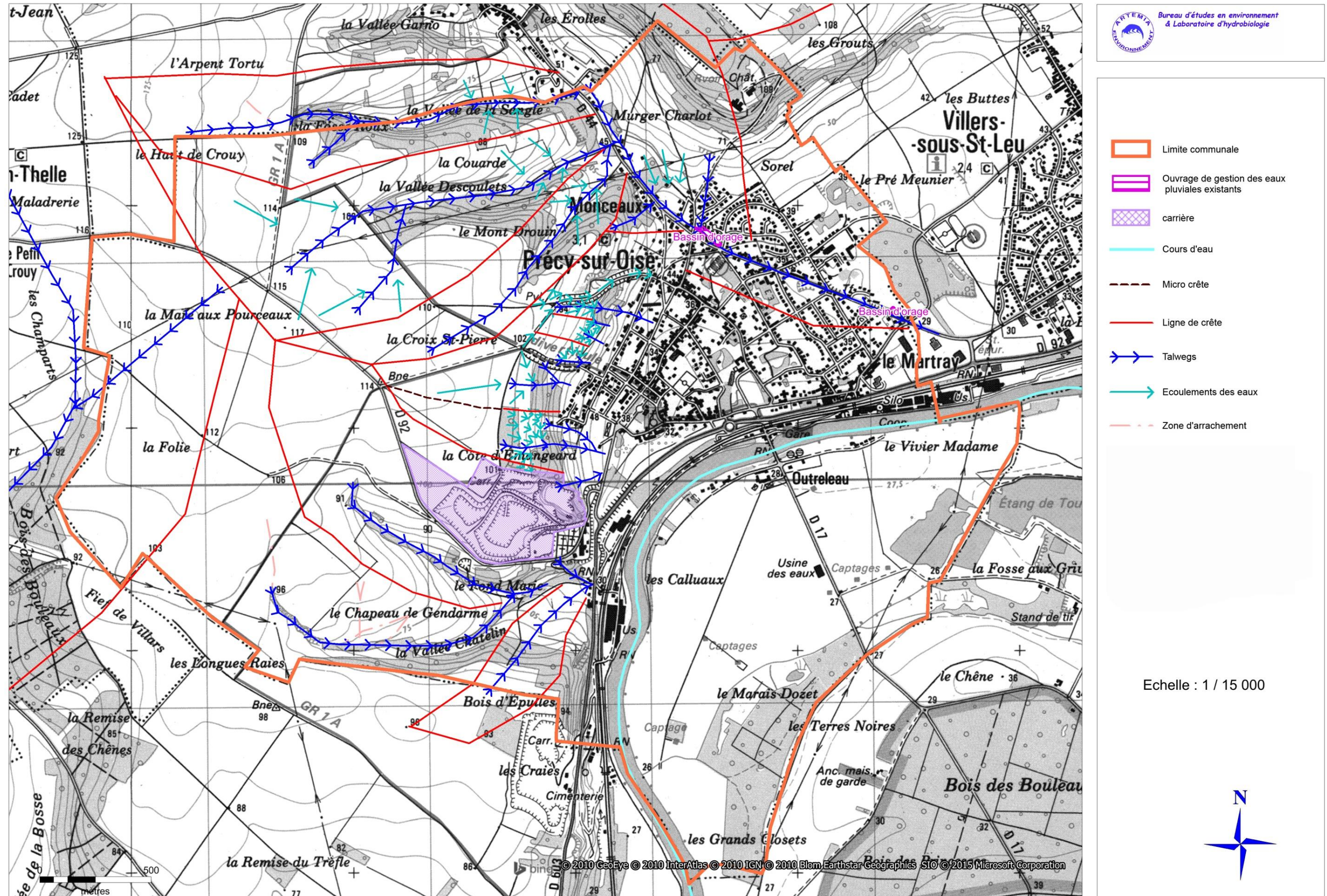
Figure 3 : Ecoulements des eaux pluviales au niveau des bassins versants agricoles
