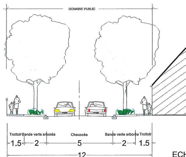
Coupe de principe AA' (à adapter suivant les contraintes du terrain)
