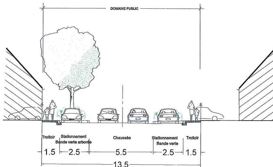
Coupe de principe AA'
