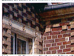
Linéau métallique, modénature en brique silico-calcaire et brique anglie
