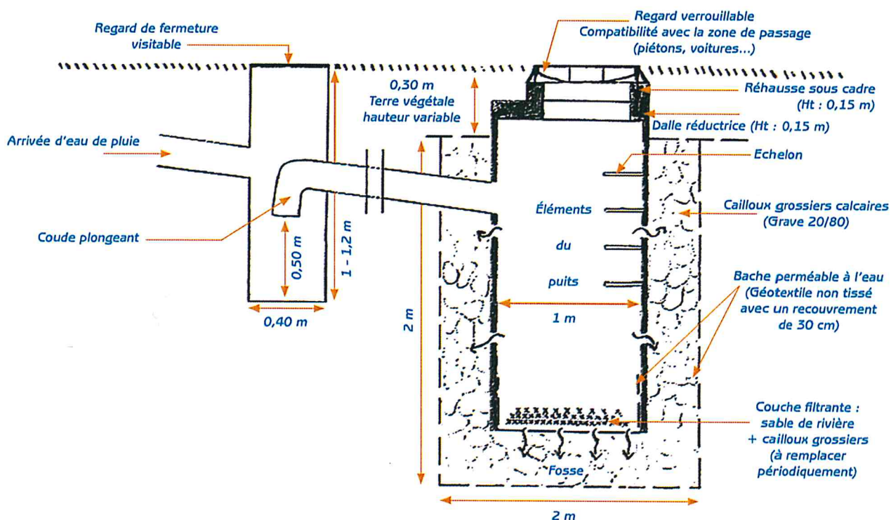
PUITS D'INFILTRATION
