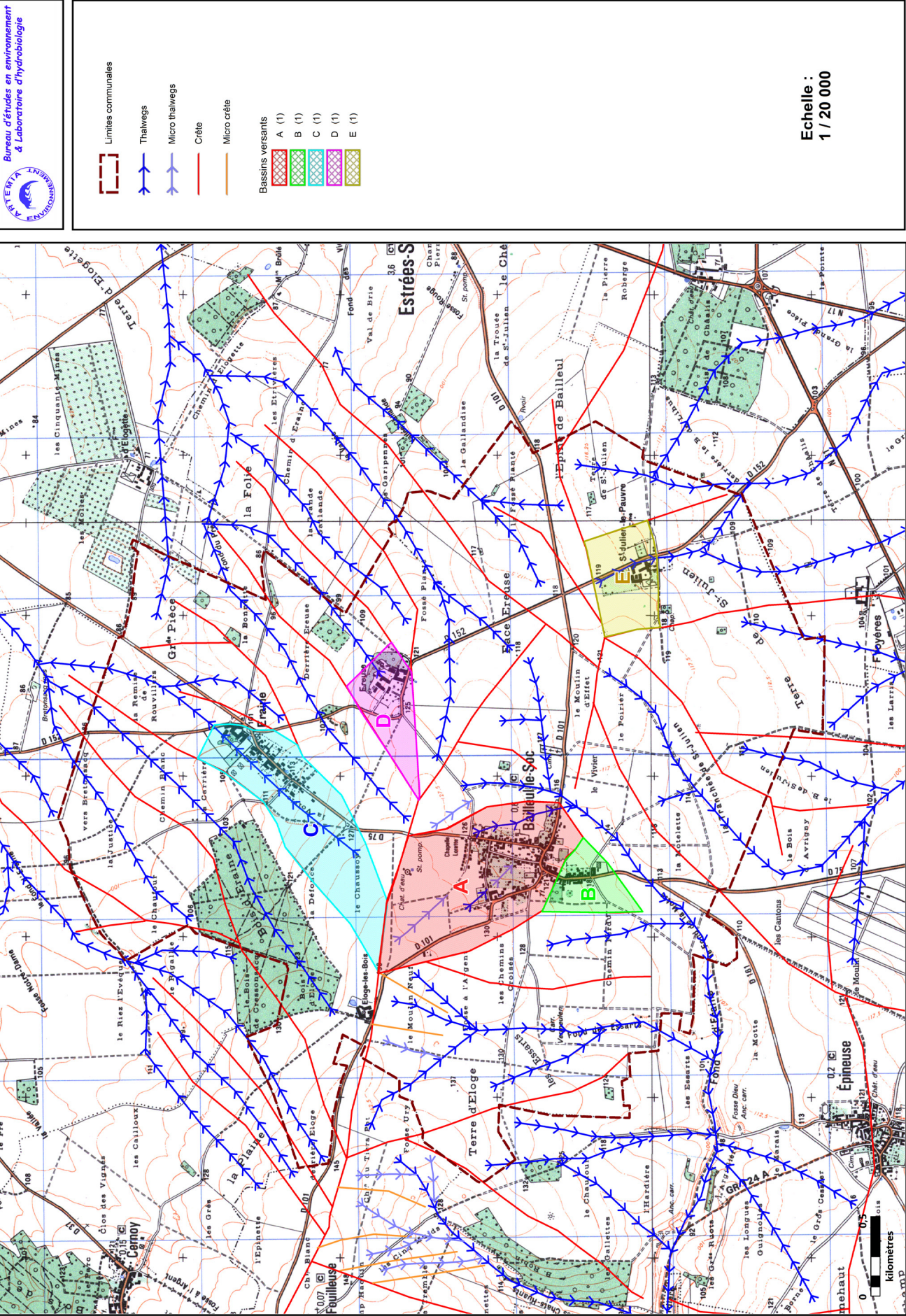
Figure 9 : Carte des bassins versants de la commune de Bailleul-Le-Soc
