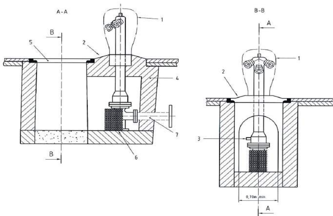
schéma 5 socle de propreté pour PI à plusieurs demi-raccords
