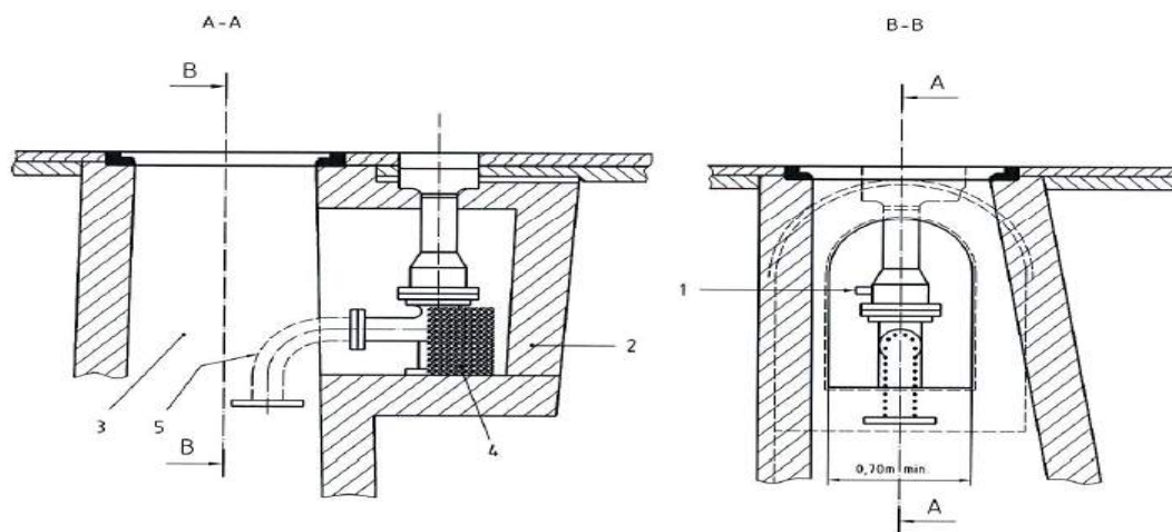
schéma 3 installation d'une BI accolée à un regard de vidange
