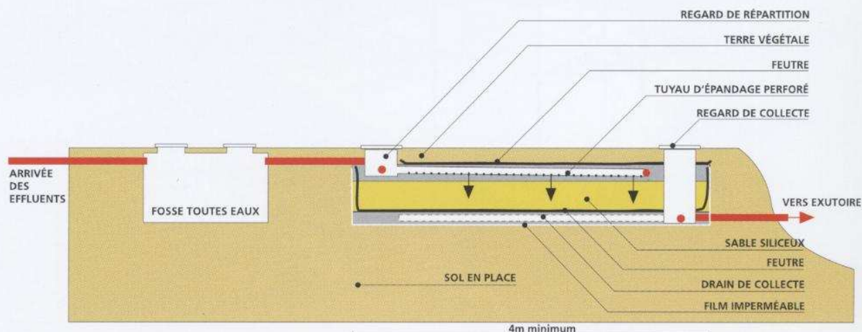
COUPE LONGITUDINALE
