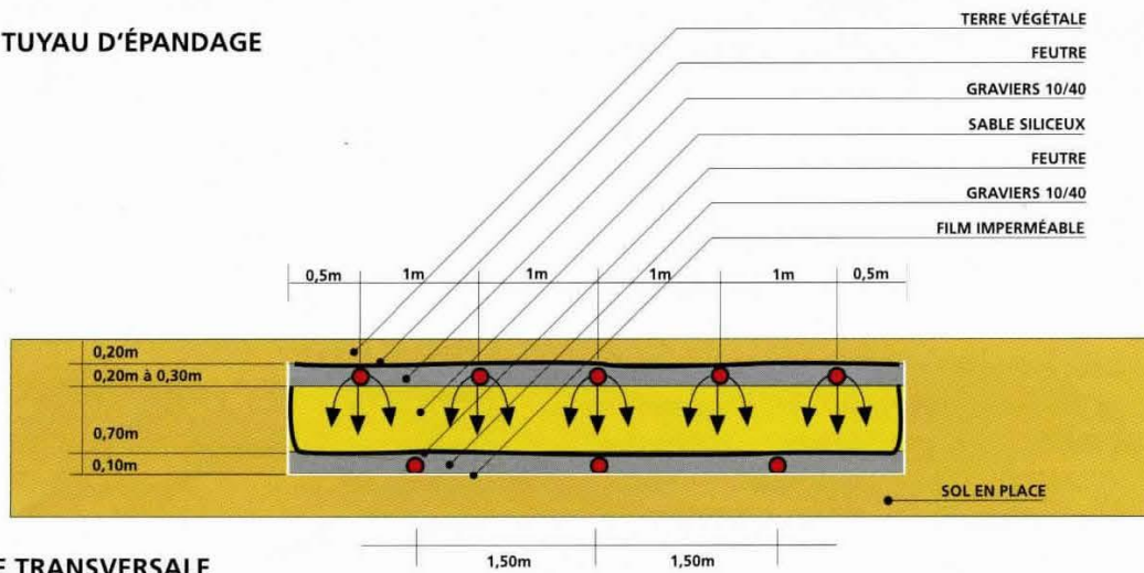
COUPE TRANSVERSALE
