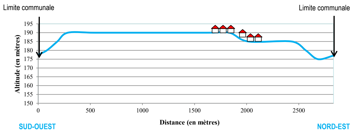
Coupe topographique n°1
