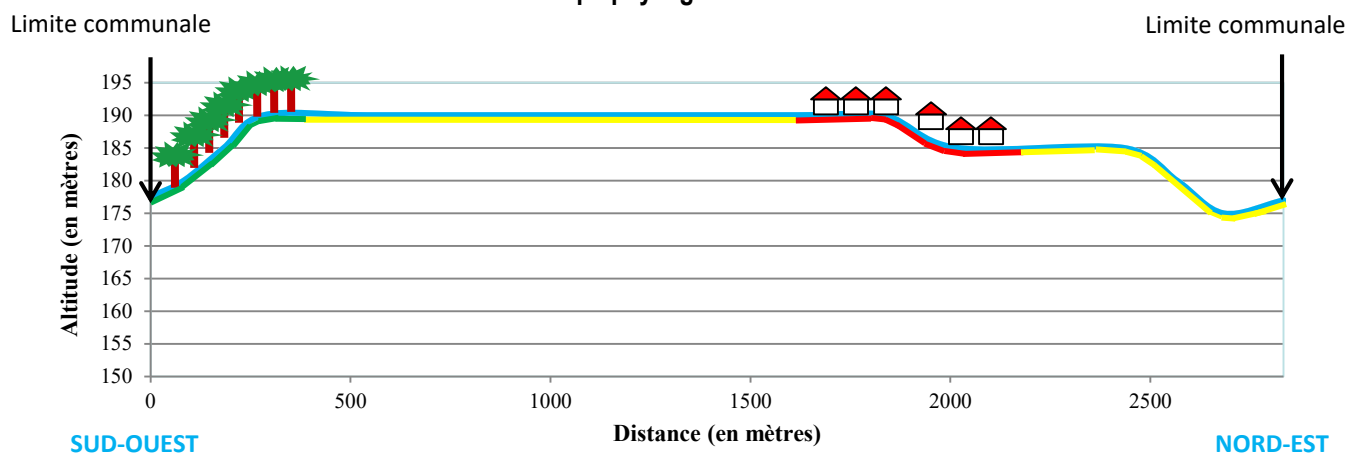
Coupe paysagère n°1
