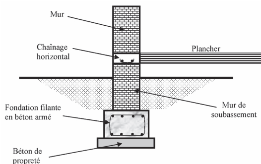
Figure 9 Fondation filante en béton armé
