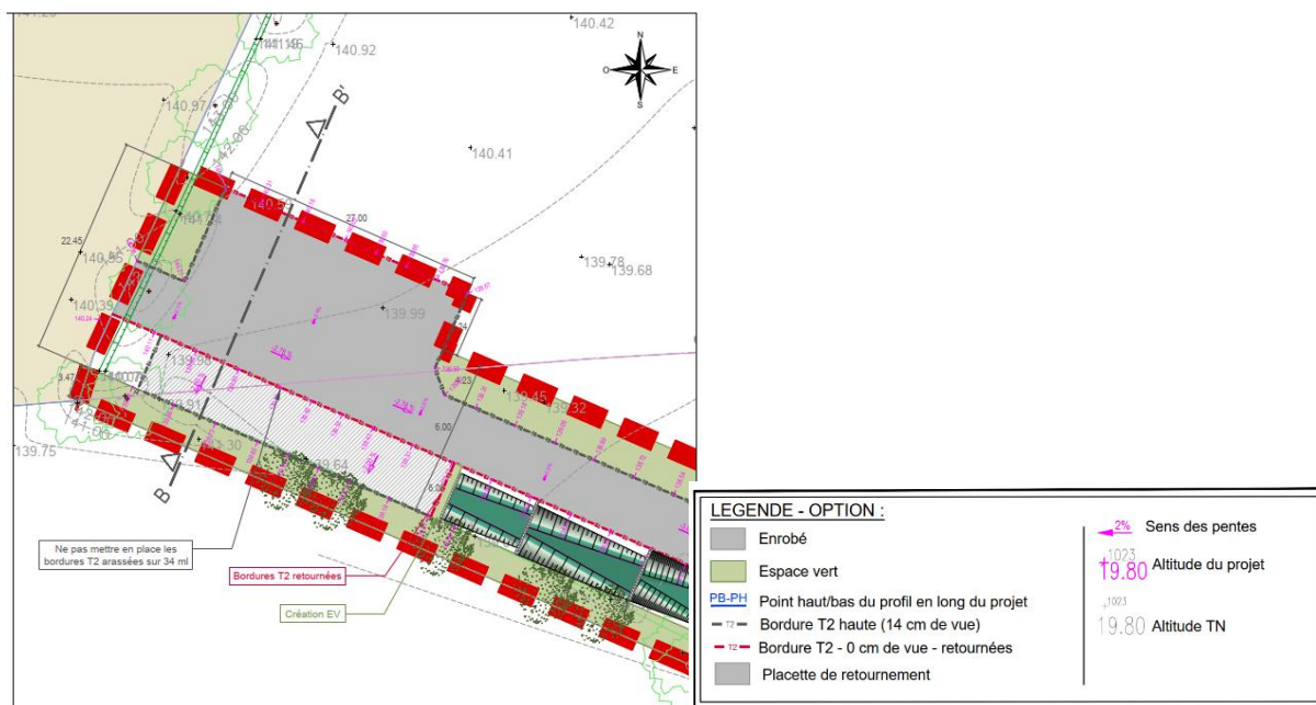
Illustration N°73: Plan de travaux- Voie Sud - Option- Placette de retournement (Source : URBAe, 5 juin 2024)
