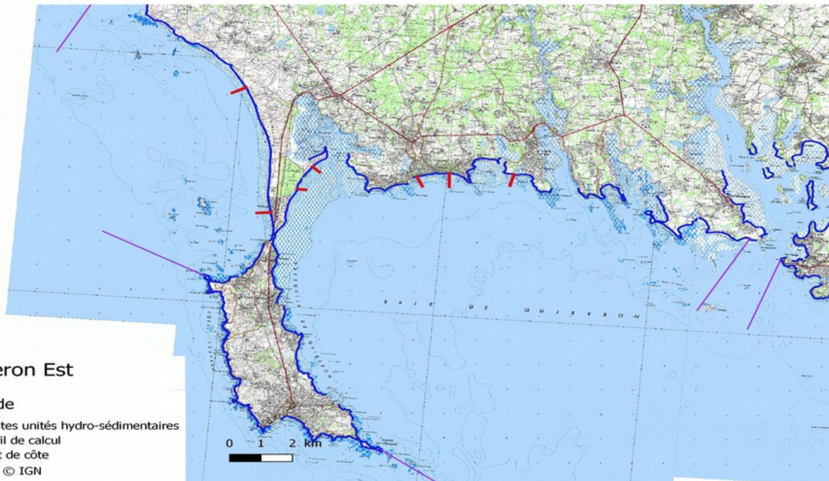
Figure 8.3 : Emplacement des profils de calcul de la composante changement climatique pour l'unité « Quiberon Est »
