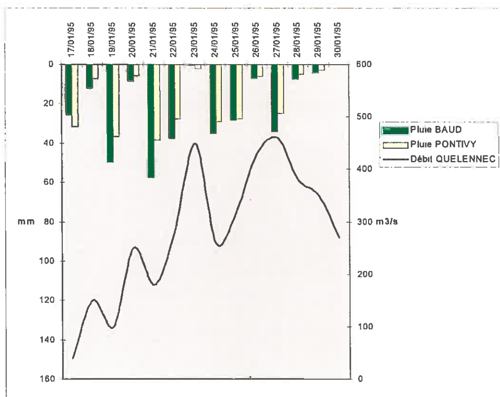
Hydrogramme à Queleennec et pluie journalière correspondante
