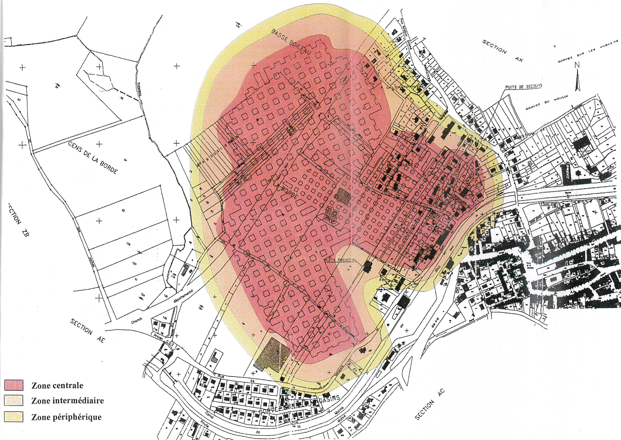
Figure 1 : Identification des zones sensibles à des mouvements de surface en cas d'ennoyage non maîtrisé de la mine.
