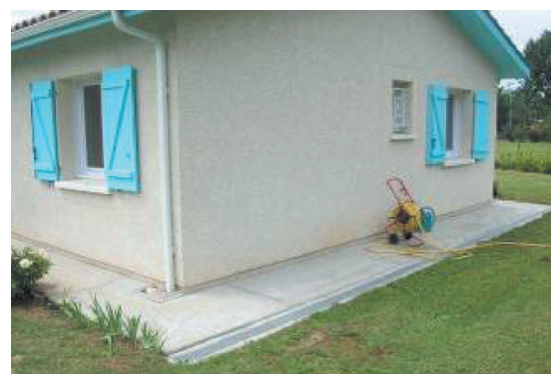
Figure 20 Large trottoir avec caniveau de collecte des eaux de ruissellement (Source Socabat)
