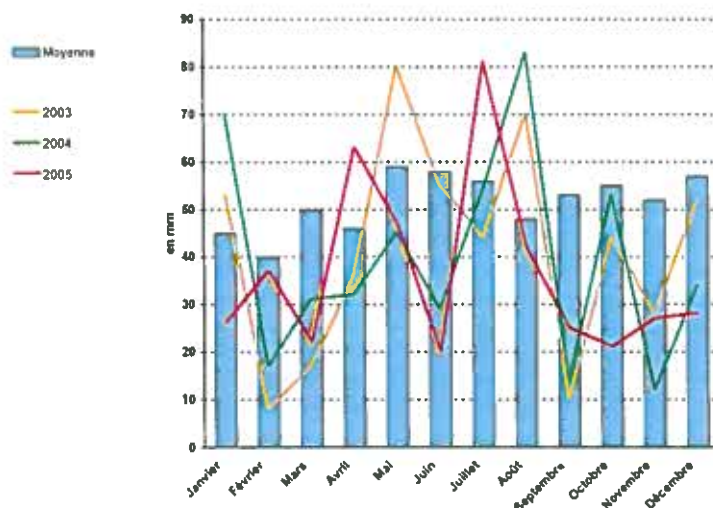
Histogramme des précipitations
