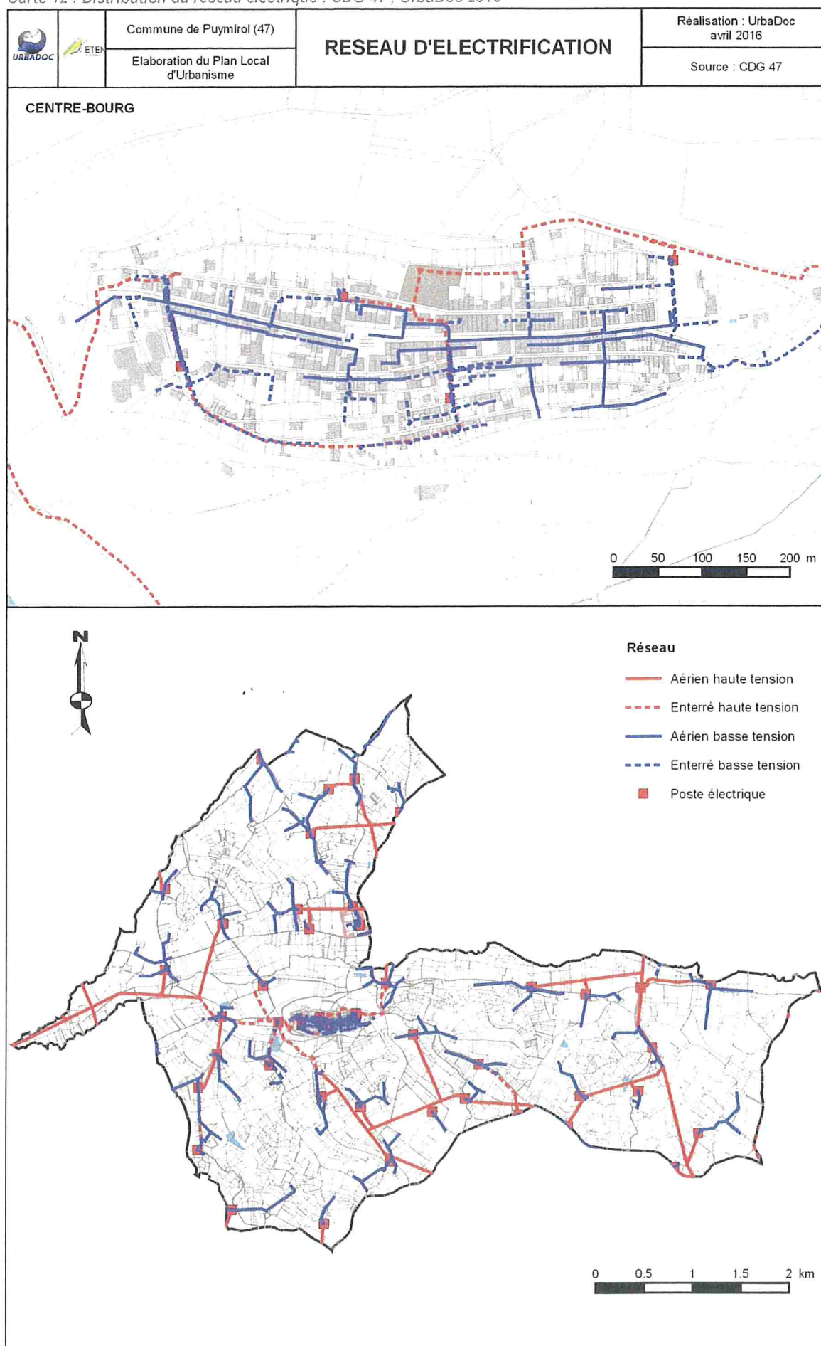
Carte 12 : Distribution du réseau électrique ; CDG 47 ; UrbaDoc 2016
