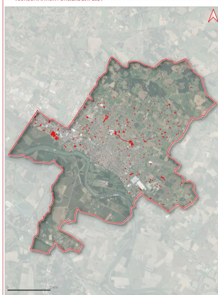
CONSOMMATION FONCIERE 2011-2024
