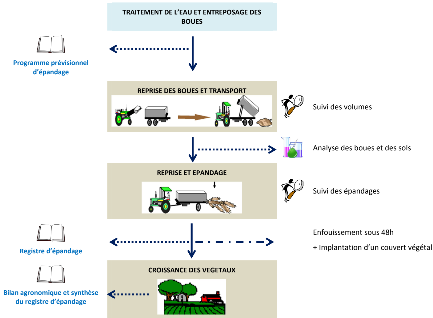
Figure 3 : Déroulement de la filière de valorisation agricole
