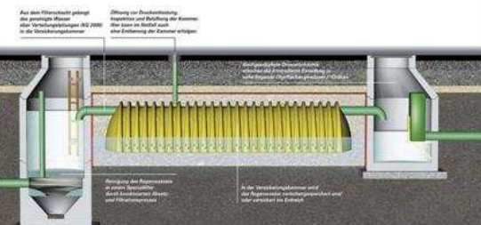
Technologie « eurofiltrator »
